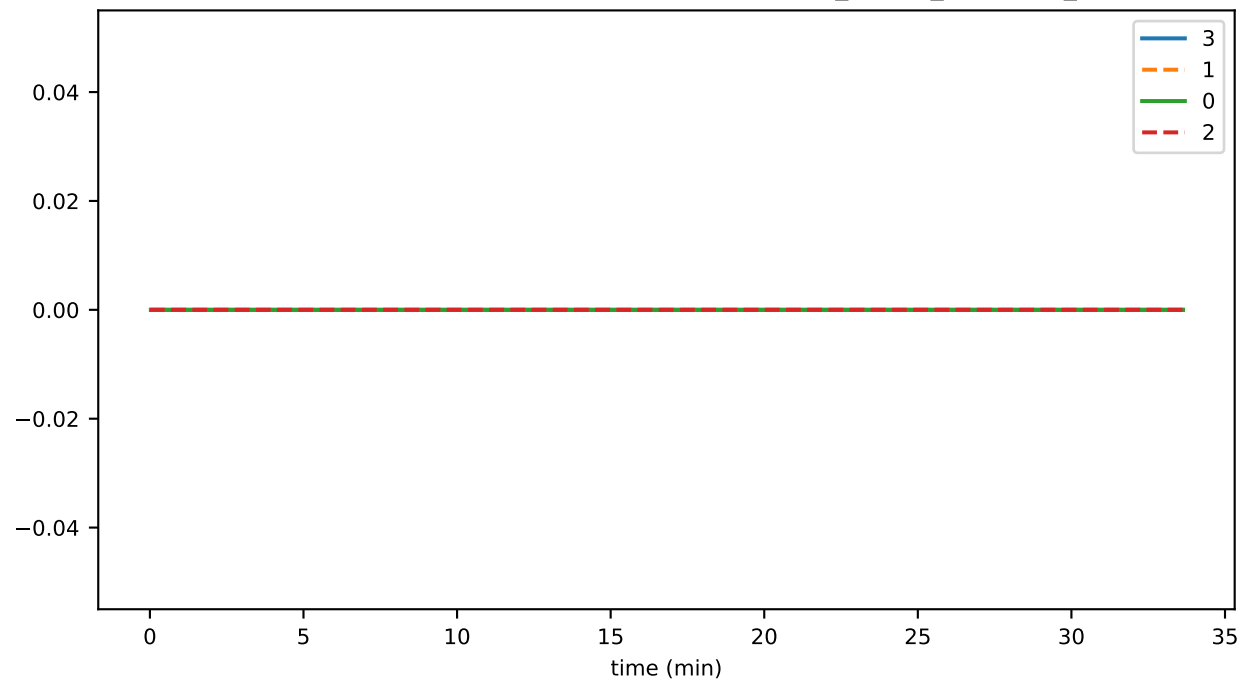
SmartContractService:SystemContractMethodCall_PAUSE_UNPAUSE_total
