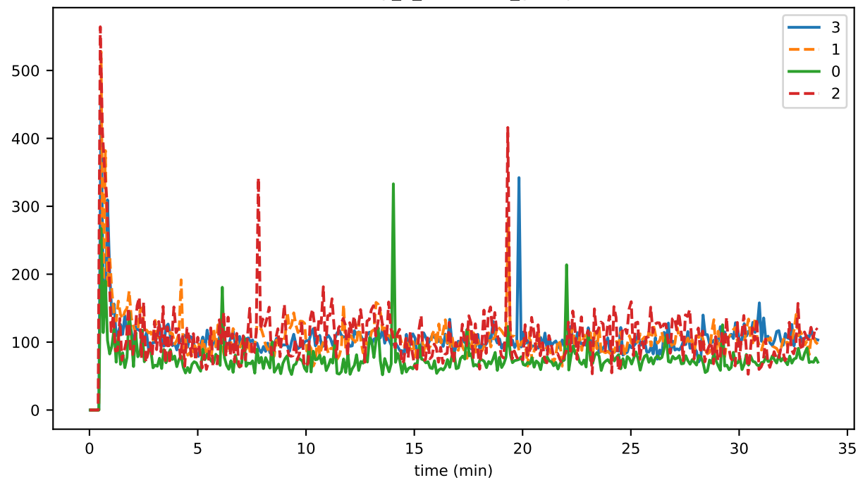
eventDelay_2_validation_runtimeMAX
