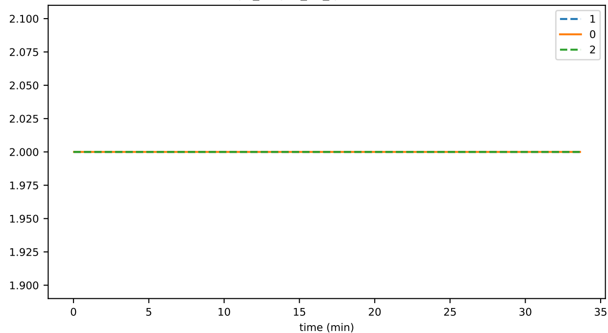
rpc_output_queue_poll_time
