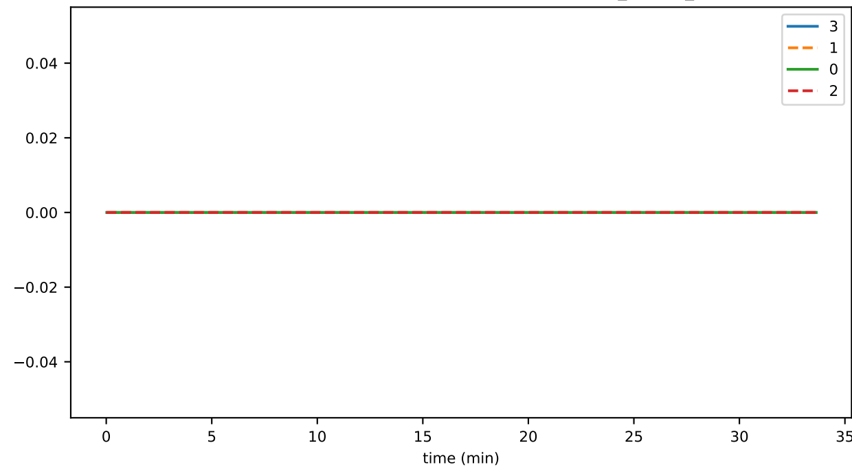
SmartContractService:SystemContractMethodCall_PROXY_failed
