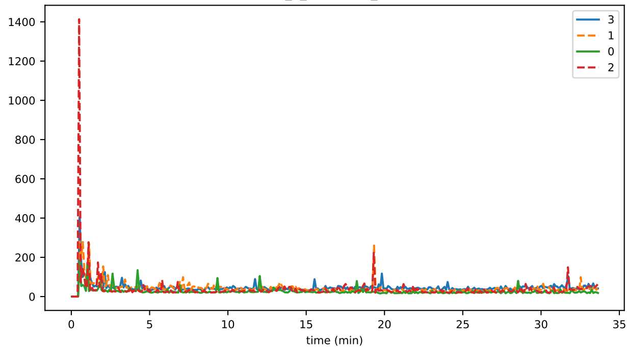
eventDelay_2_validation_runtimeMAX
