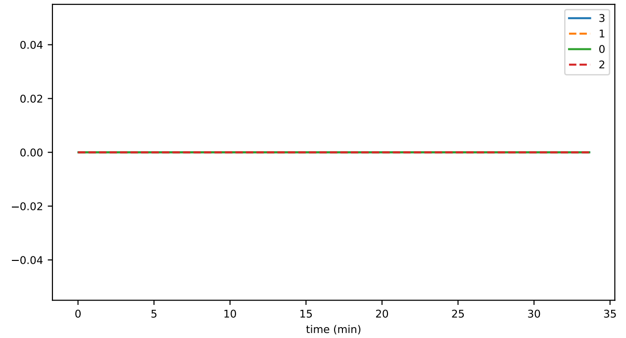
DigSubWrkItmTime
