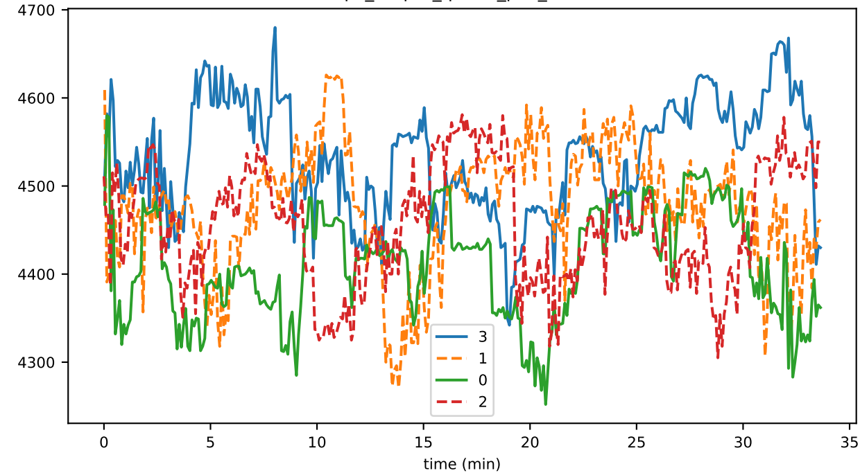
rpc_output_queue_poll_time
