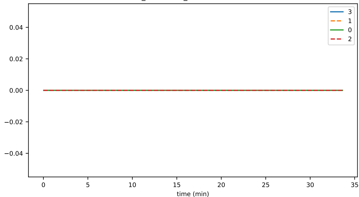
conn_connClose_internalError
