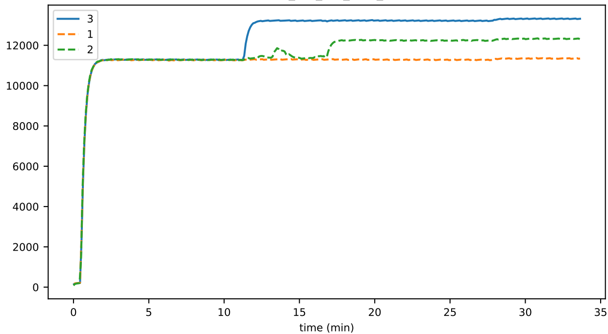
bytes_per_sec_sent_00
