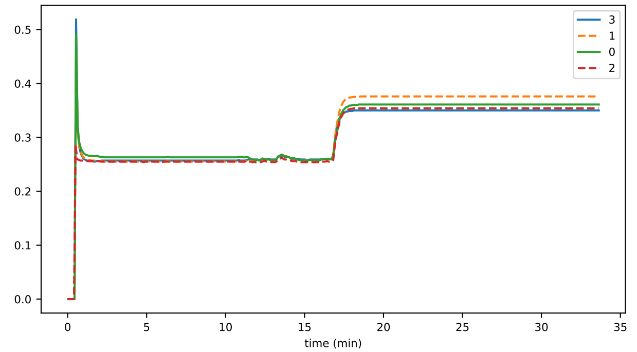
secC2RC
