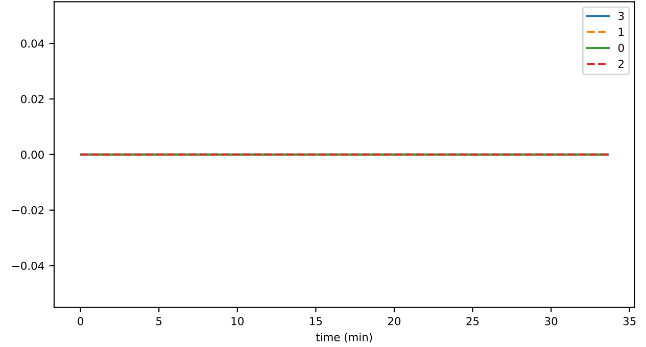
SmartContractService:SystemContractMethodCall_IS_AUTHORIZED_failed
