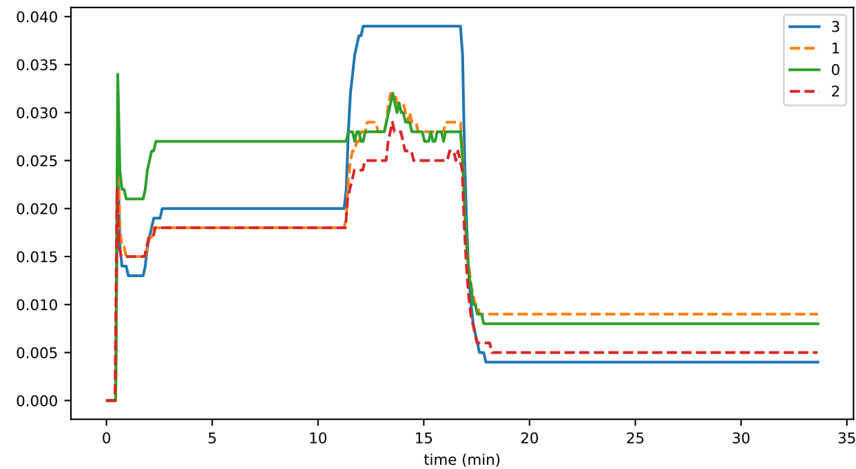
secR2F
