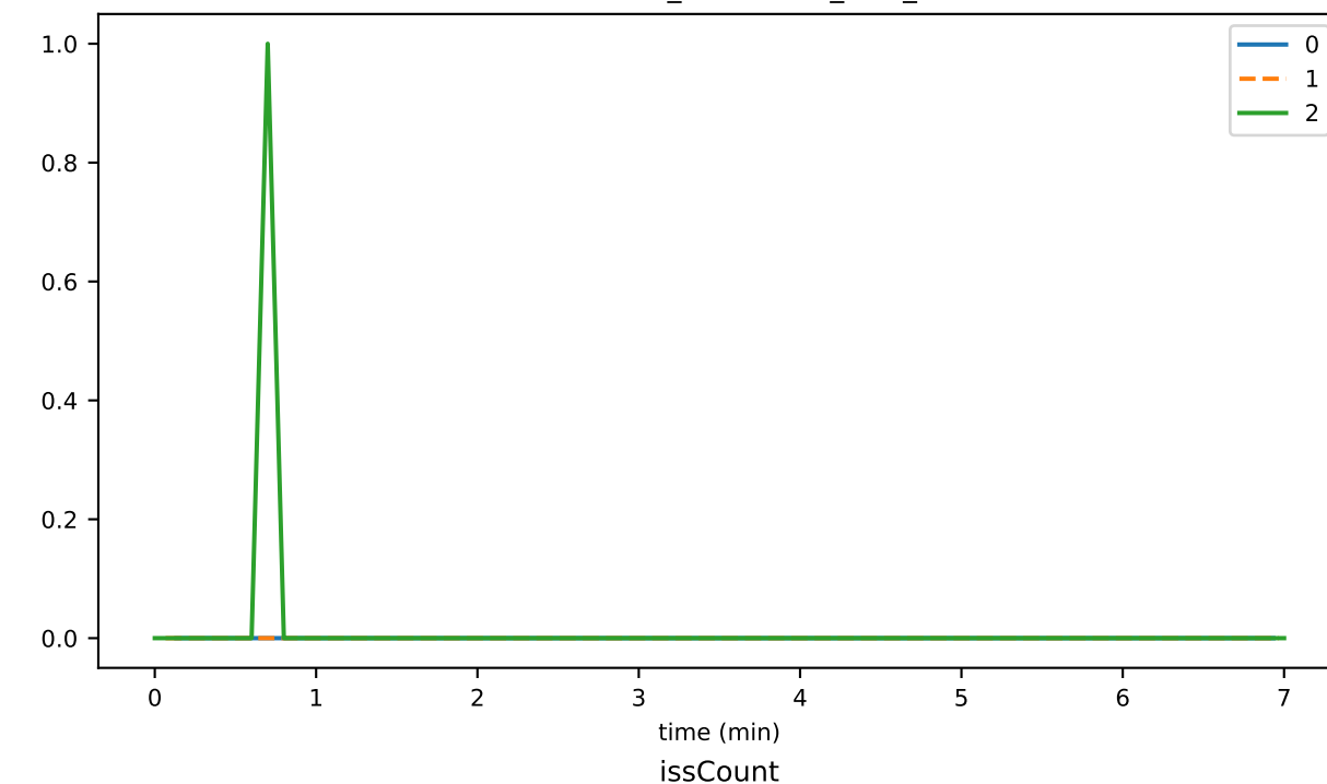
InlinePcesWriter_unhandled_task_count
