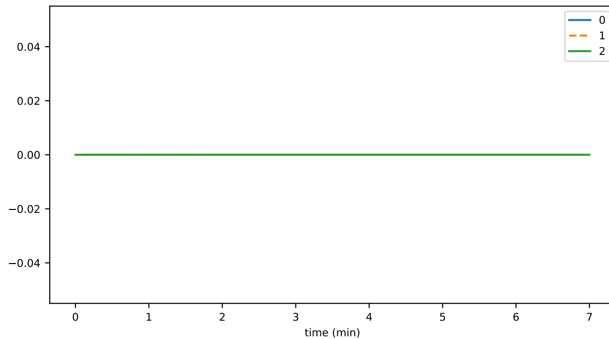
issCount
