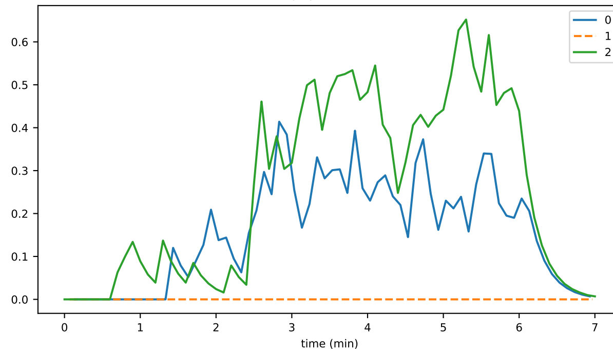
PlatformMonitor_unhandled_task_count
