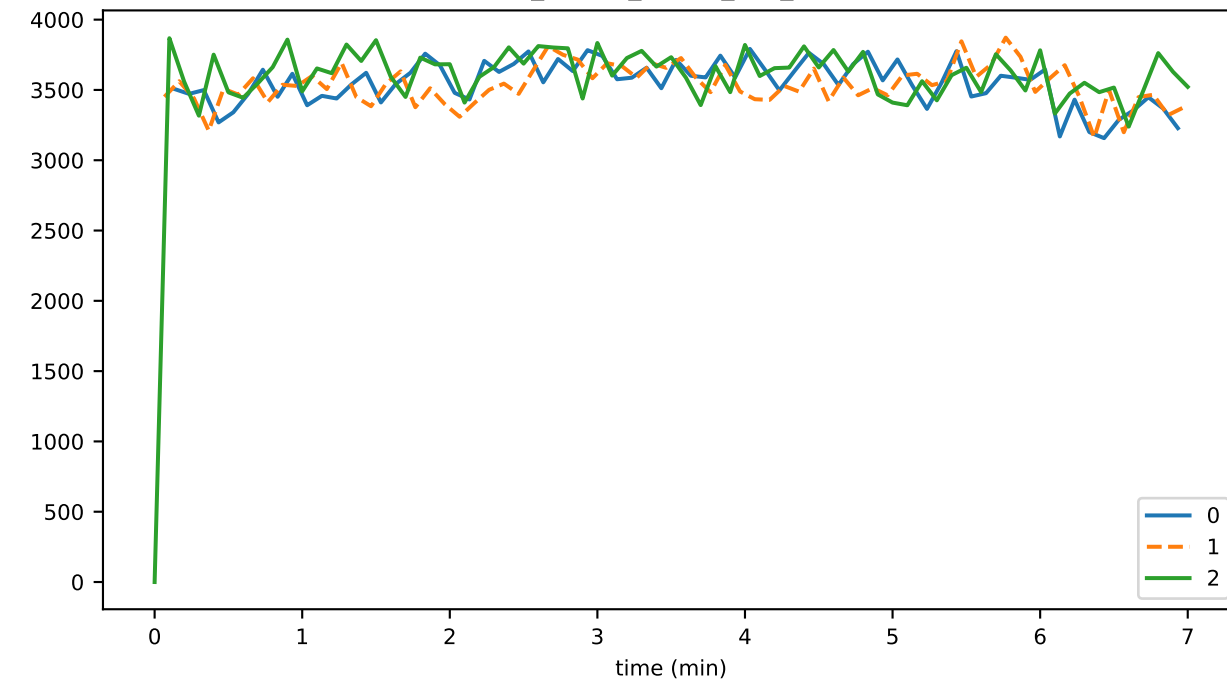
rpc_output_queue_poll_time
