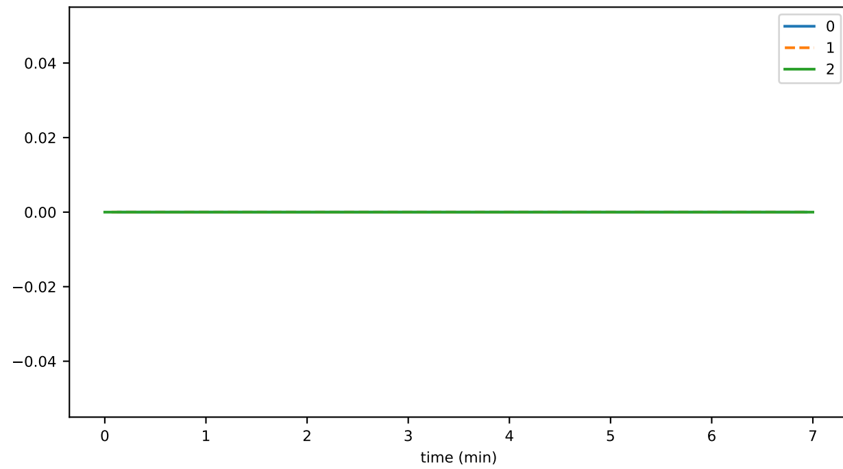
scheduleCreateThrottledTxns
