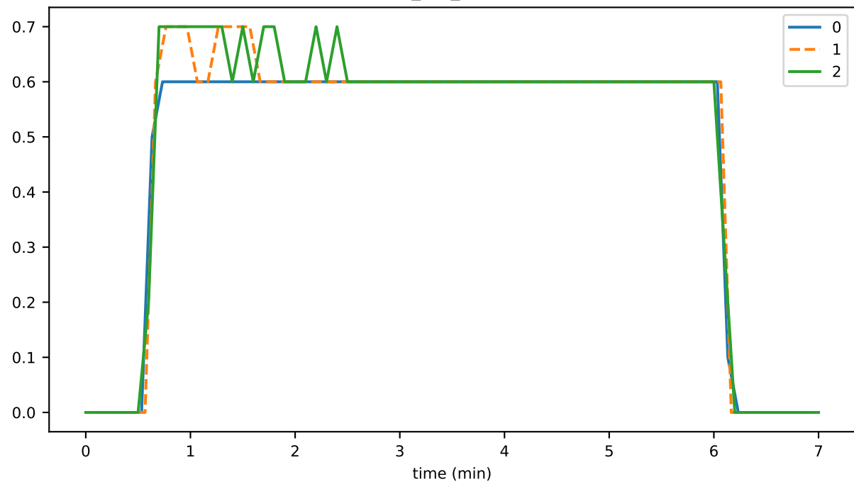
ev_per_syncR
