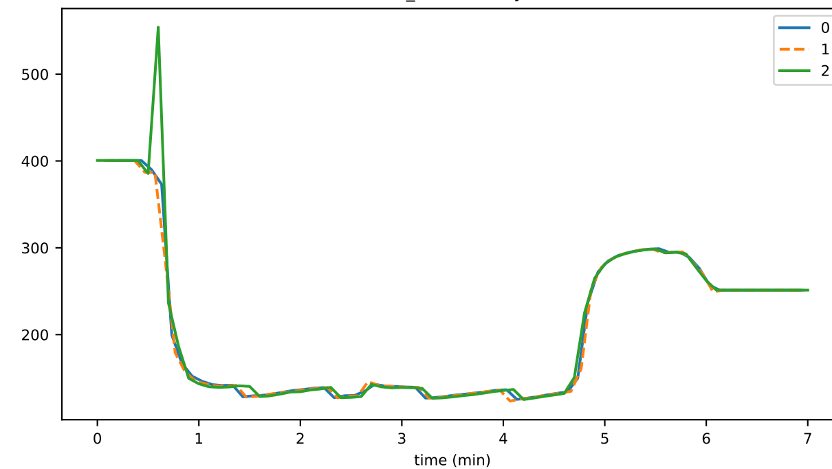
buffer_blockItemBytes
