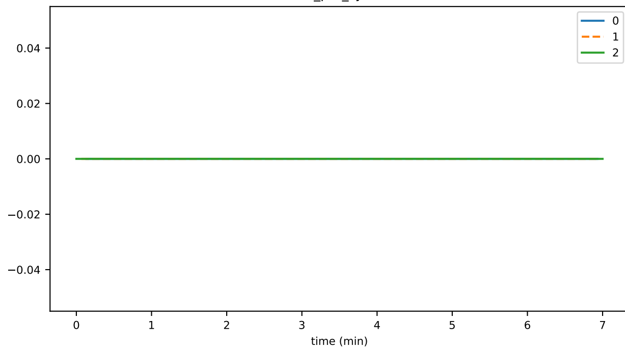
secC2R
