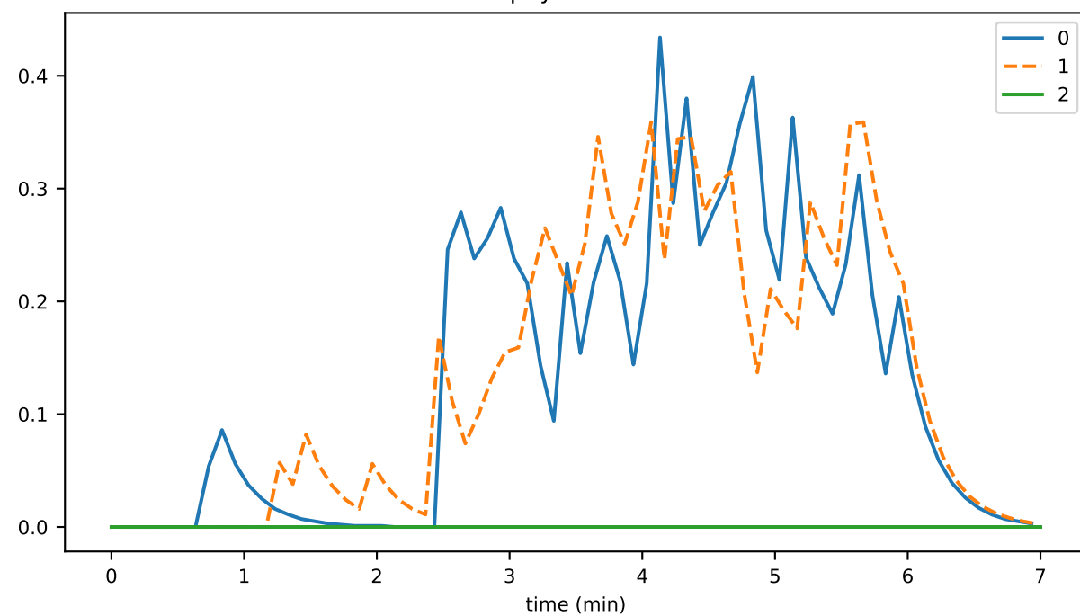
pityParent2
