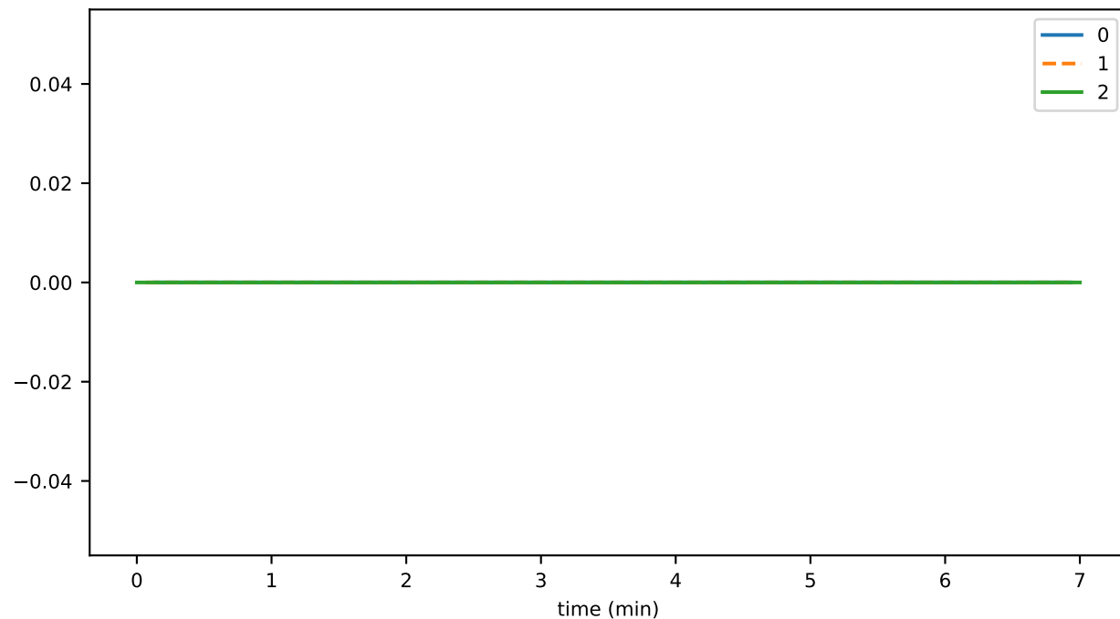
nodeUpdateThrottledTxns
