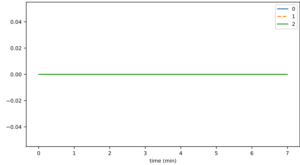
gossip_unhandled_task_count
