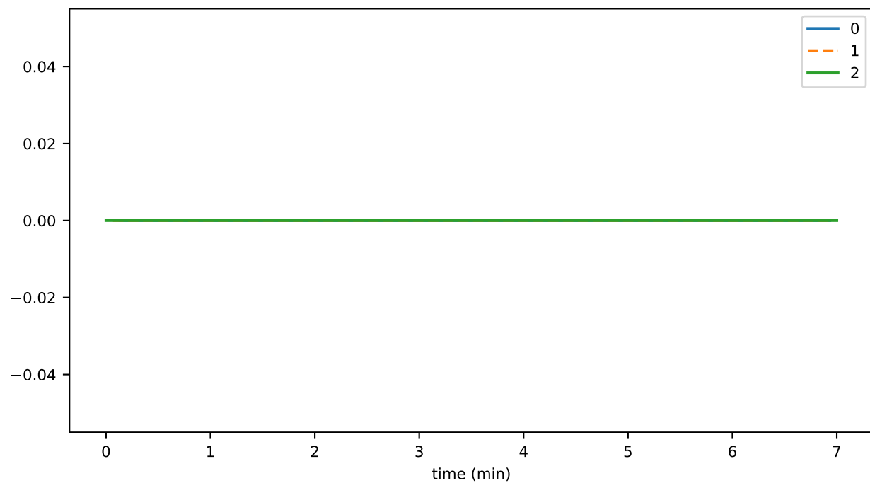
endsReconnectAsSender
