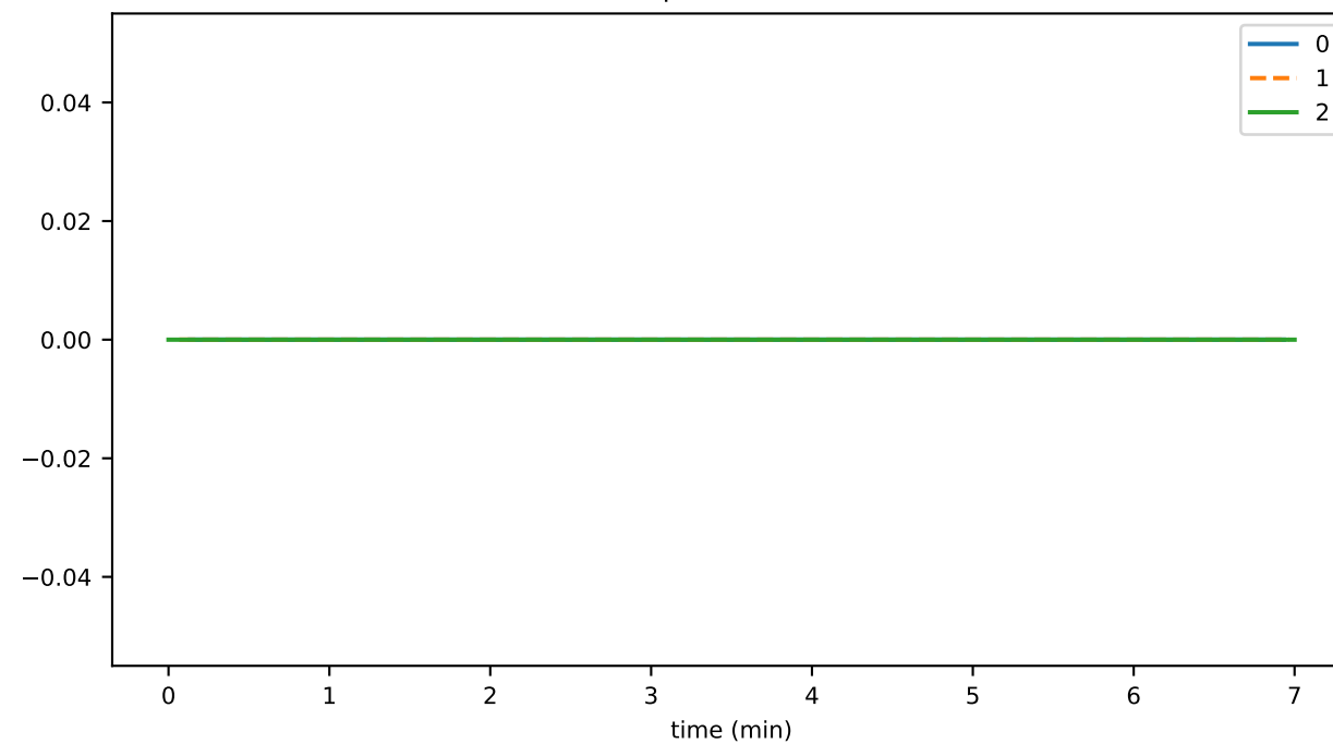
numReportFallenBehind
