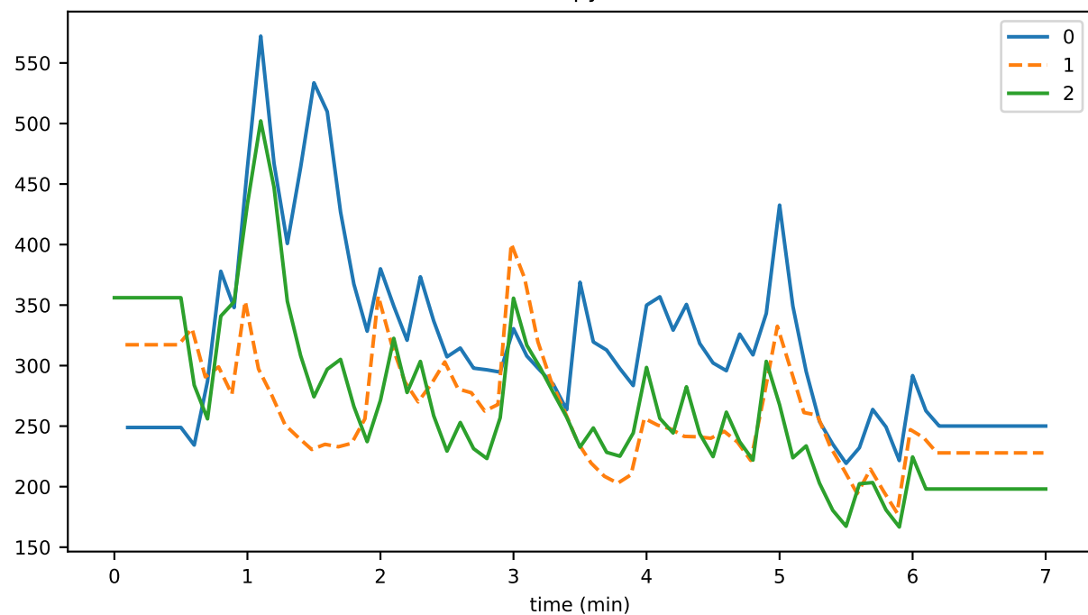
StateHasher_busy_fraction
