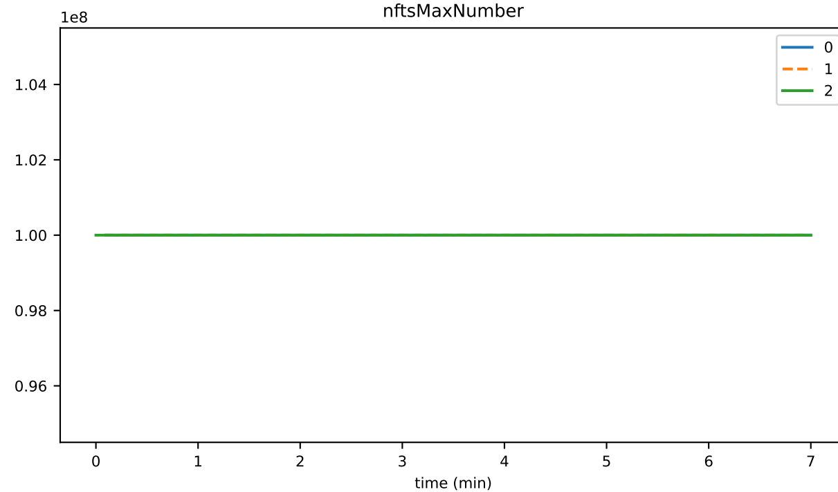
nftsMaxNumber
