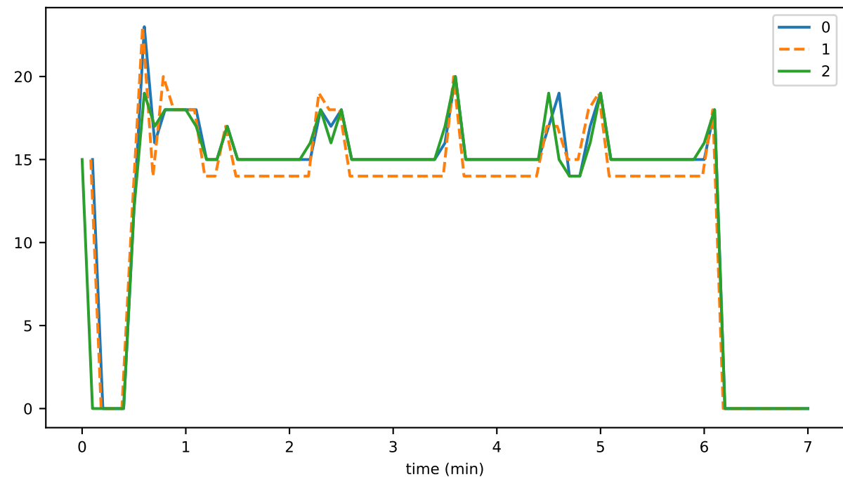
numReportFallenBehind
