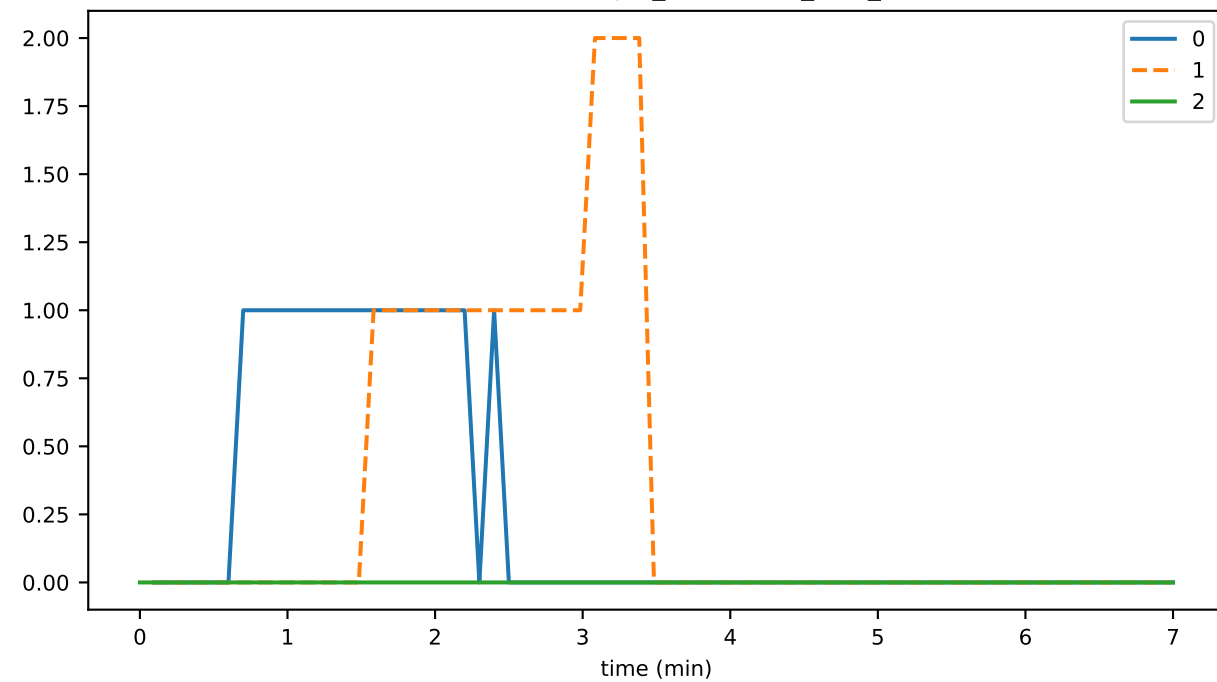
EventDeduplicator_unhandled_task_count
