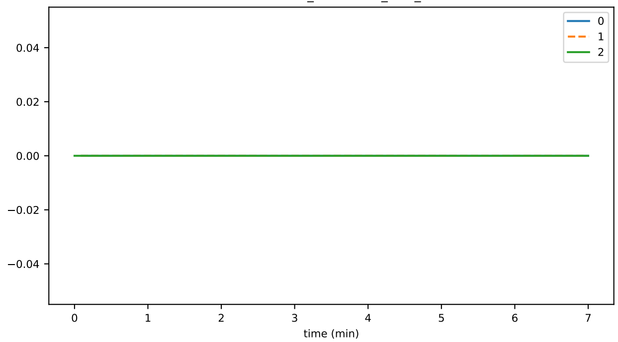
PlatformMonitor_unhandled_task_count
