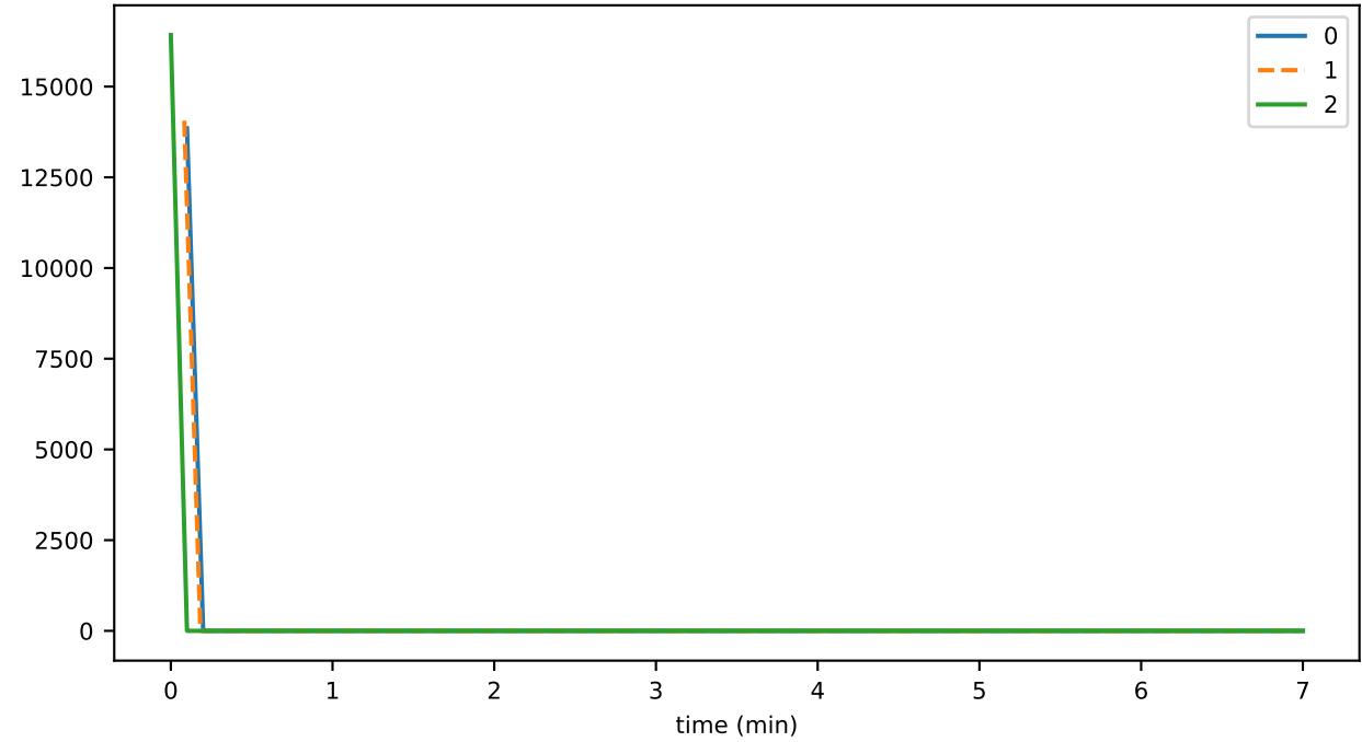
eventDelay_2_validation_gossipMAX
