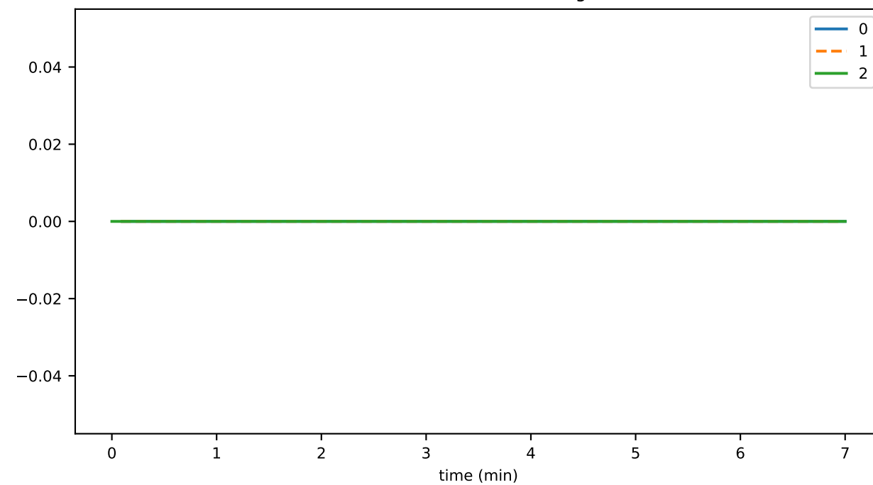
tokenPauseThrottledTxns
