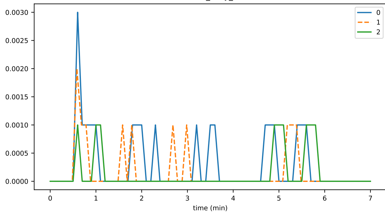
StateHasher_busy_fraction
