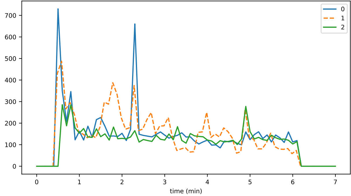
eventDelay_2_validation_gossipMAX
