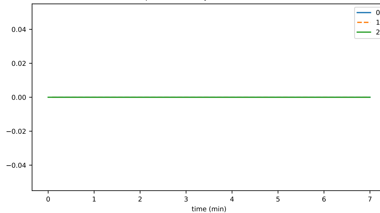
hapiBalanceQueryLimitsPercentUsed
