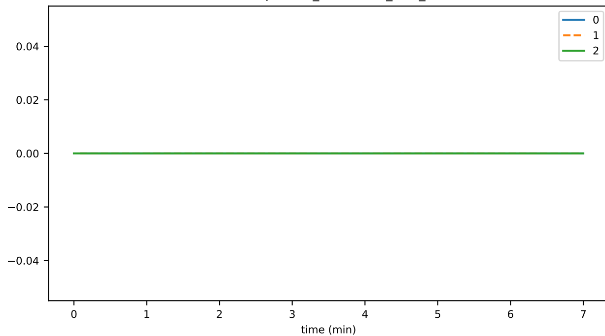
EventDeduplicator_unhandled_task_count
