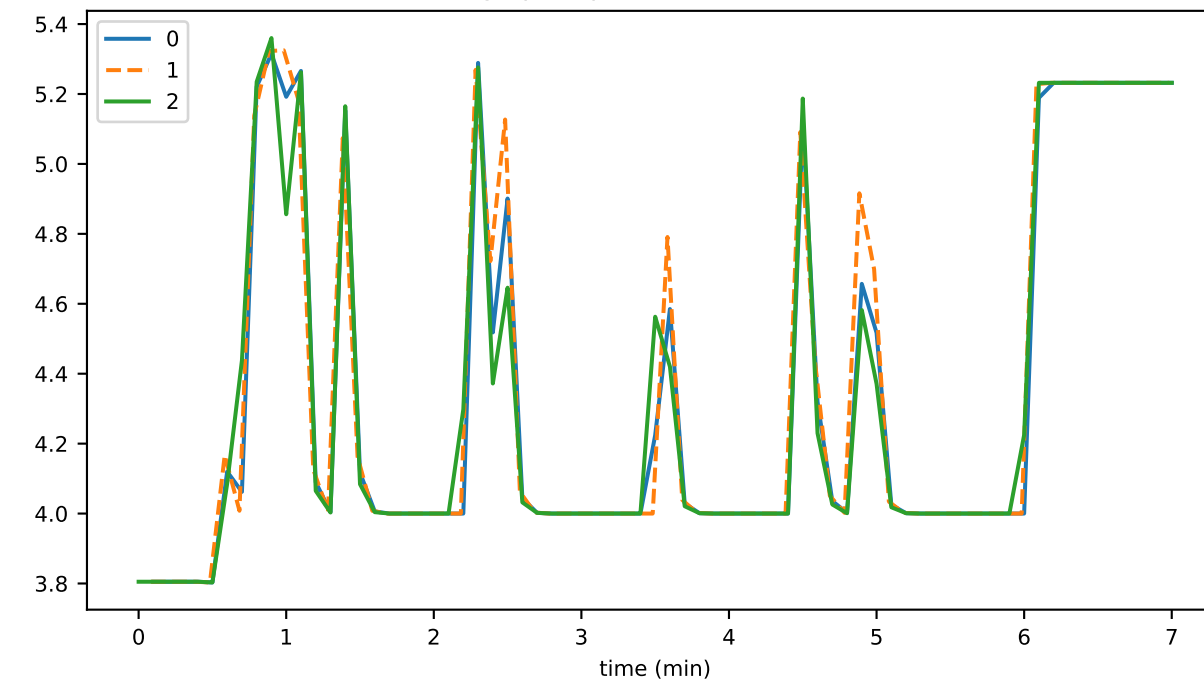
hapiBalanceQueryLimitsPercentUsed
