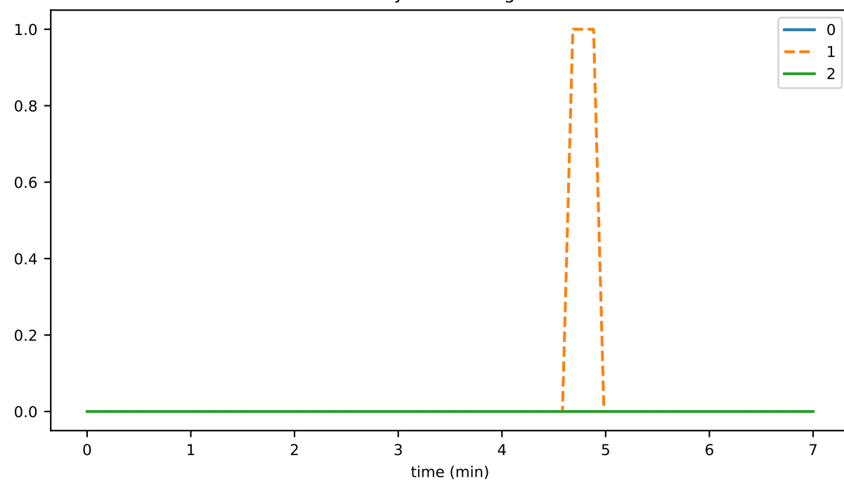
syncRoundLag
