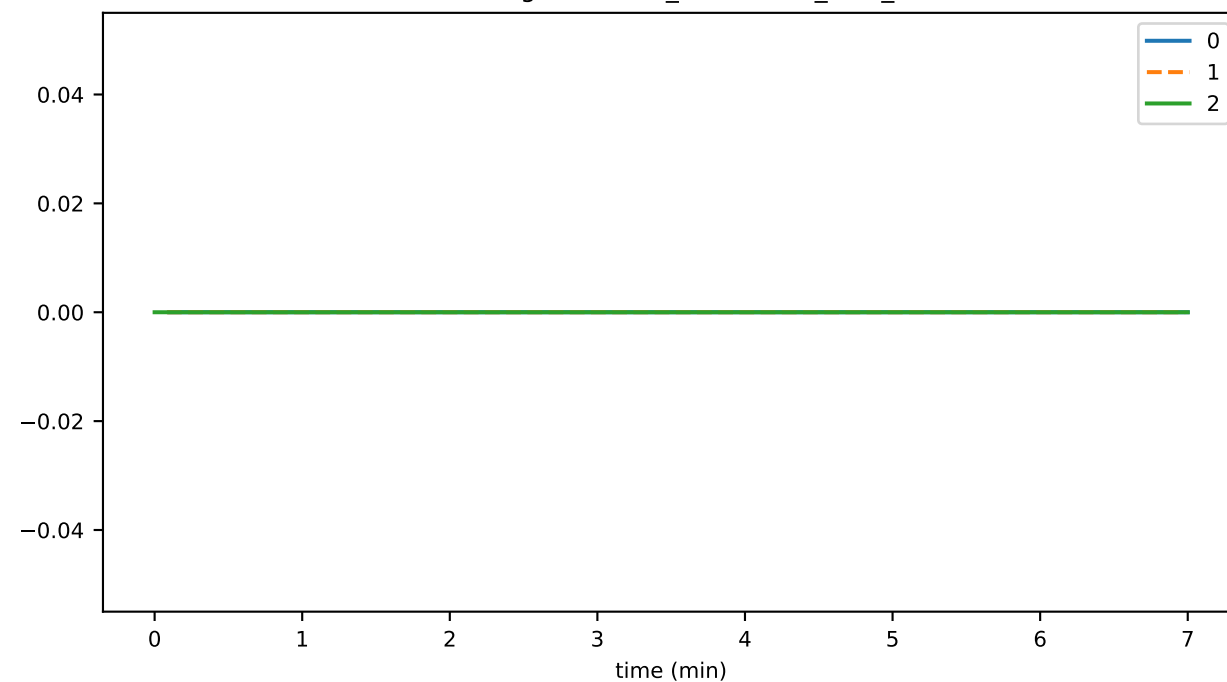
StateHasher_unhandled_task_count
