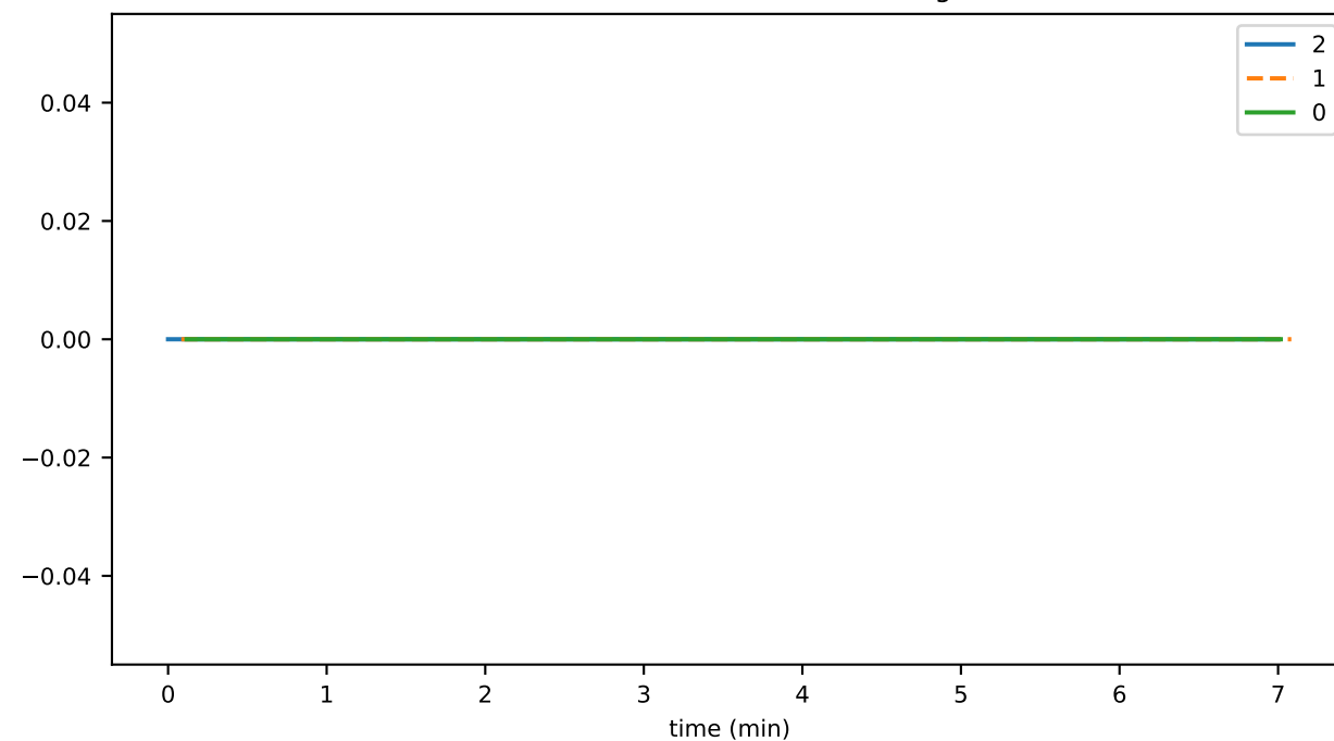
contractAutoRenewThrottledTxns
