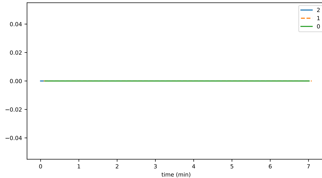
contractAutoRenewThrottledTxns
