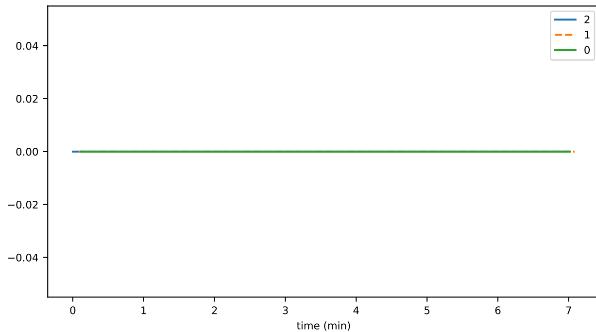
tokenCreateThrottledTxns
