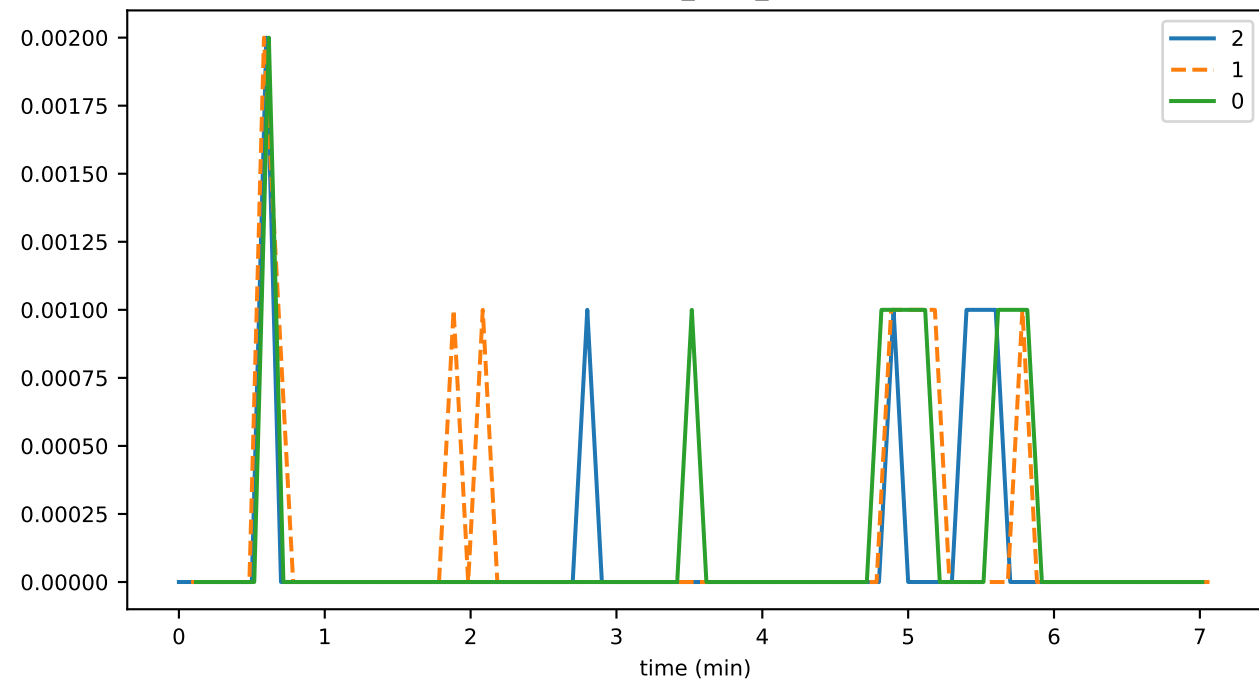
StateHasher_busy_fraction
