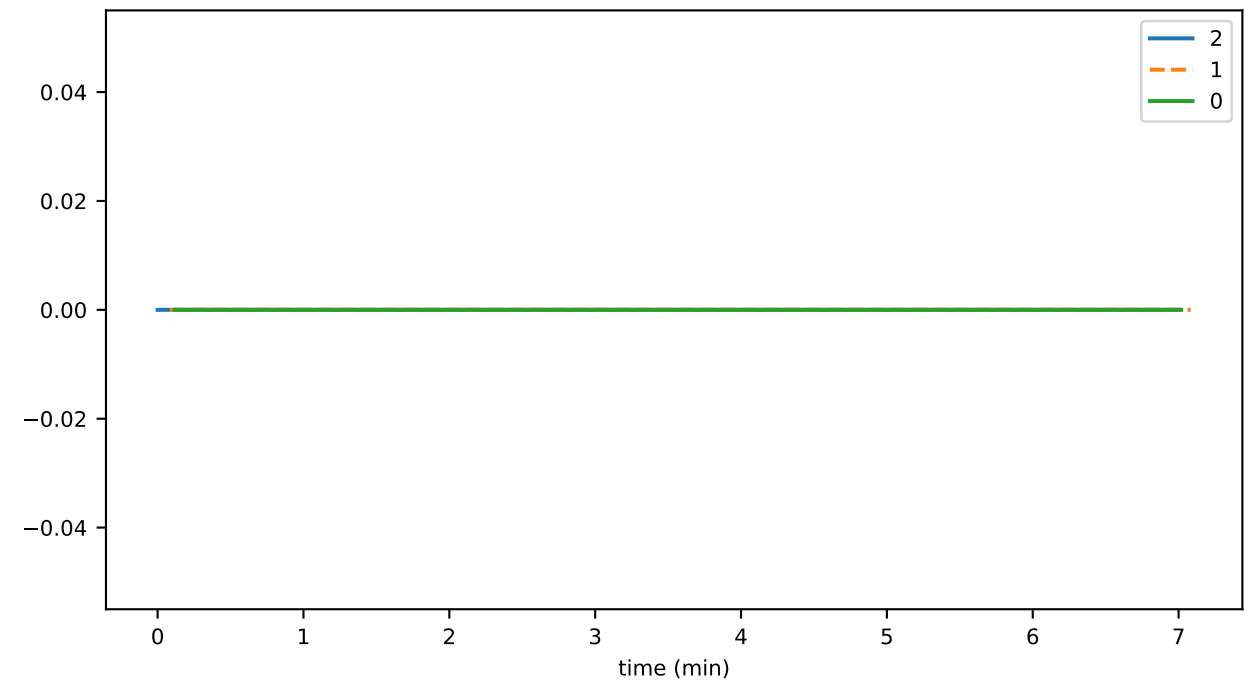
hapiBalanceQueryLimitsPercentUsed
