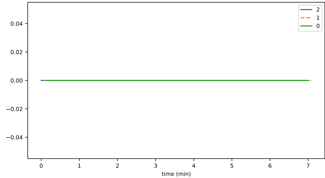
hapiGasPercentUsed
