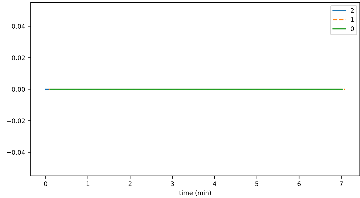
createTransactionRecordThrottledTxns
