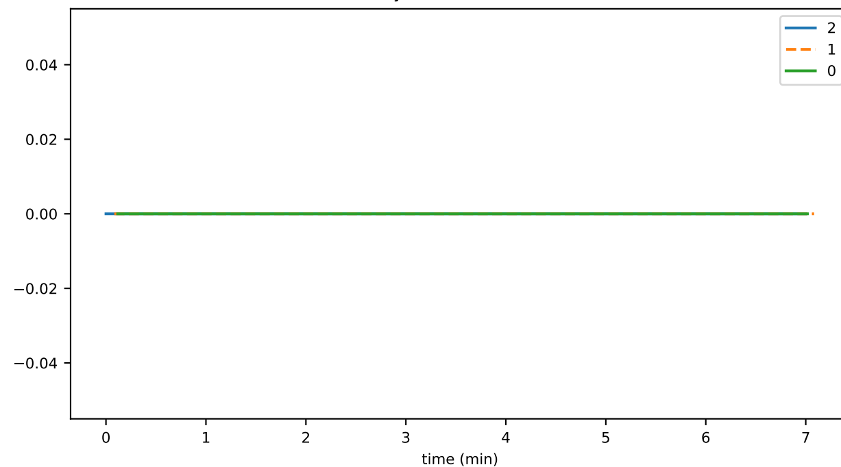
tokensPercentUsed
