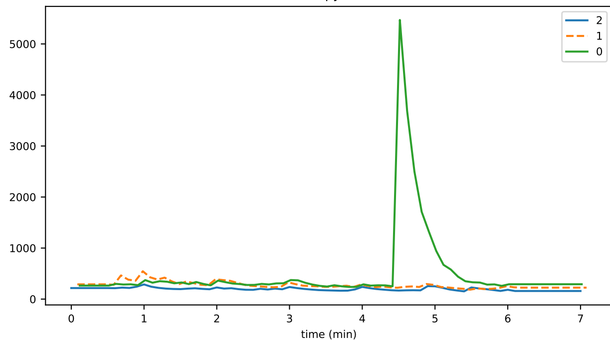
StateHasher_busy_fraction
