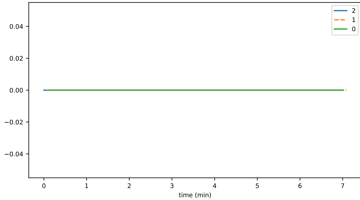
EventDeduplicator_unhandled_task_count
