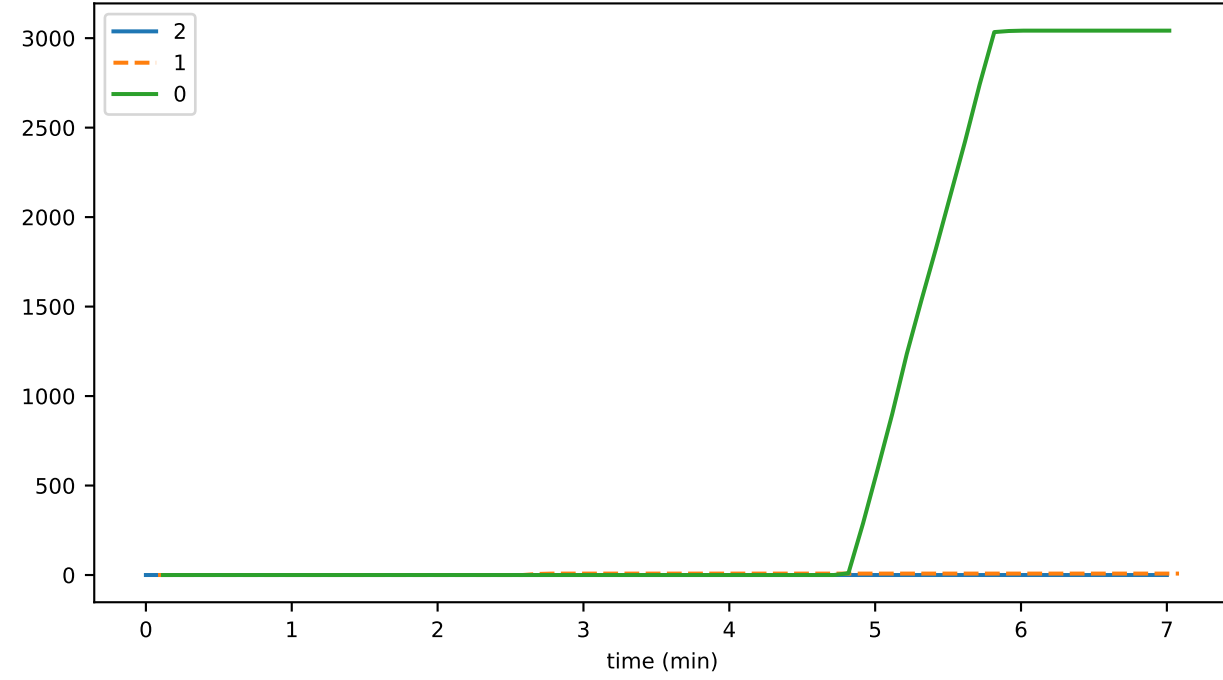
DeprTxnsRcv
