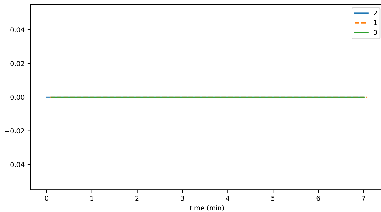
tokenFreezeAccountThrottledTxns
