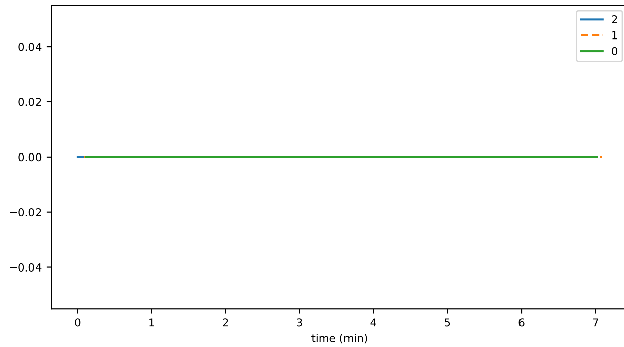
tokenUpdateNftsDurationMax
