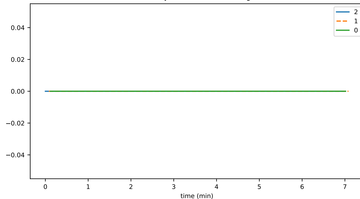
historyProofVoteThrottledTxns
