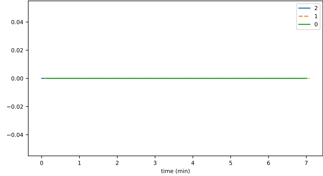
gasPerConsSec
