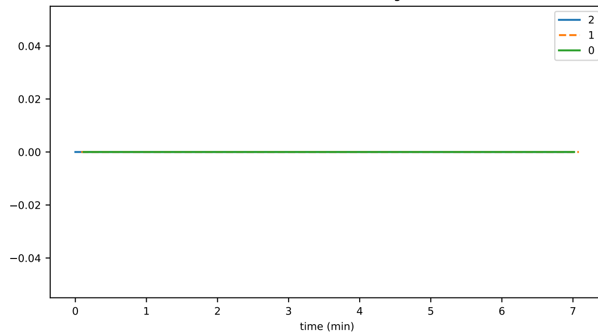
tokenPauseThrottledTxns
