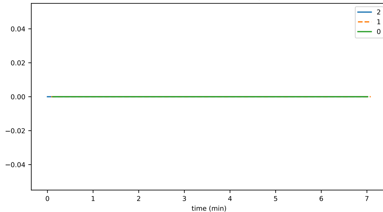
lambdaSStoreThrottledTxns
