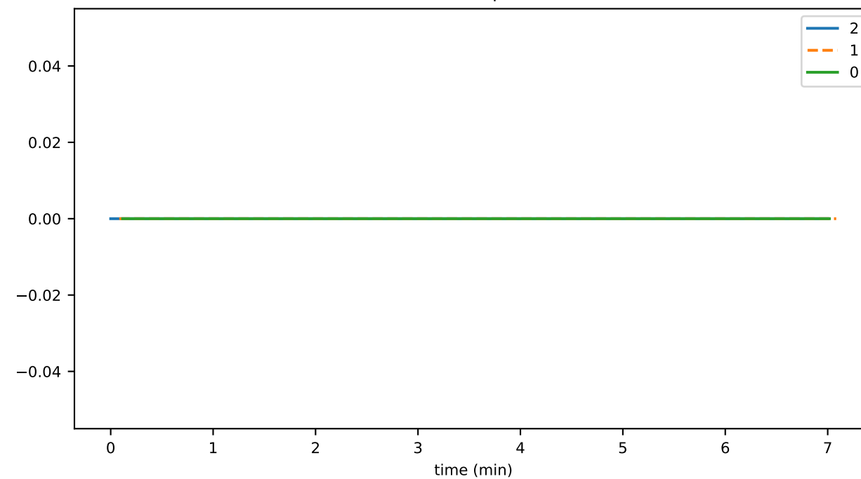
tokenCancelAirdropDurationMax
