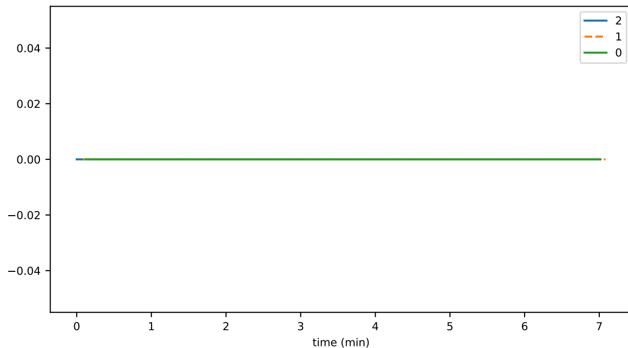
nodeCreateThrottledTxns
