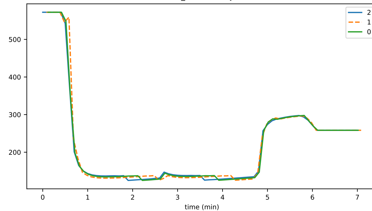
buffer_blockItemBytes
