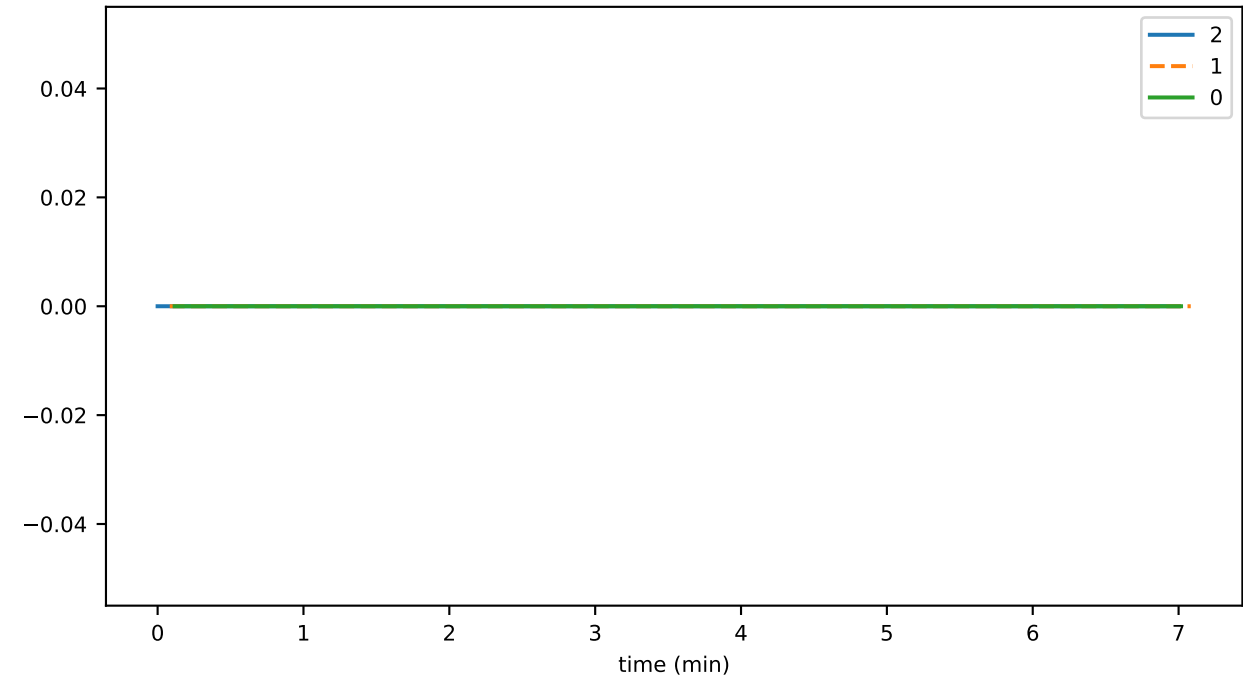
SmartContractService:SystemContractMethodCall_IS_AUTHORIZED_failed
