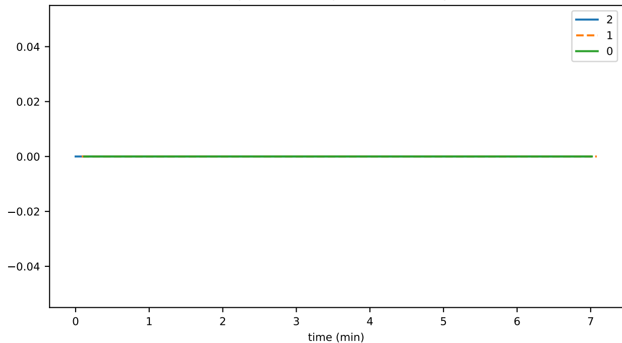
registeredNodeUpdateThrottledTxns
