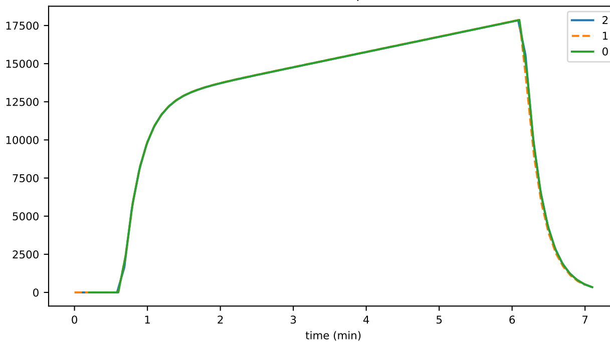
roundSup
