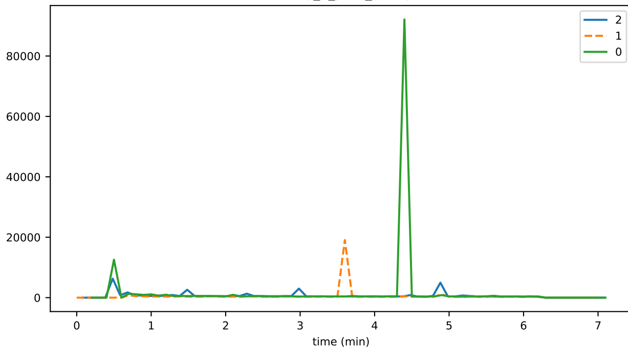
eventDelay_6_pces_runtimeMAX
