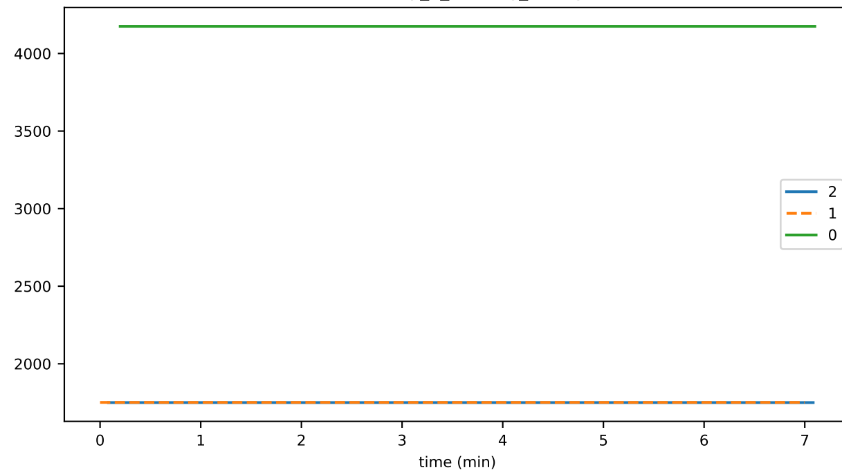
eventDelay_2_validation_gossip
