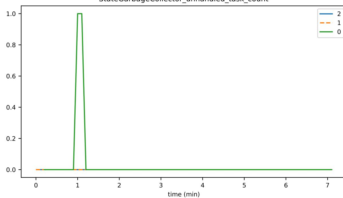
StateGarbageCollector_unhandled_task_count
