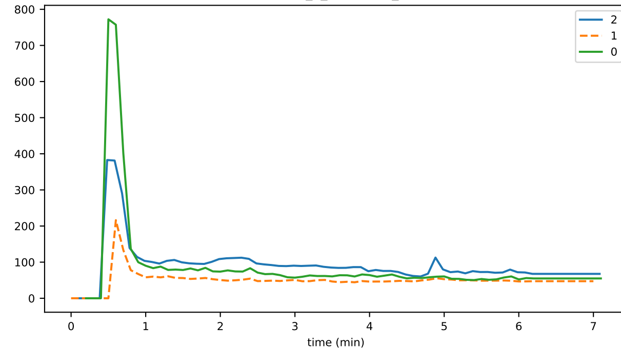
eventDelay_2_validation_gossip
