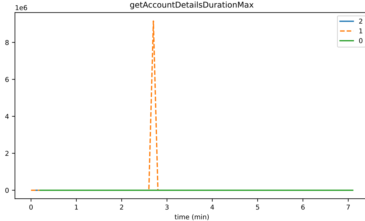
getAccountDetailsDurationMax
