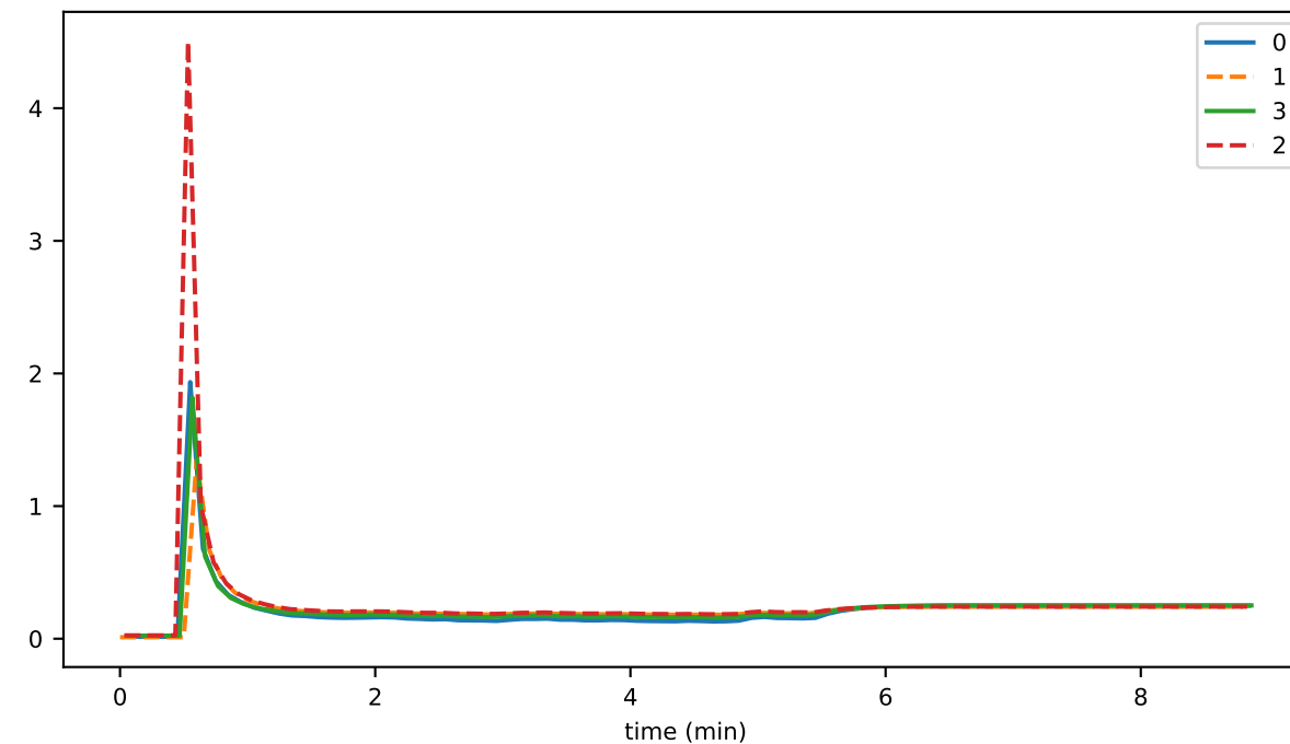
memFree (1e10)
