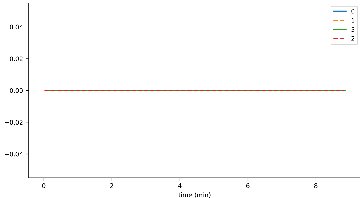
SigPulse_per_sec
