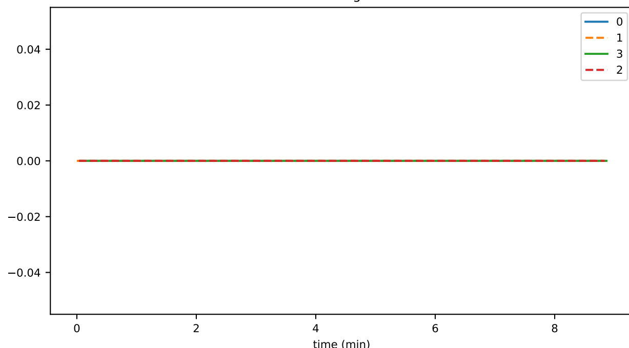
TtIDig
