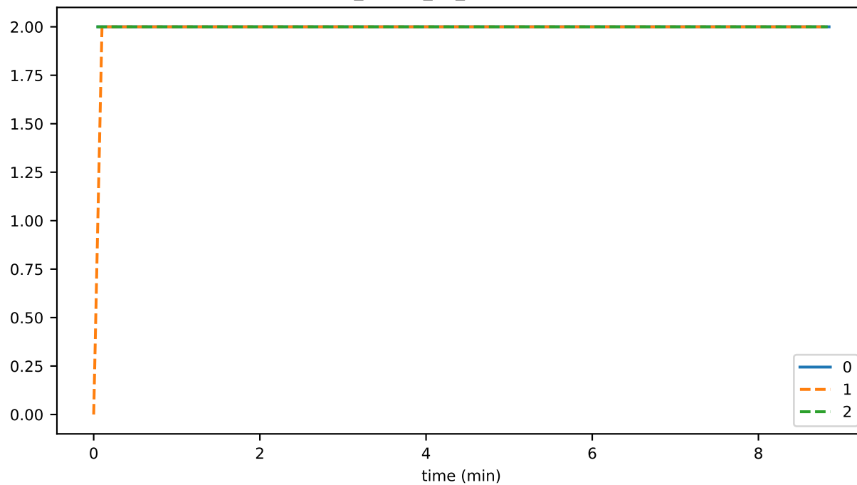
rpc_output_03_queueMaxSize
