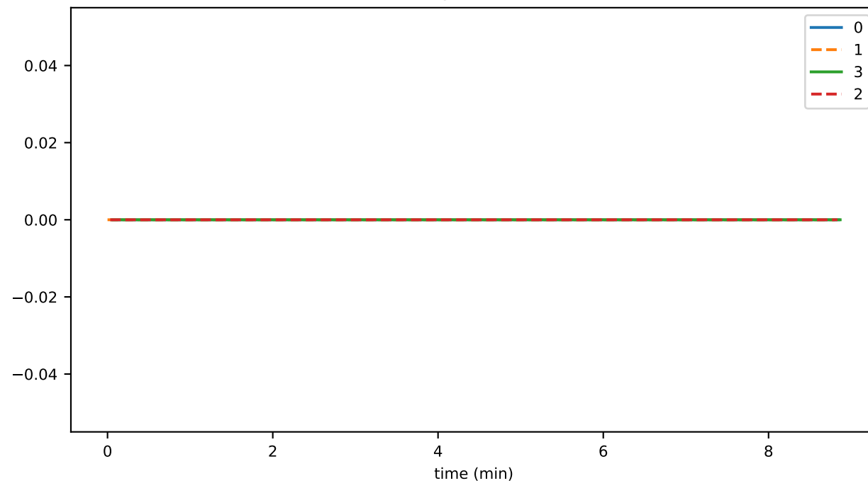
SigIntakeListSize
