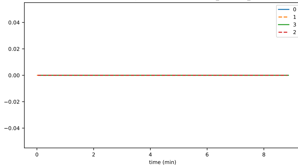
SmartContractService:SystemContractMethodCall_ALIASES_total
