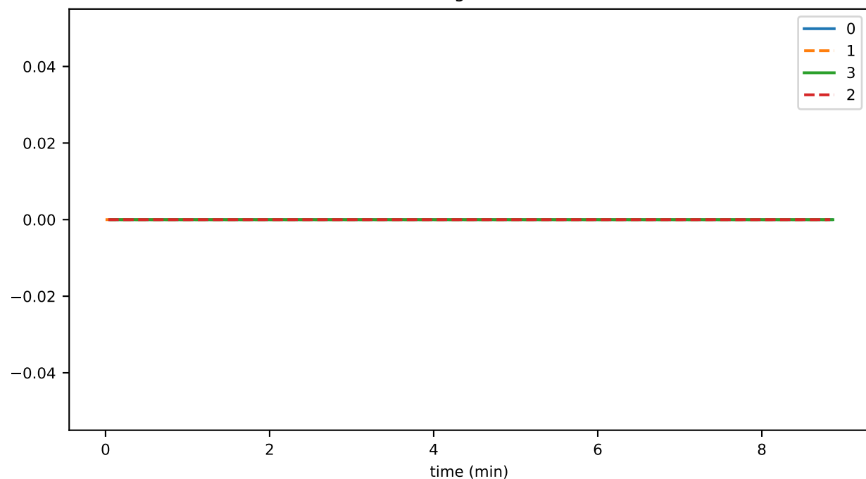
eventsInMem
