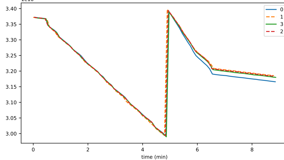
memFree (1e10)
