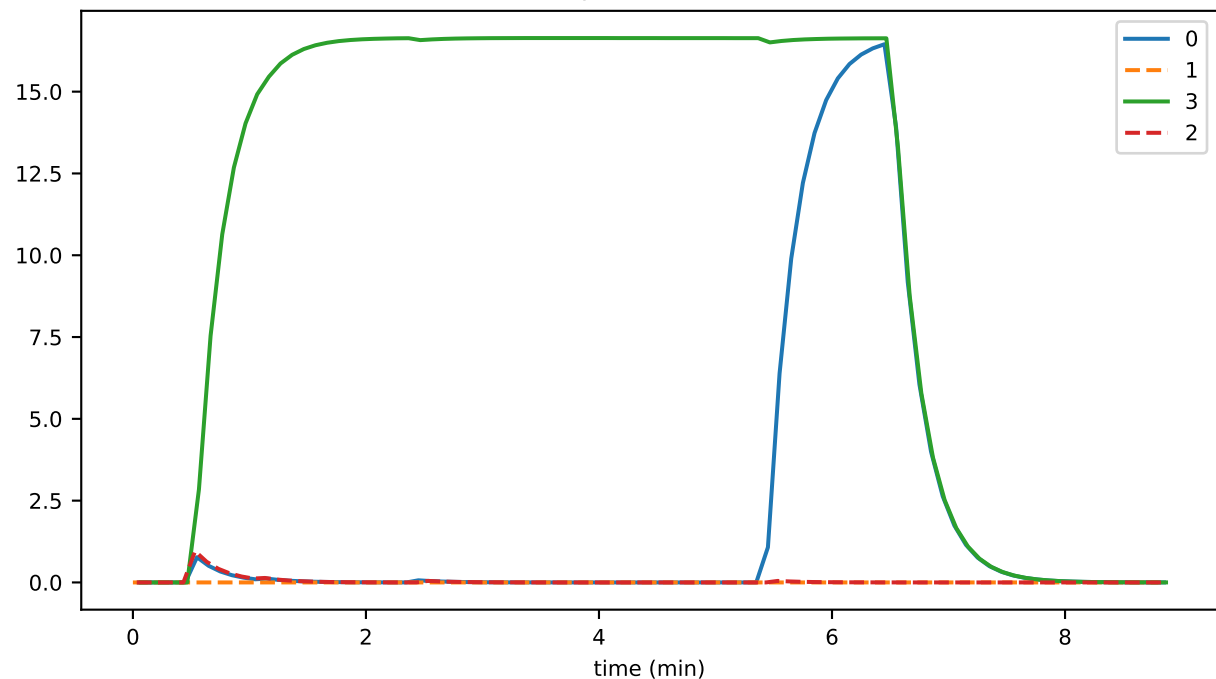
tipsetParent3
