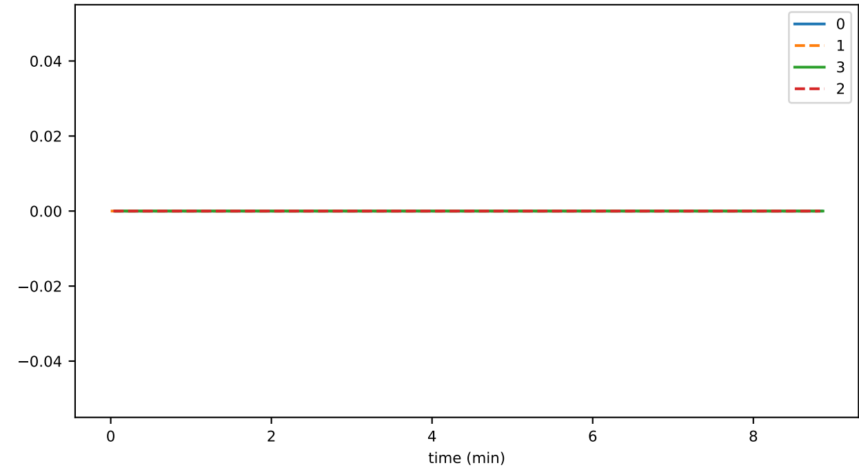
cryptoUpdateThrottledTxns
