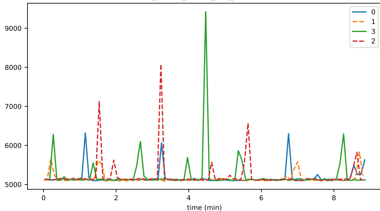
rpc_output_queue_poll_timeMAX
