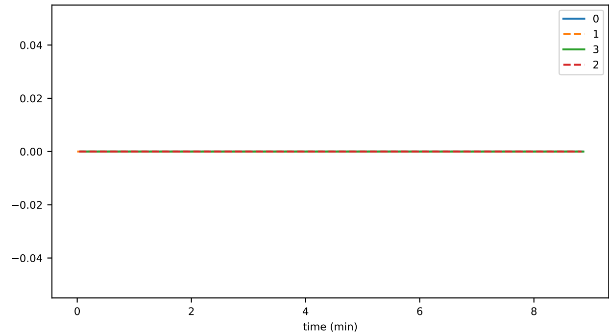
gasPerConsSec
