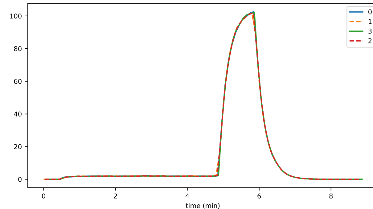
TtISig
