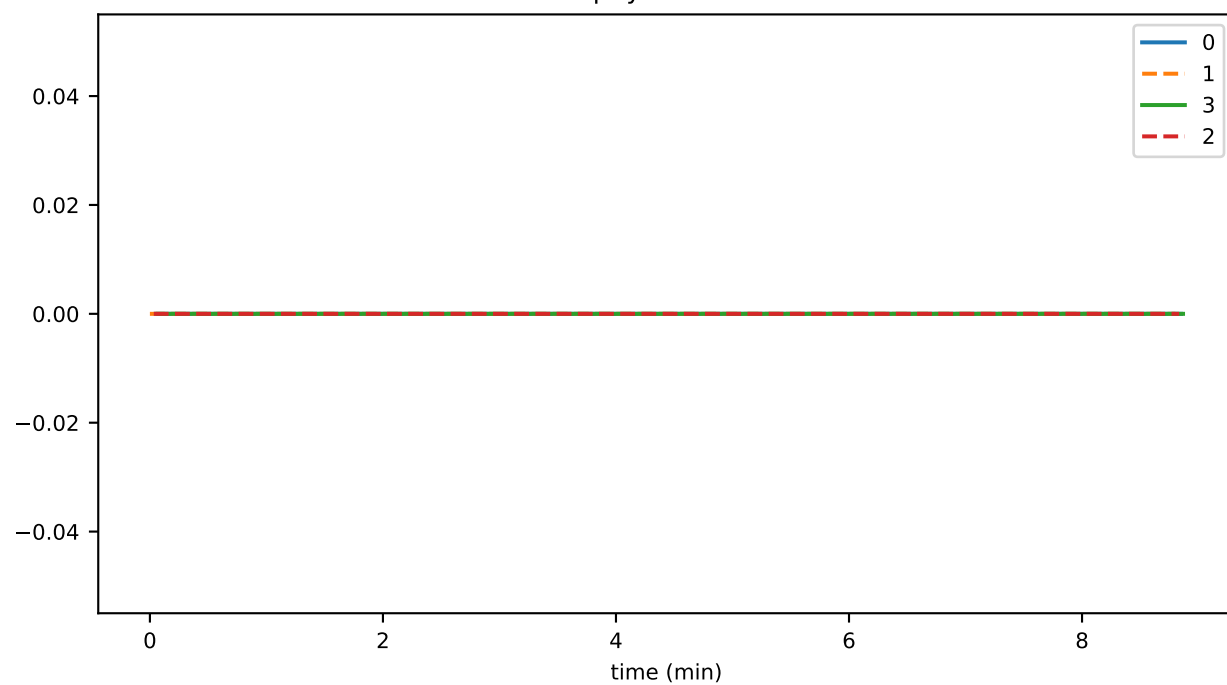
pityParent3
