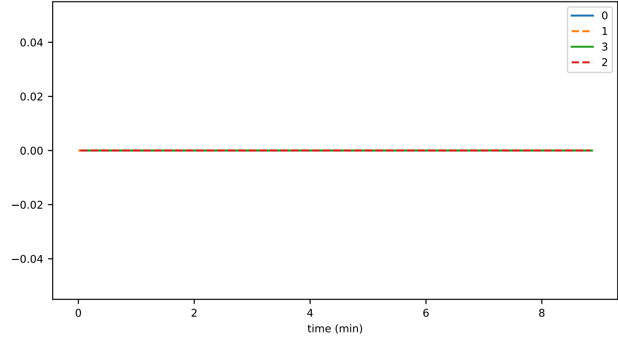
ev_per_syncR
