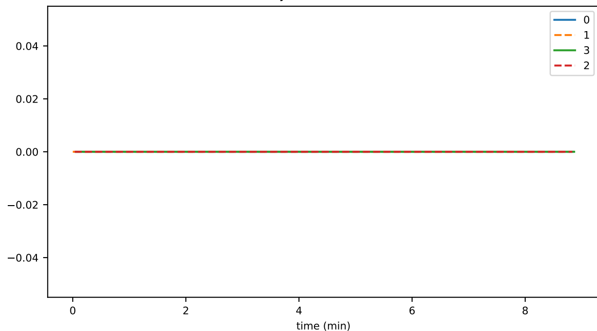
1e6 tokensMaxNumber
