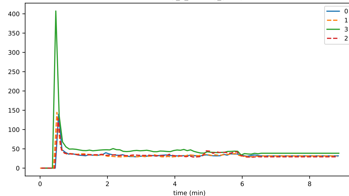
eventDelay_1_hashing_storage
