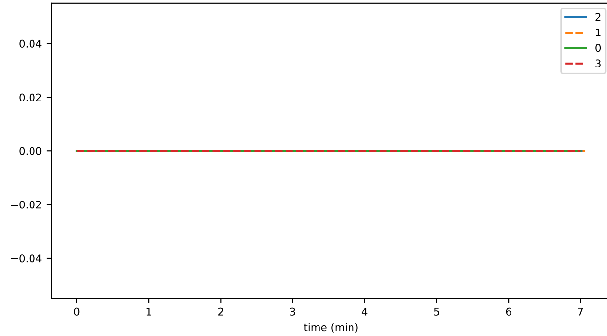
tokenCreateThrottledTxns
