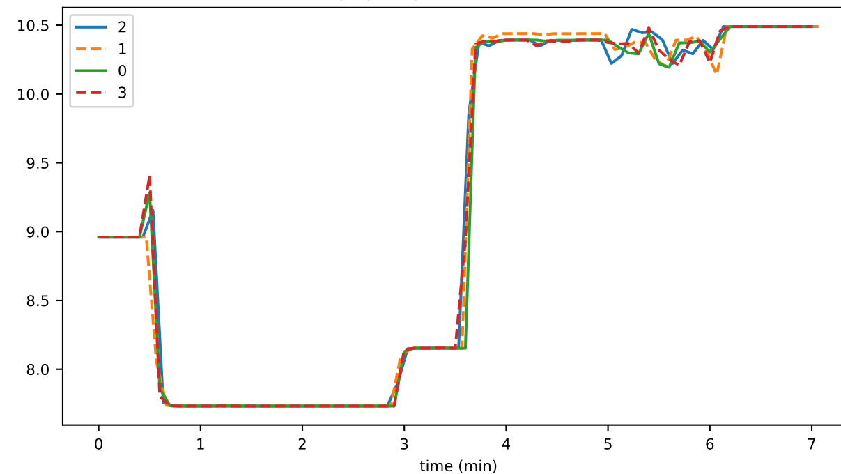
hapiBalanceQueryLimitsPercentUsed
