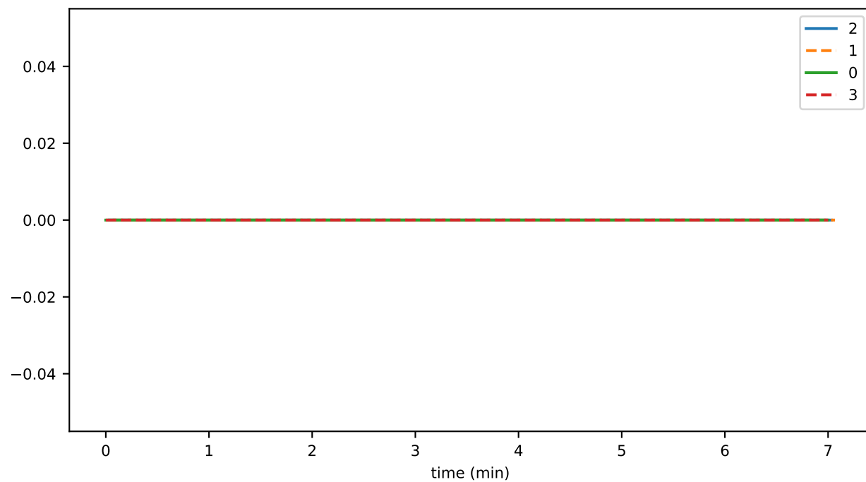
tokenGetNftInfoThrottledTxns
