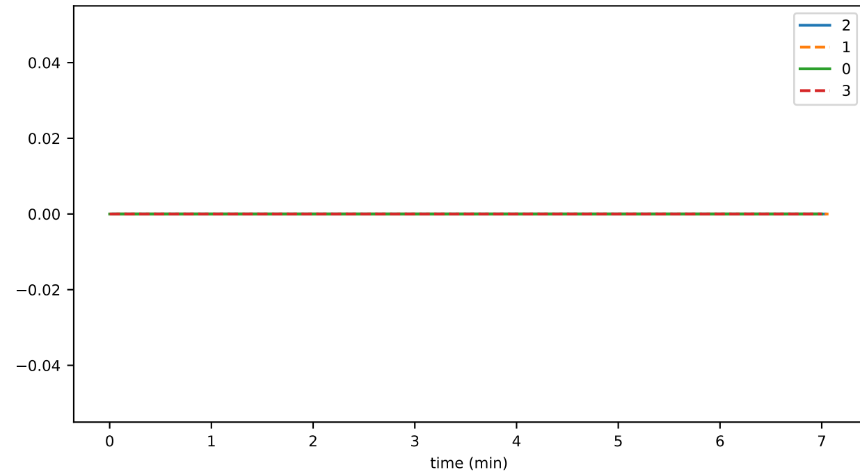
SmartContractService:SystemContractMethodCall_IS_AUTHORIZED_total
