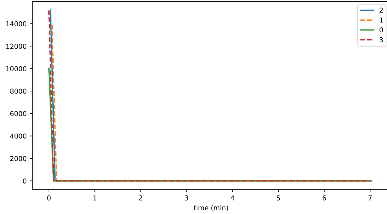
eventDelay_2_validation_gossipMAX
