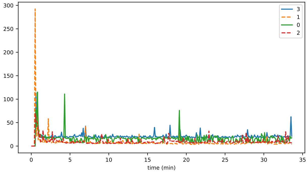
eventDelay_1_eventCreation_runtimeMAX
