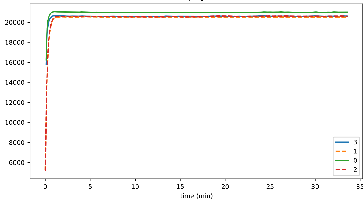
ping_us_00MIN
