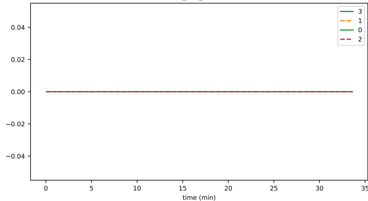
ev_per_syncS
