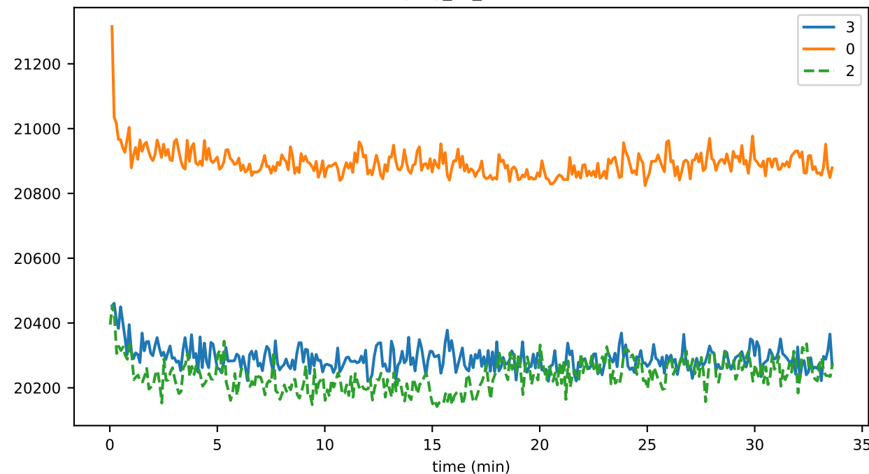
ping_us_02MIN
