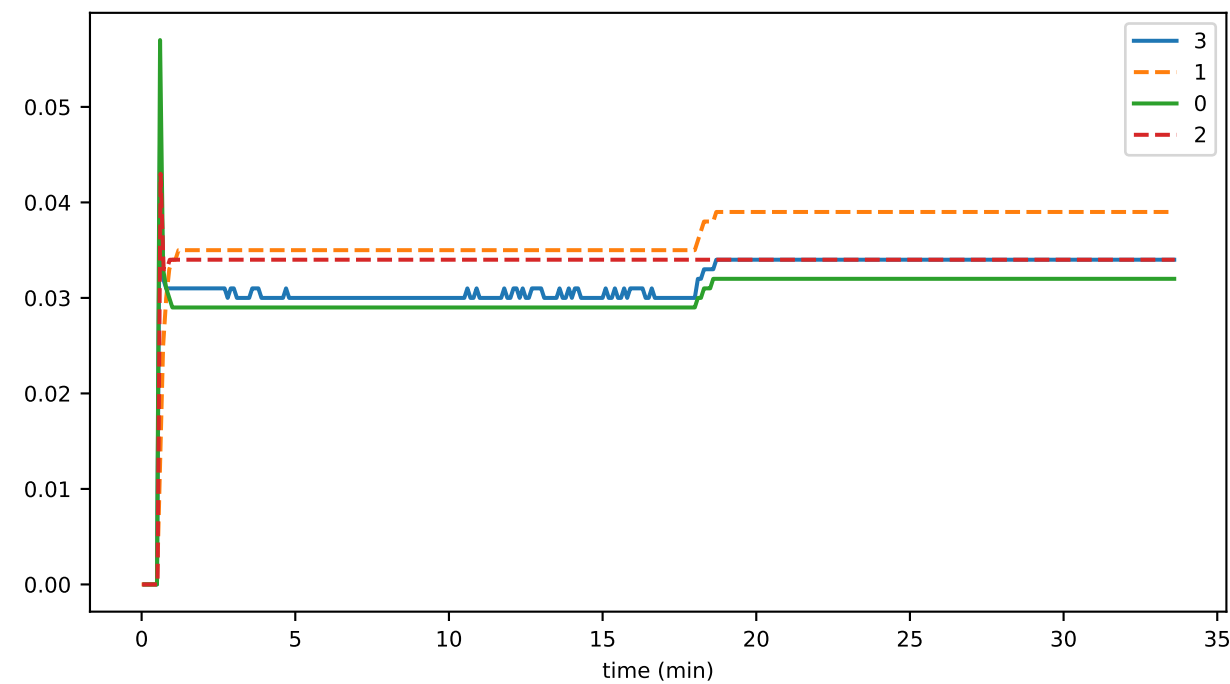
secR2F
