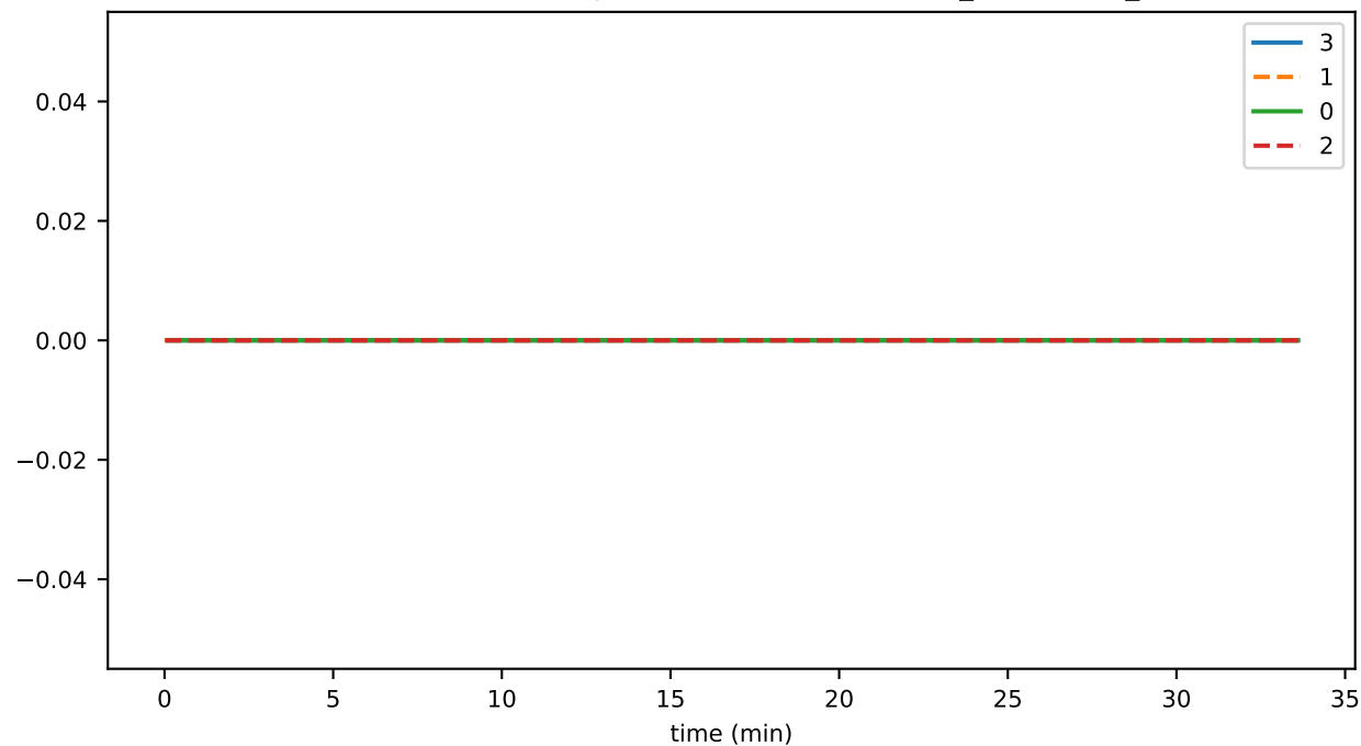
SmartContractService:SystemContractMethodCall_TOKEN_QUERY_total
