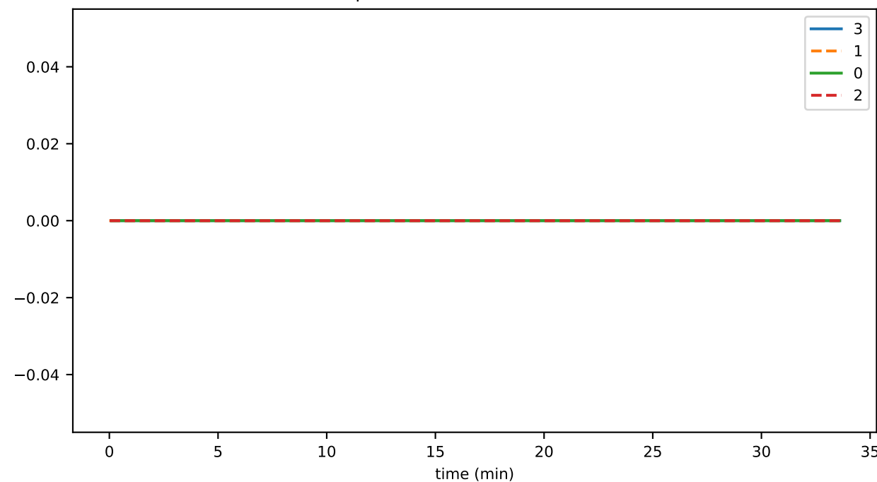
hapiGasPercentUsed
