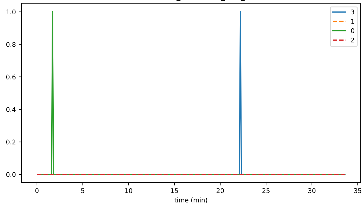
PlatformMonitor_unhandled_task_count
