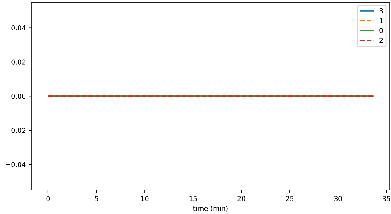
conn_connClose_configUpdate
