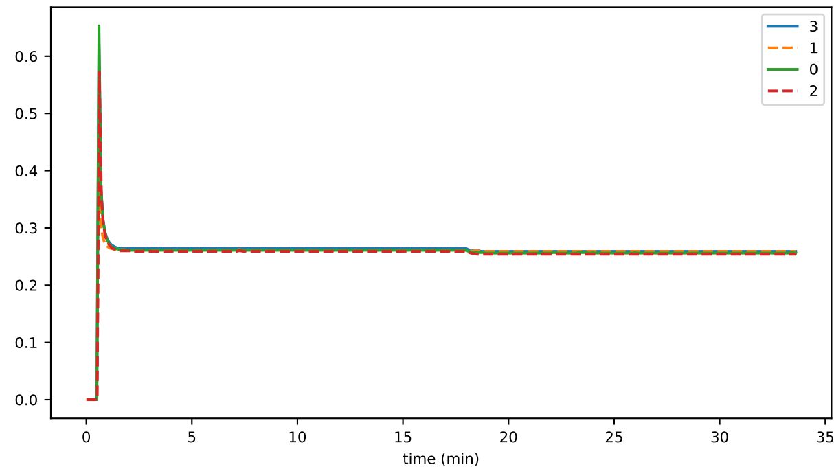
secC2RC
