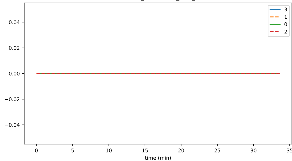
StateHasher_unhandled_task_count
