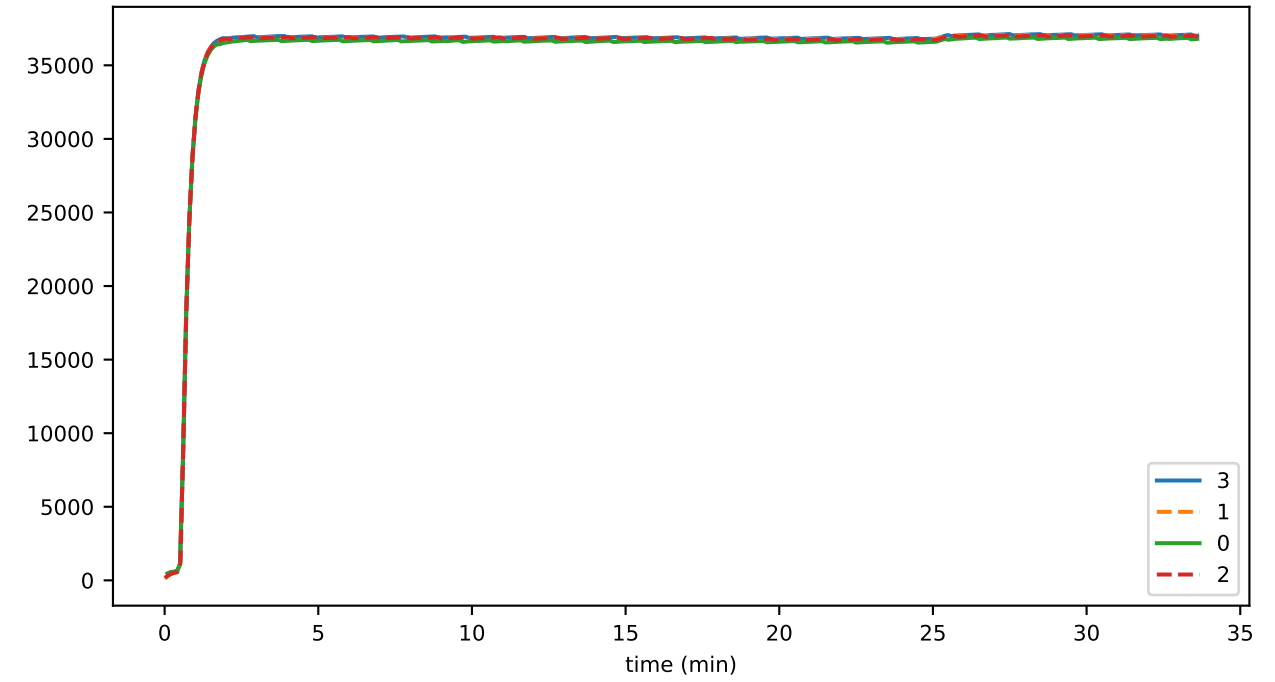
bytes_per_sec_sent_01
