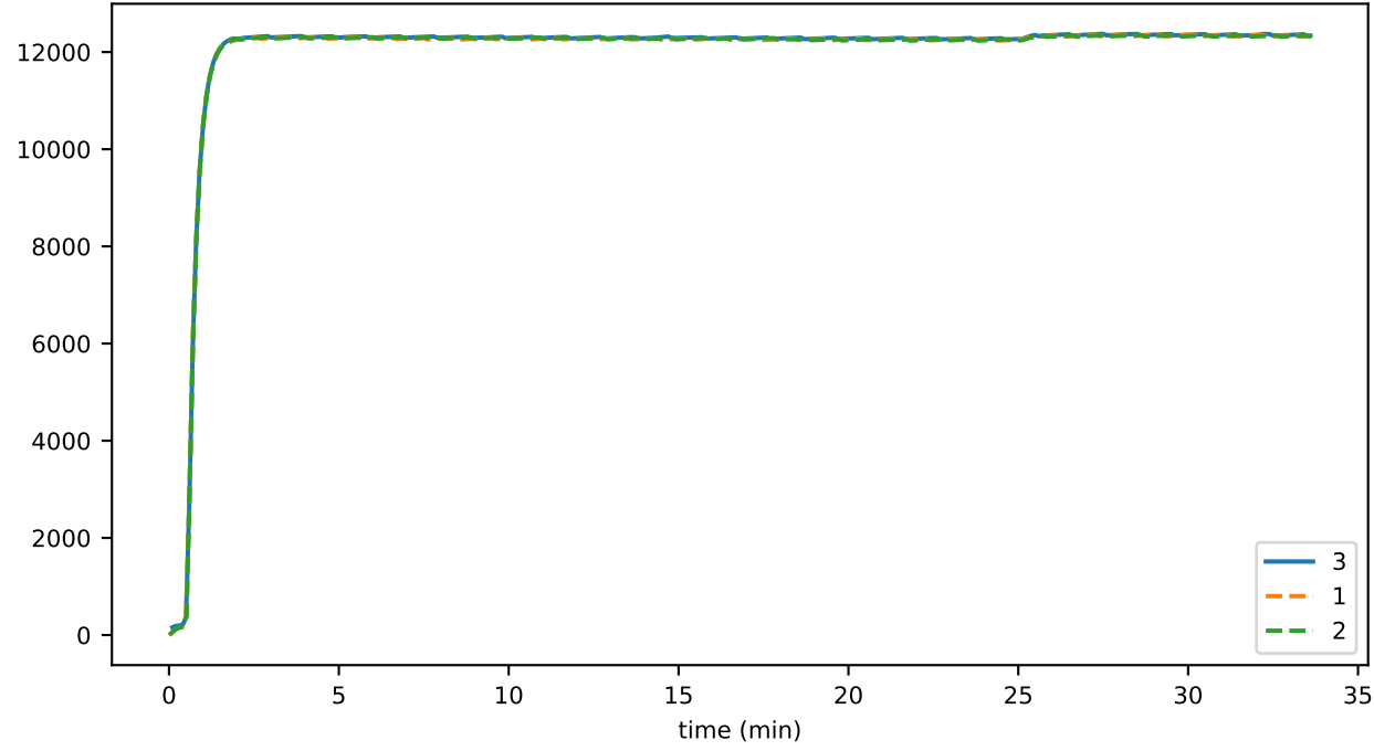
bytes_per_sec_sent_00
