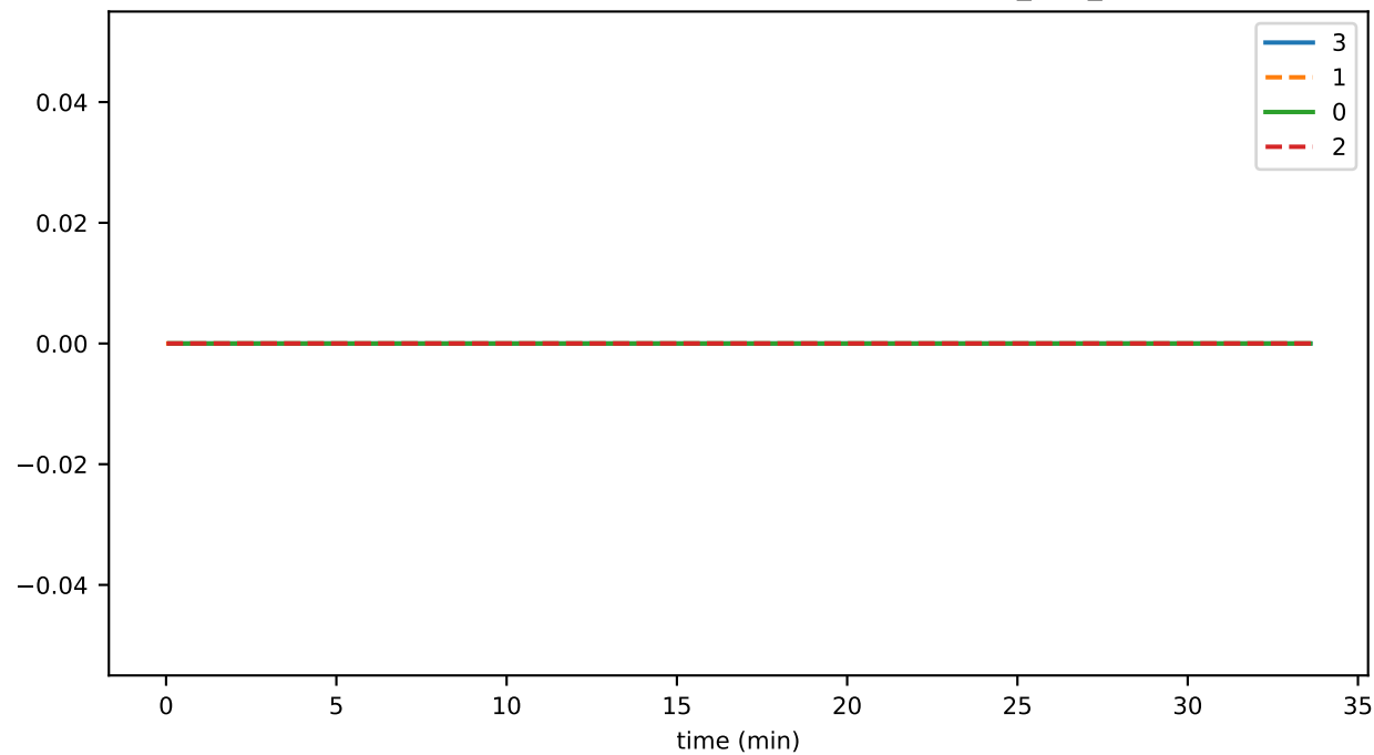
SmartContractService:SystemContractMethodCall_HTS_total
