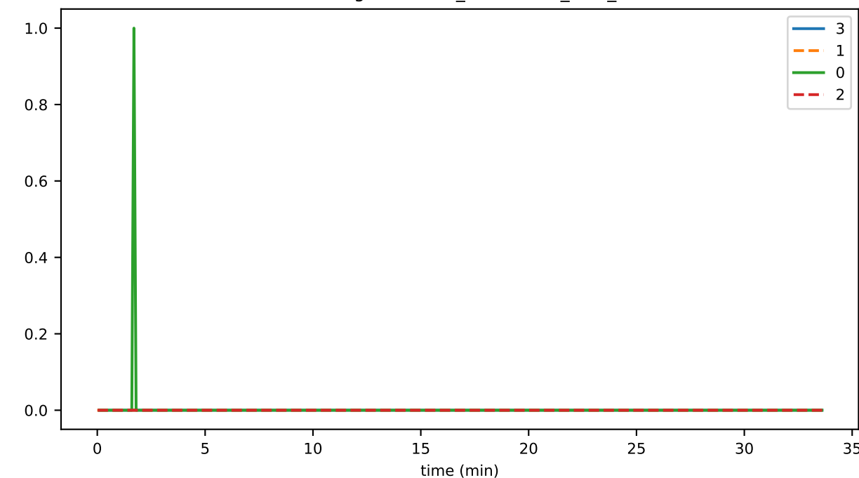
StateHasher_unhandled_task_count
