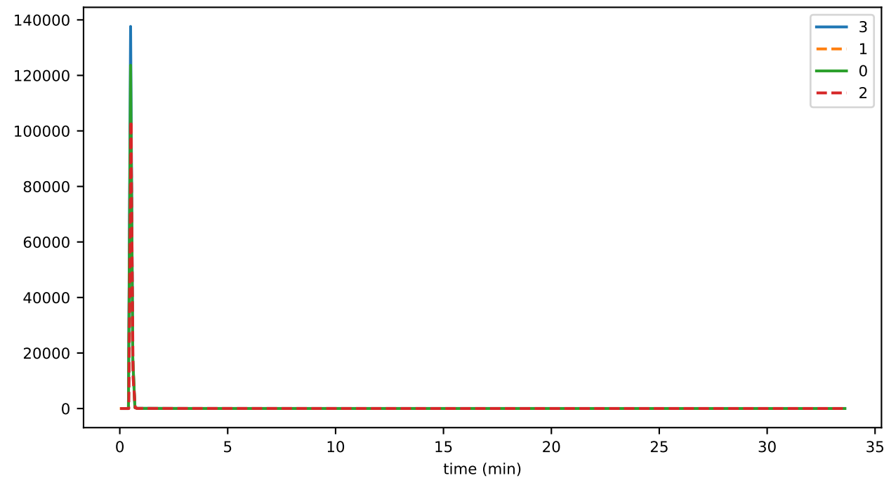
preHandleMicros
