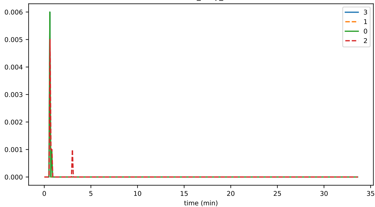
StateHasher_busy_fraction
