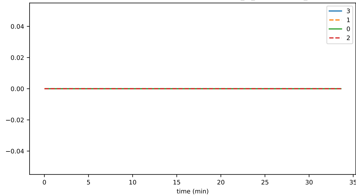
SmartContractService:SystemContractMethodCall_IS_AUTHORIZED_failed
