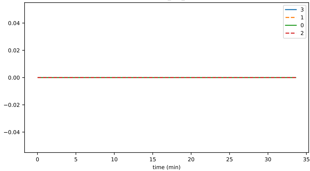
DigSpans_per_sec
