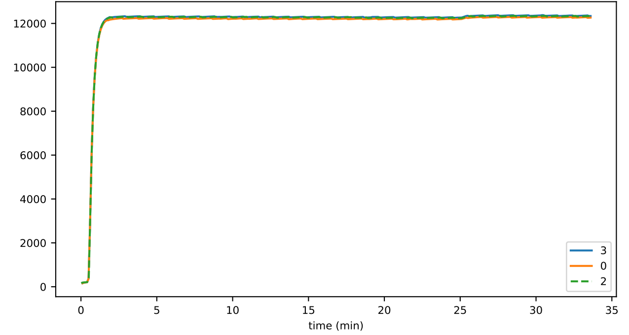
bytes_per_sec_sent_01
