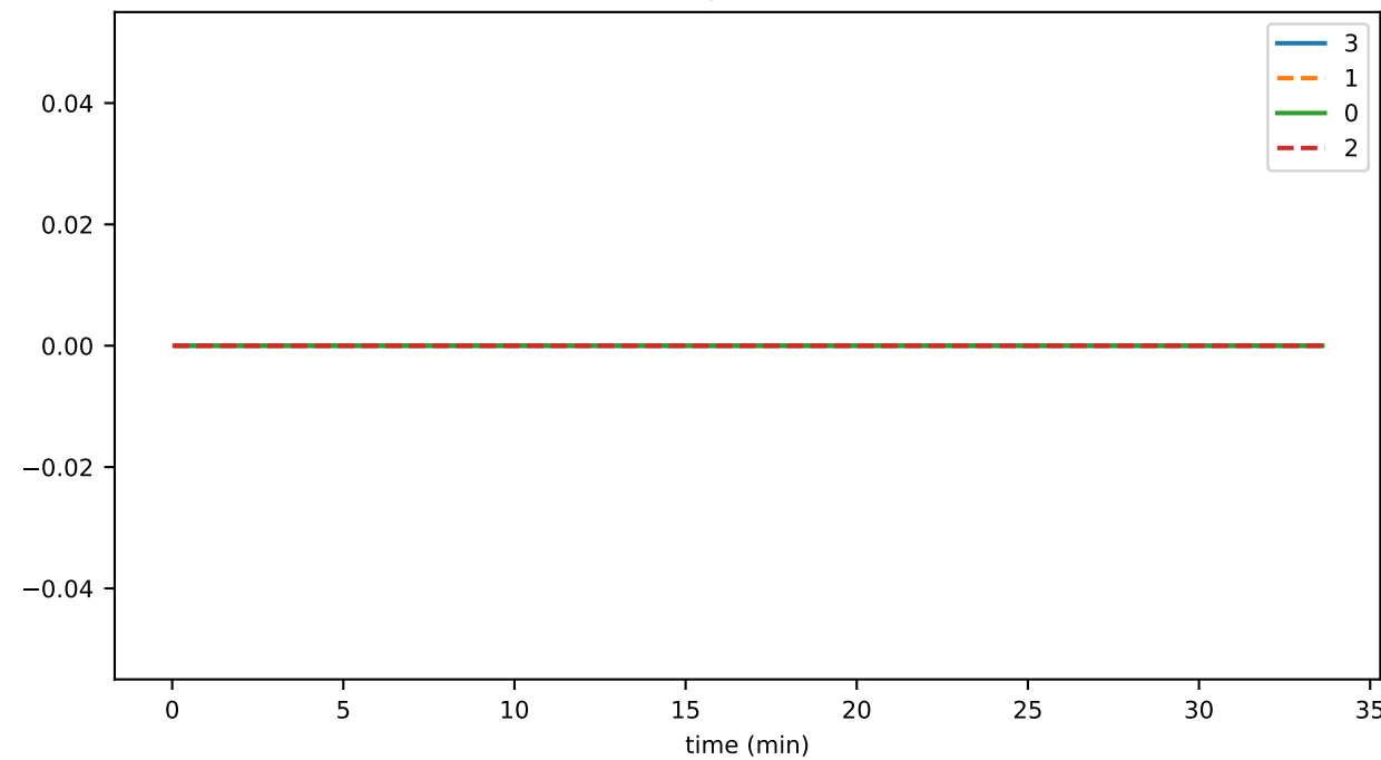
DigSubWrkItmTime
