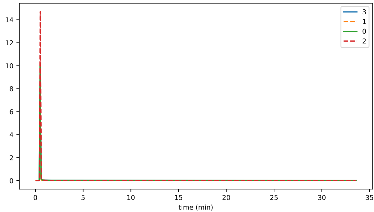
secC2R
