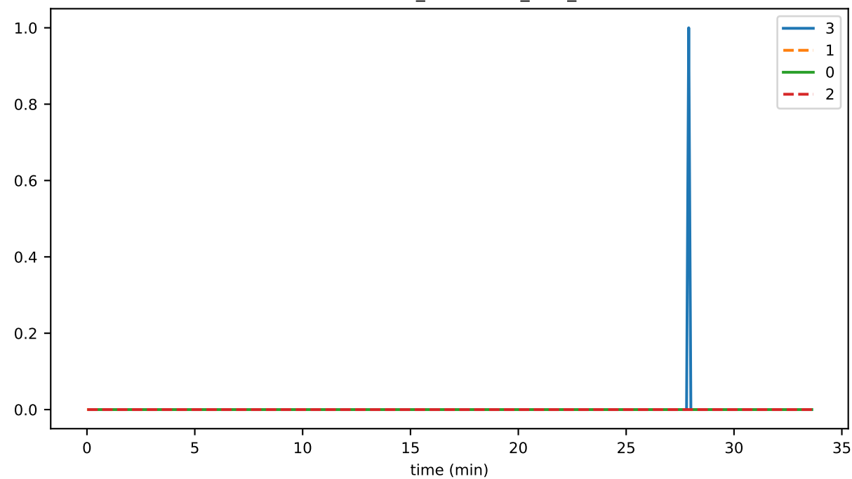
InlinePcesWriter_unhandled_task_count
