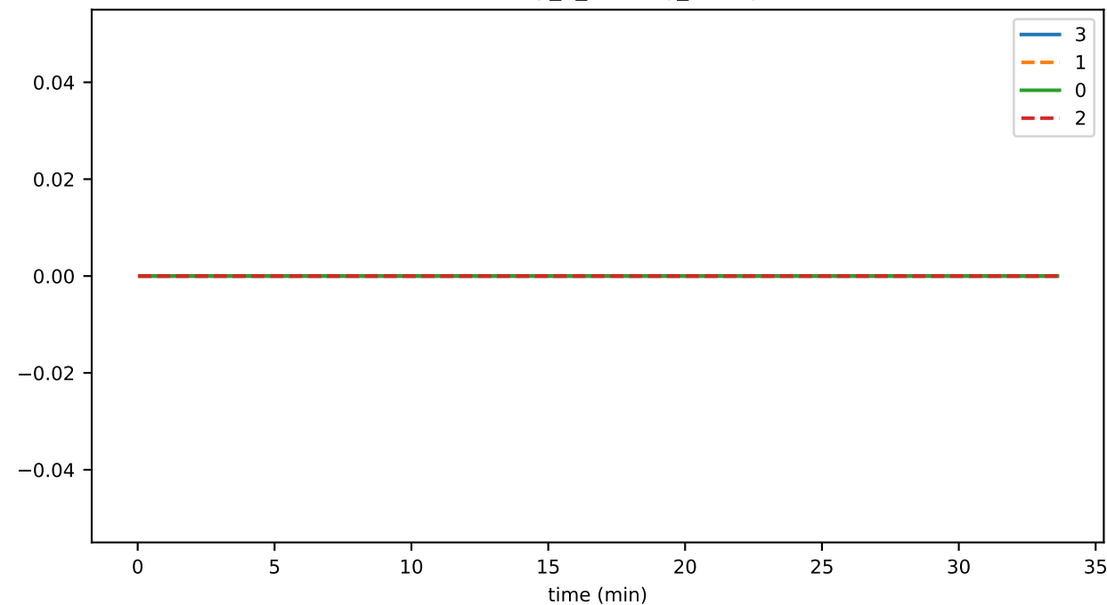
eventDelay_2_validation_gossip
