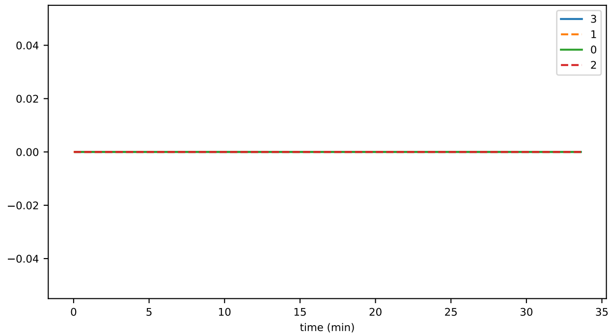
secC2R
