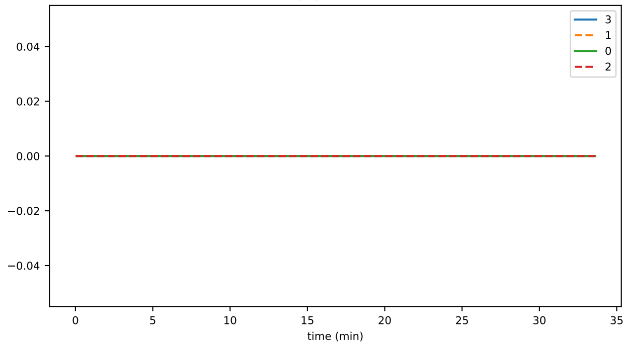
PlatformMonitor_unhandled_task_count
