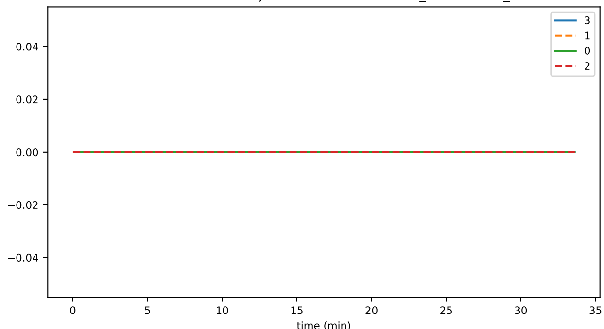
SmartContractService:SystemContractMethodCall_ALLOWANCE_total
