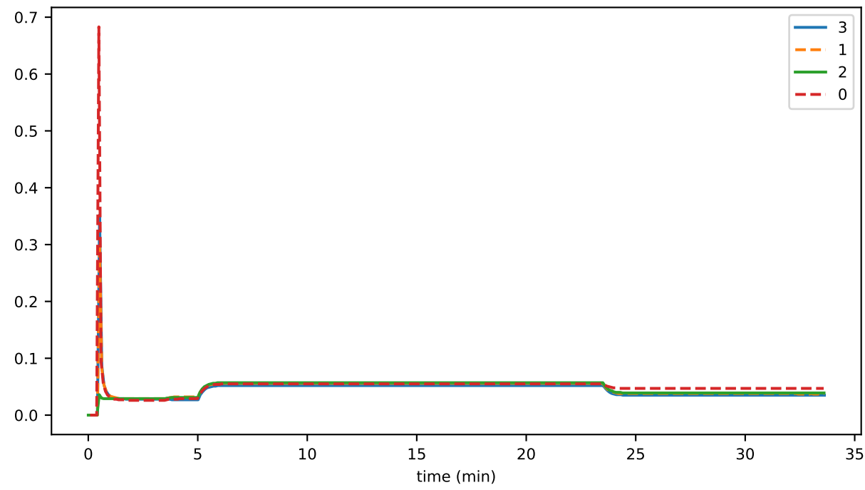
secC2R
