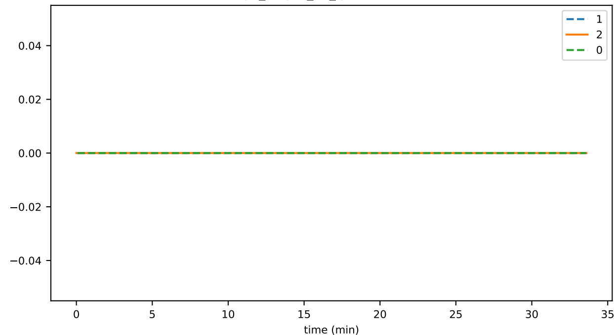
rpc_output_queue_poll_timeMAX
