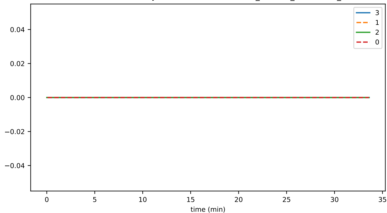
SmartContractService:SystemContractMethodCall_HAS_total
