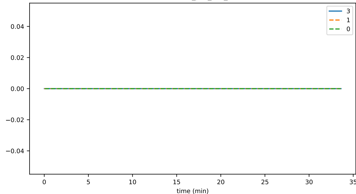
DiskspaceFree
