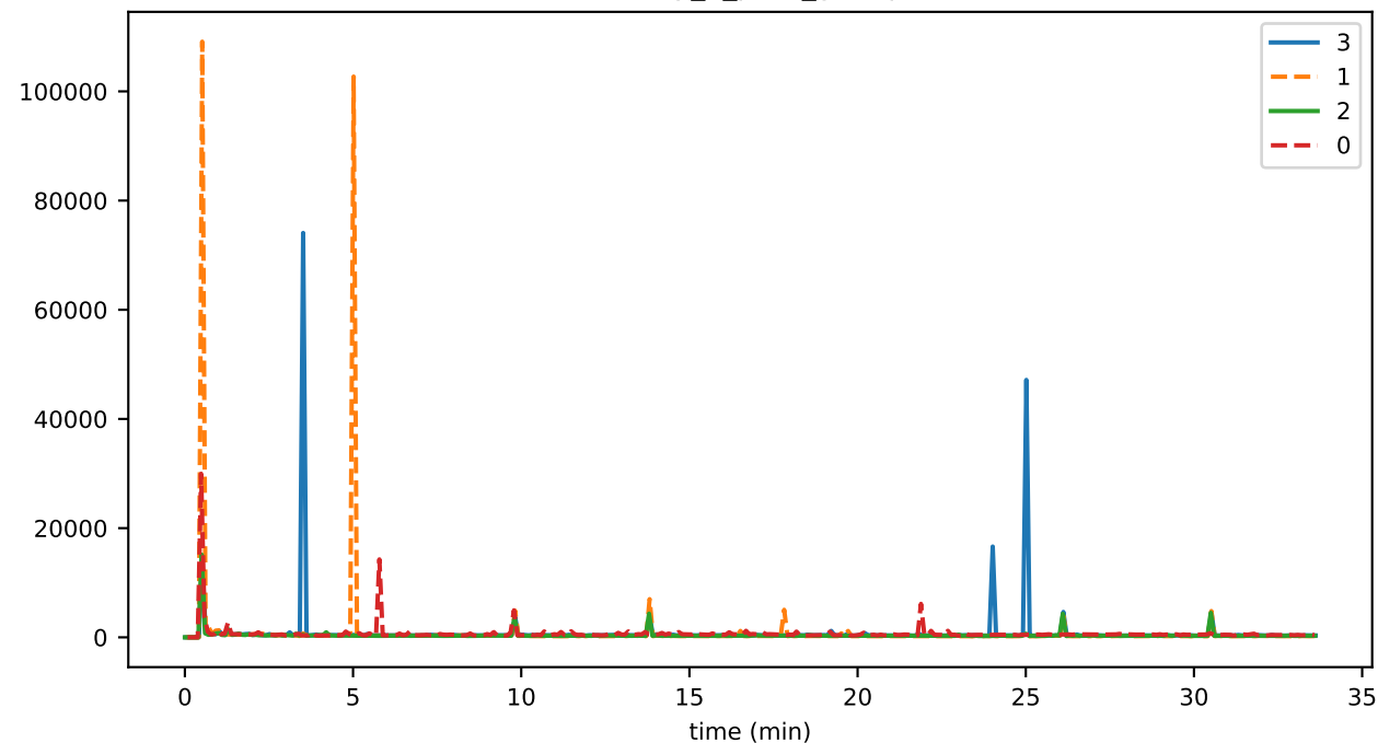
eventDelay_6_pces_runtimeMAX
