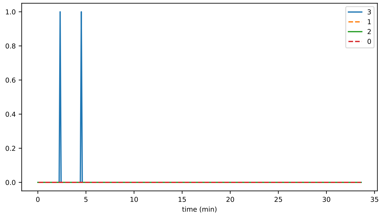
syncRoundLag
