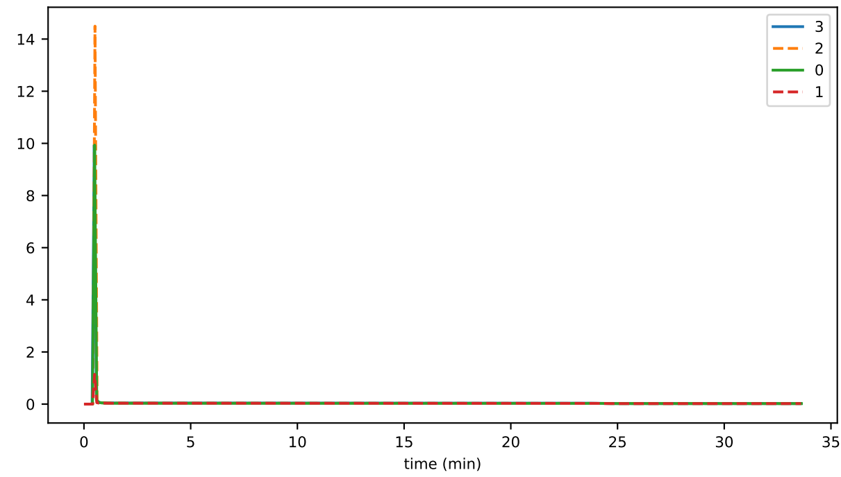
secC2R
