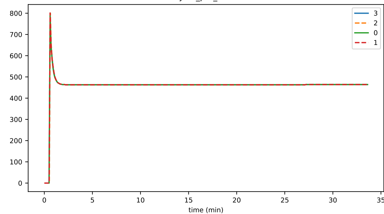
bytes_per_trans
