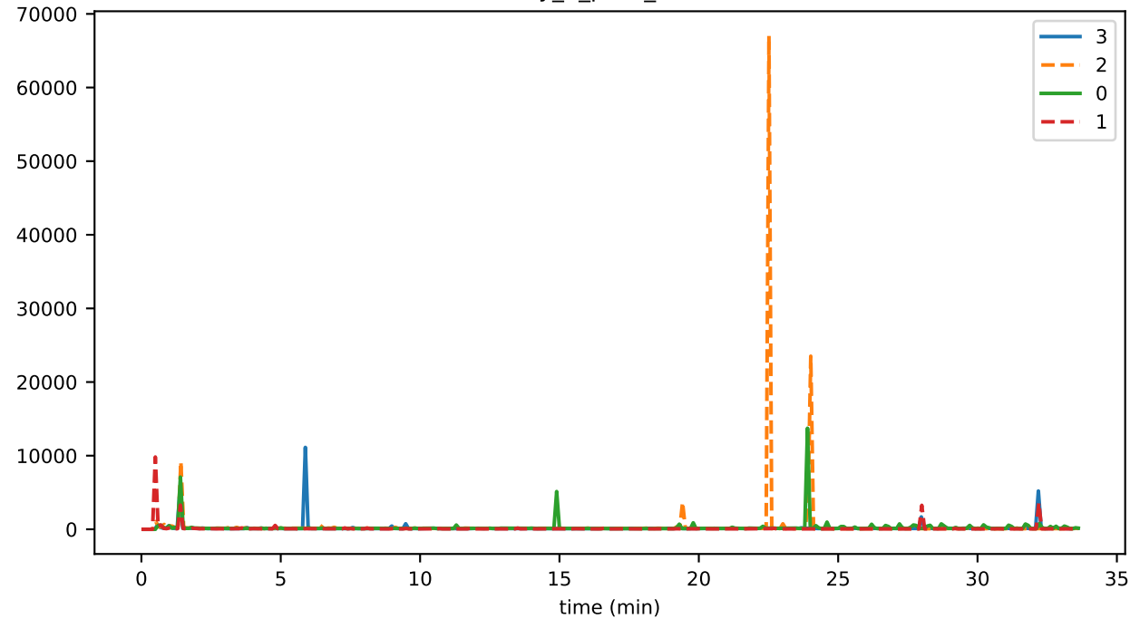
eventDelay_6_pces_runtimeMAX
