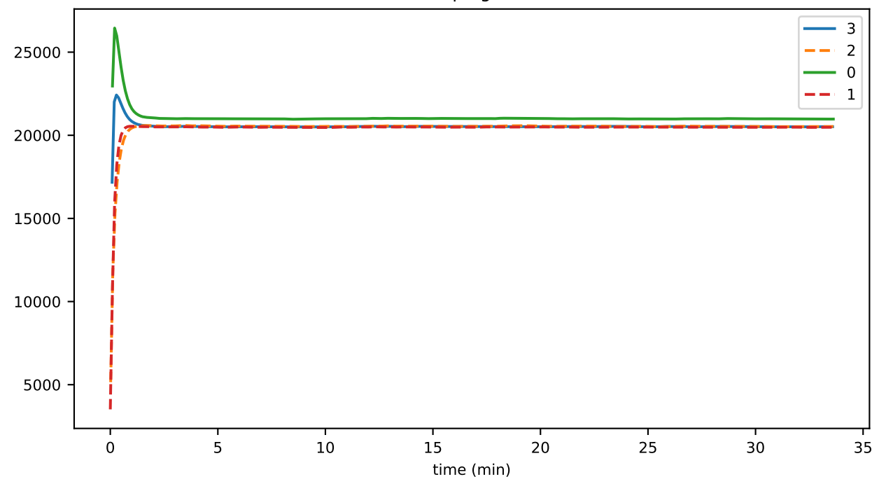
ping_us_00MIN
