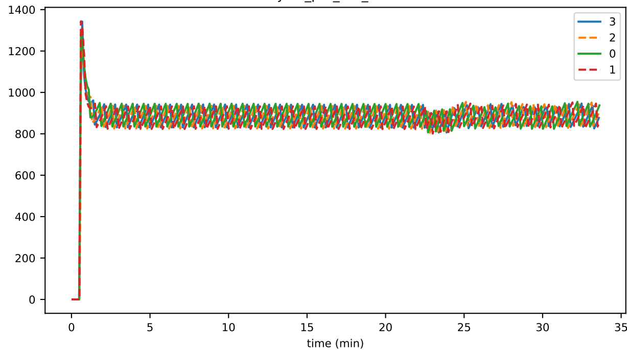
bytes_per_sec_trans
