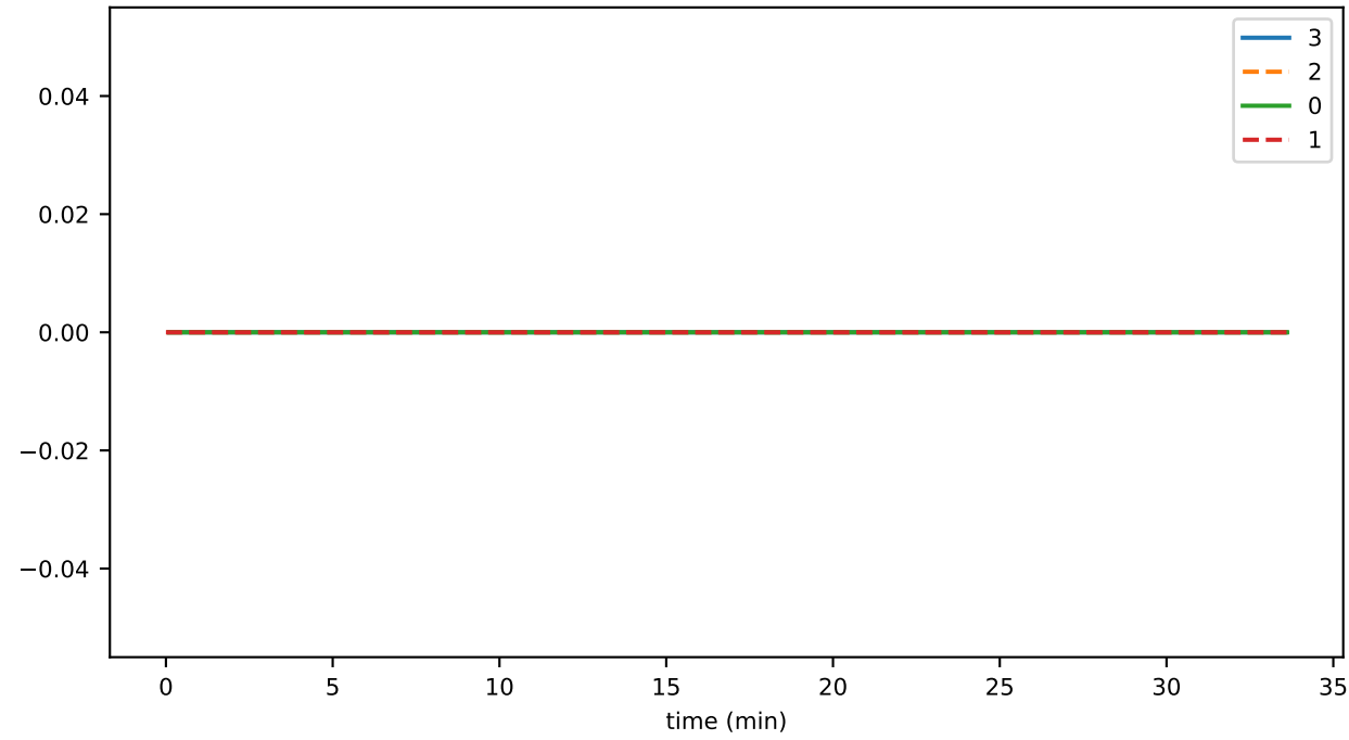
conn_connClose_tooManyEndStreamResponses
