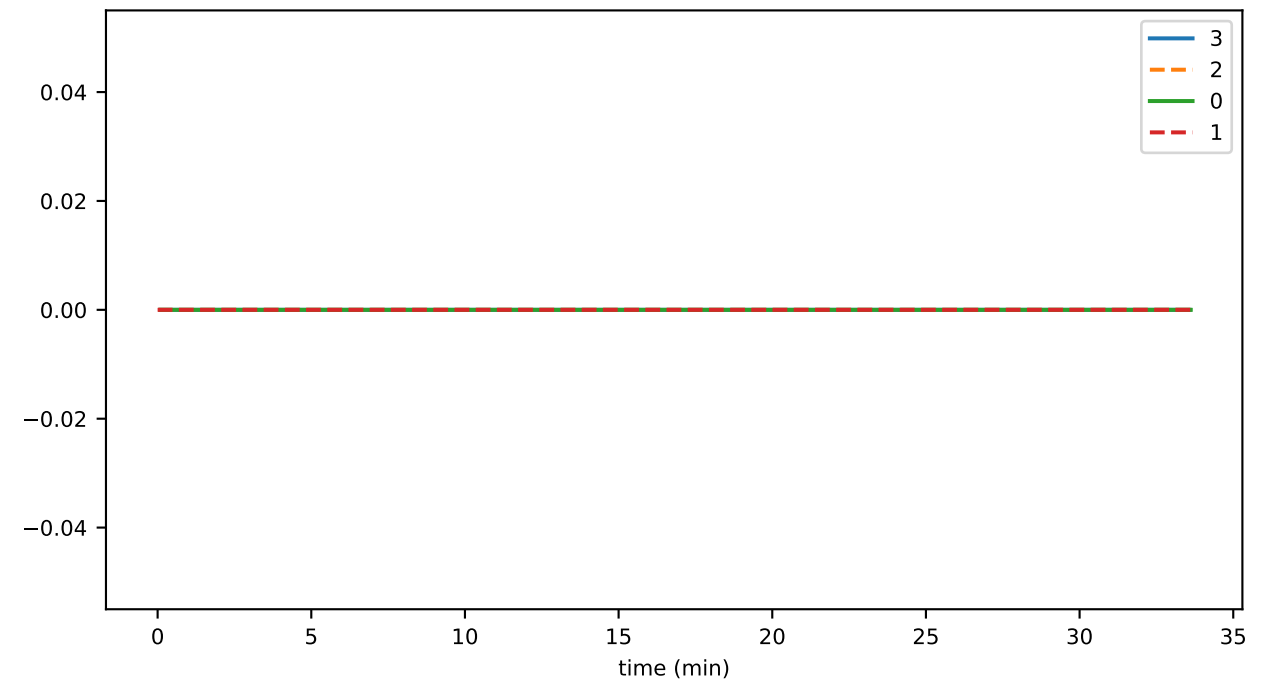
hapiGasPercentUsed
