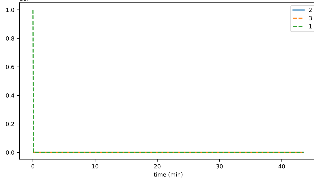
ping_us_00MIN
