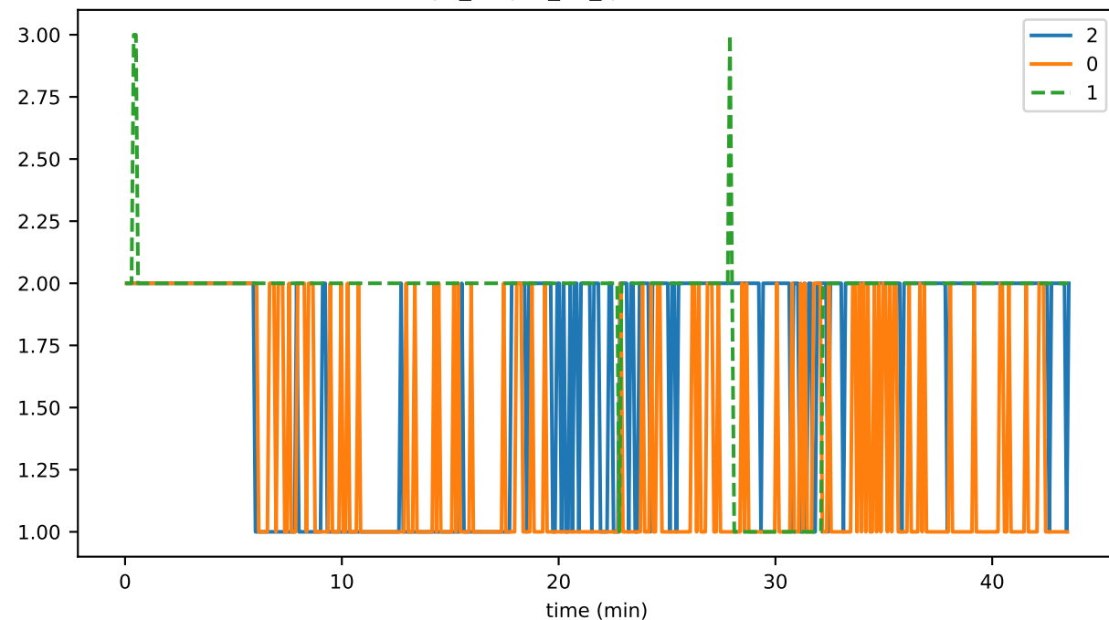
rpc_output_queue_poll_time
