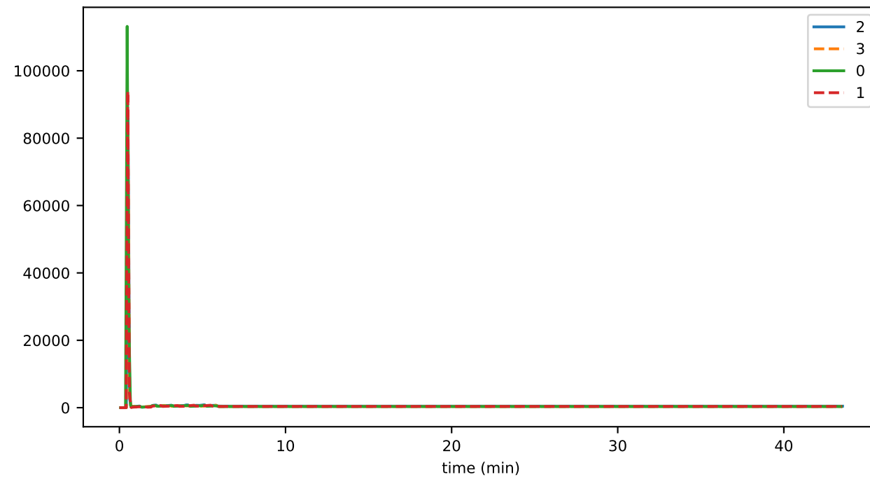
preHandleMicros
