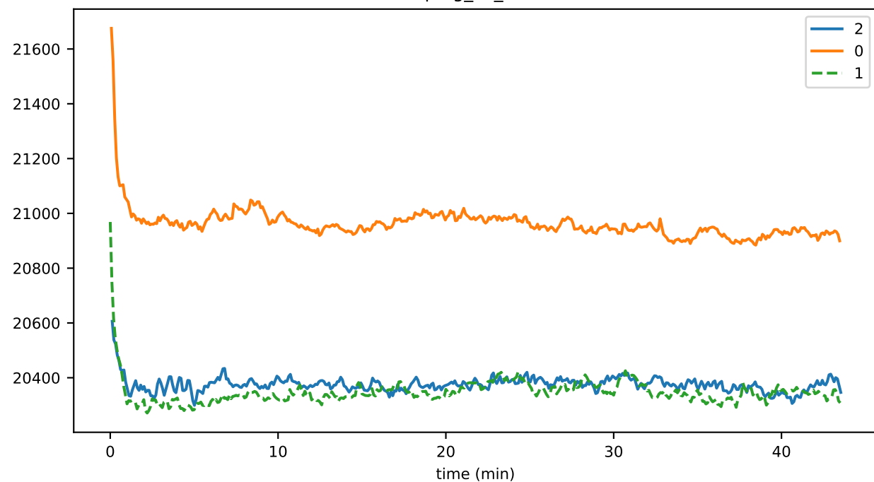
pityParent0
