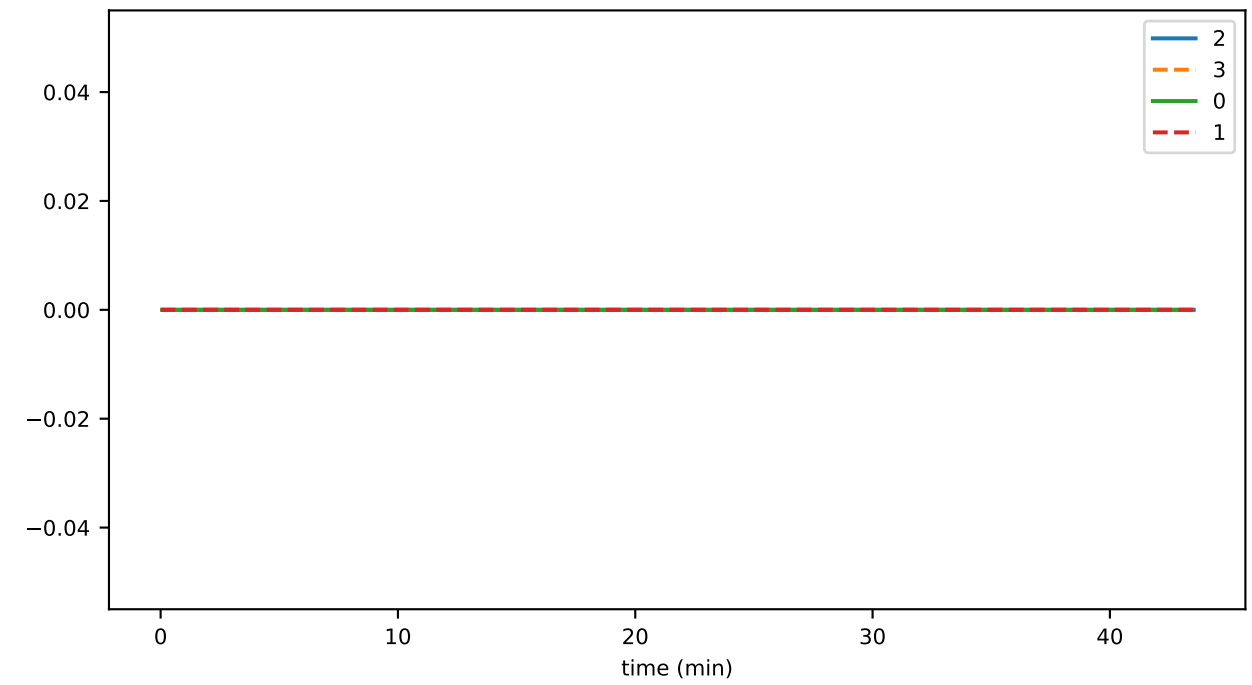
contractsUsed
