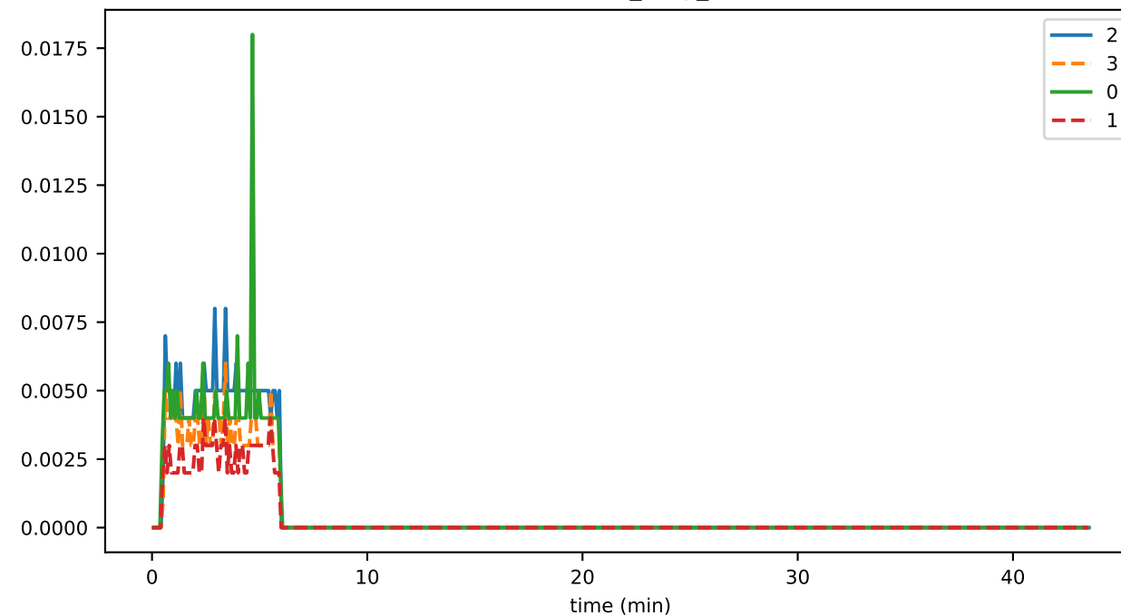
InternalEventValidator_unhandled_task_count
