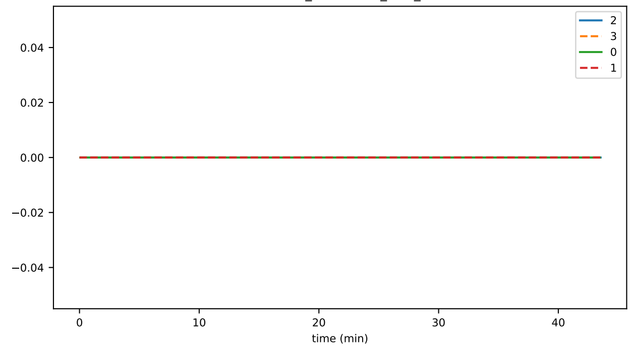
EventHasher_unhandled_task_count
