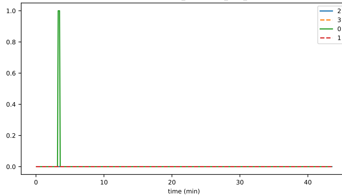
InternalEventValidator_unhandled_task_count
