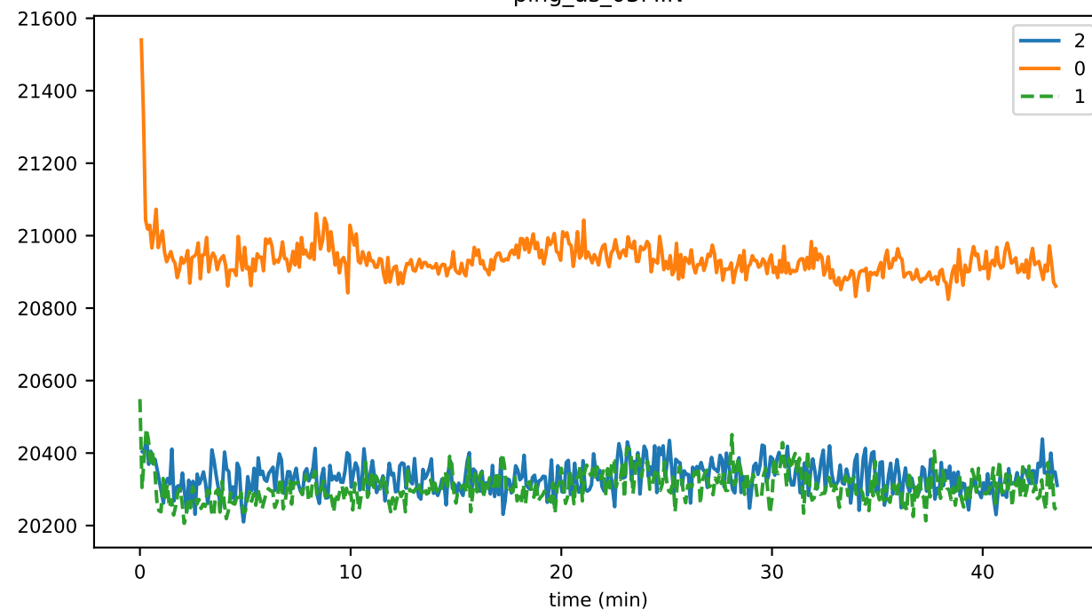
pityParent1
