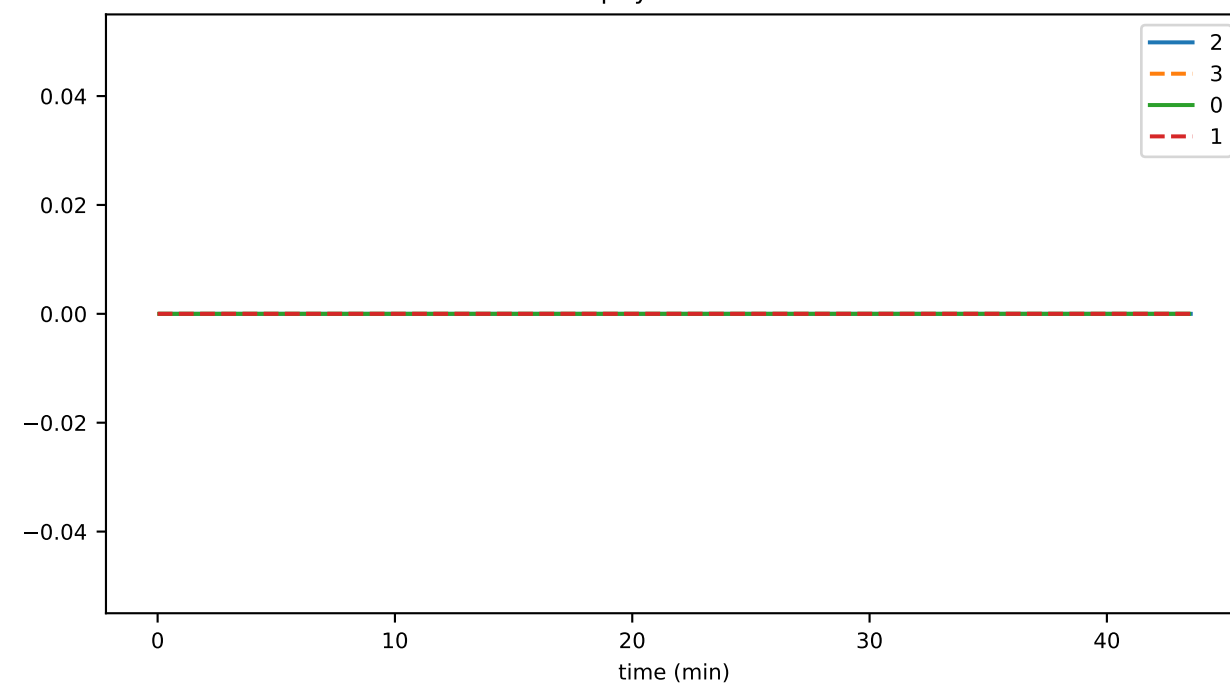
pityParent1
