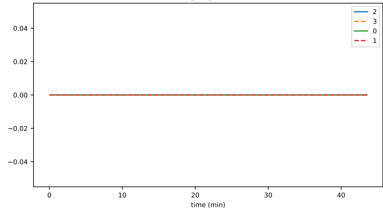
ev_per_syncS
