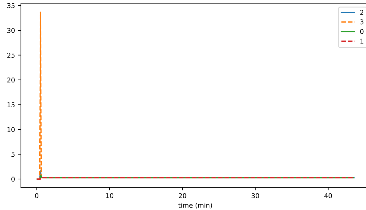
secC2RC
