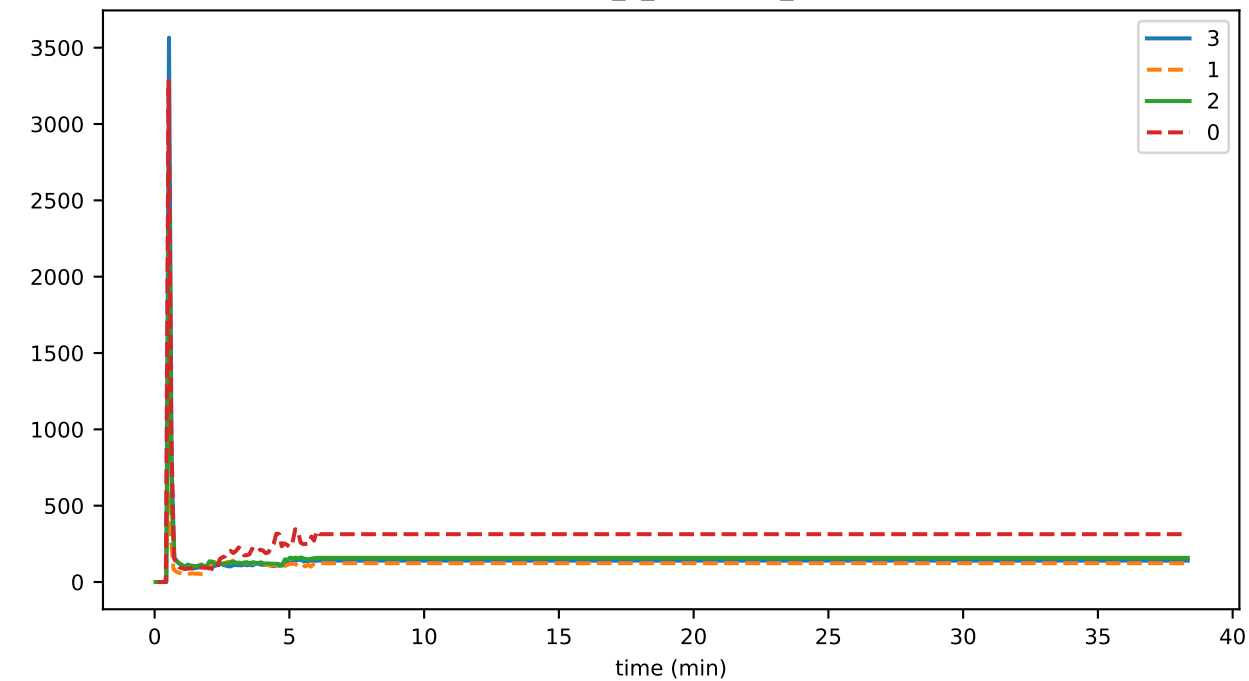
eventDelay_2_validation_gossip
