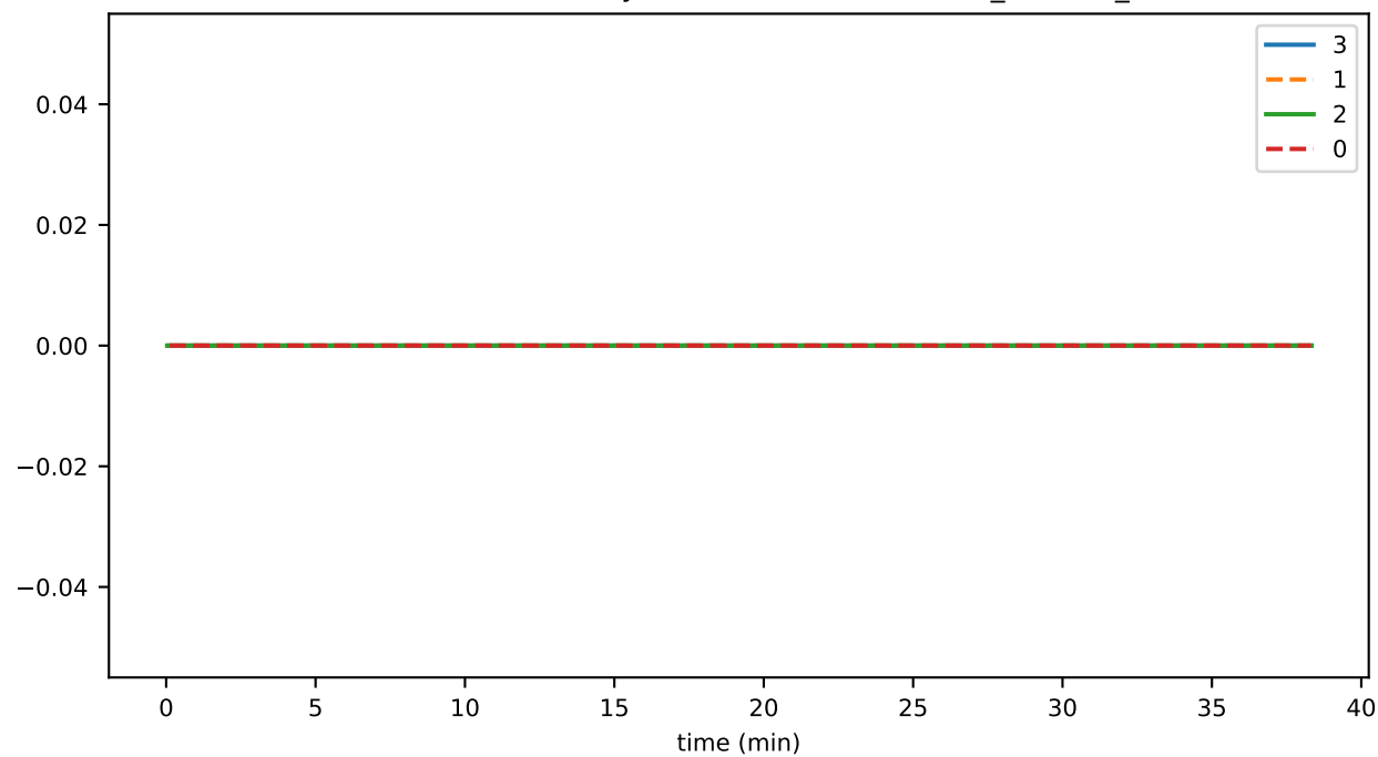
SmartContractService:SystemContractMethodCall_ERC721_total
