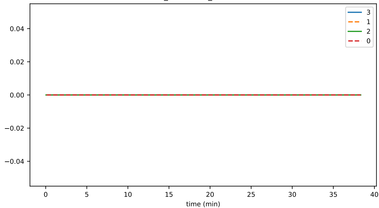
conn_connClose_internalError
