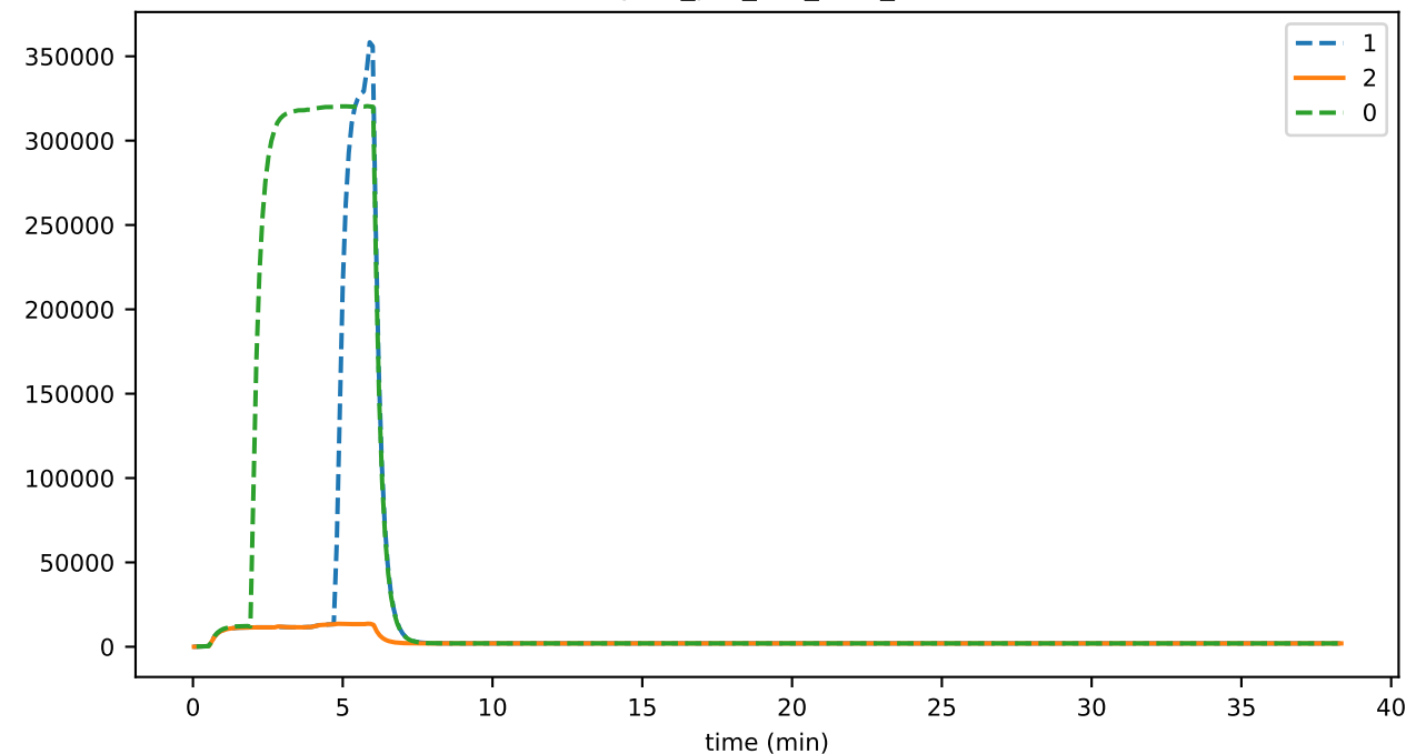
bytes_per_trans
