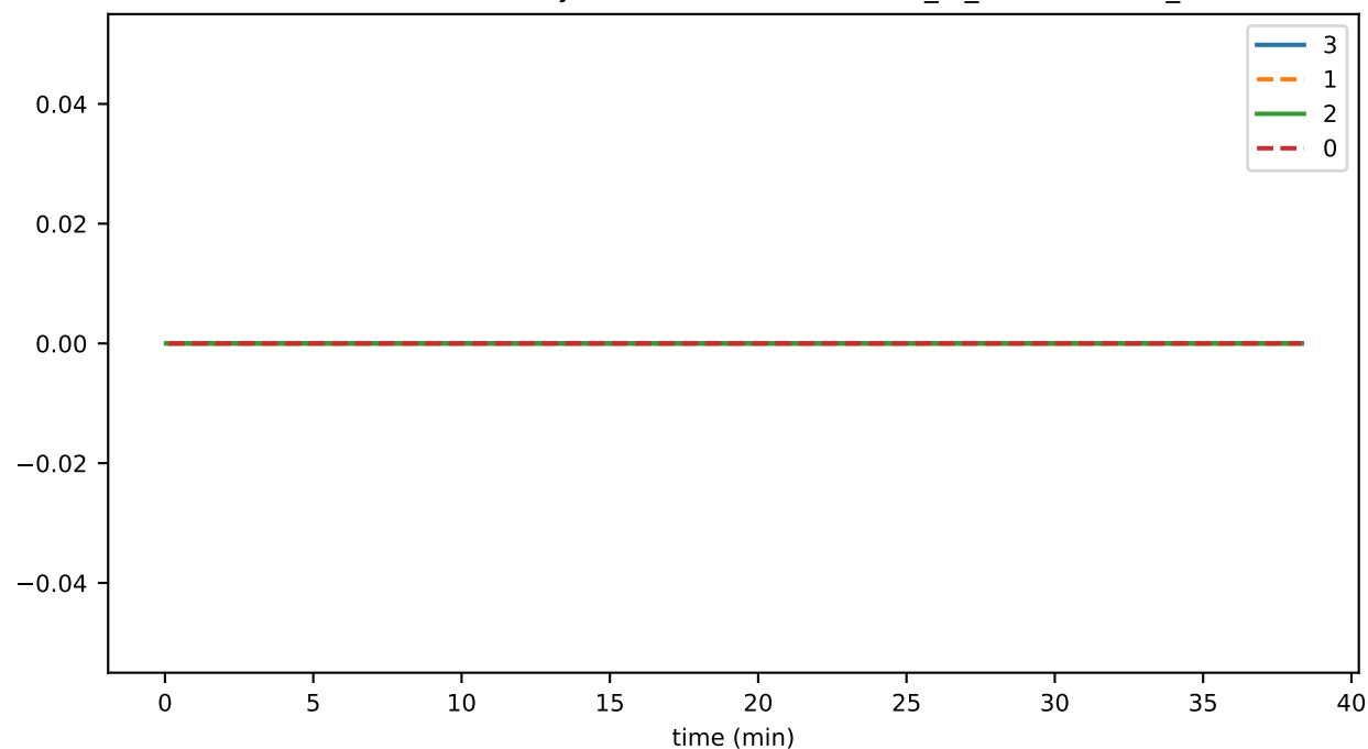
SmartContractService:SystemContractMethodCall_KYC_total
