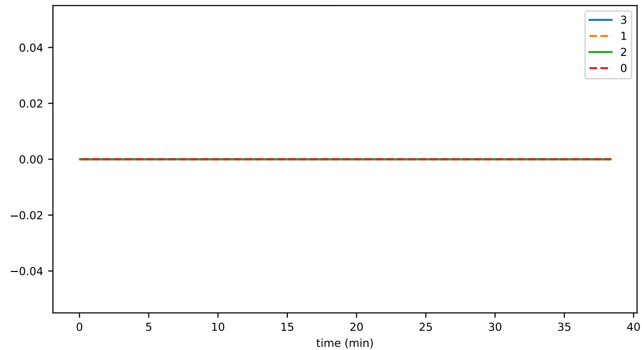
DigSubWrkItmTime
