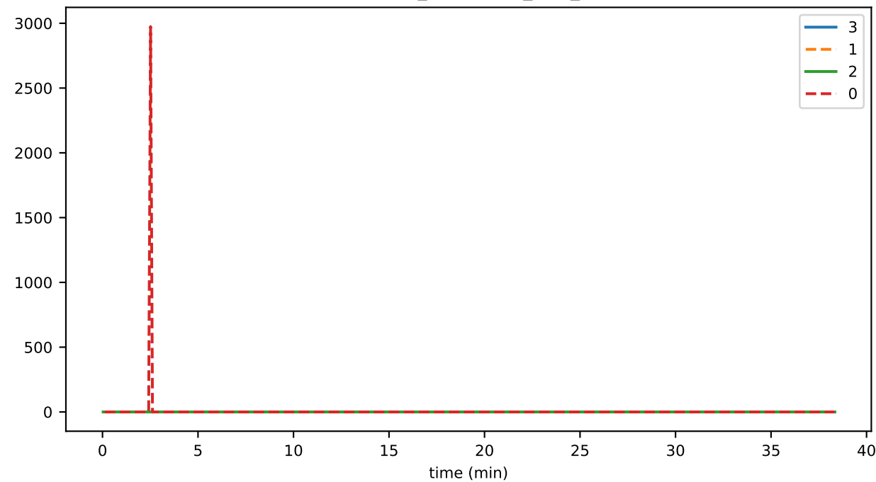
StateHasher_unhandled_task_count
