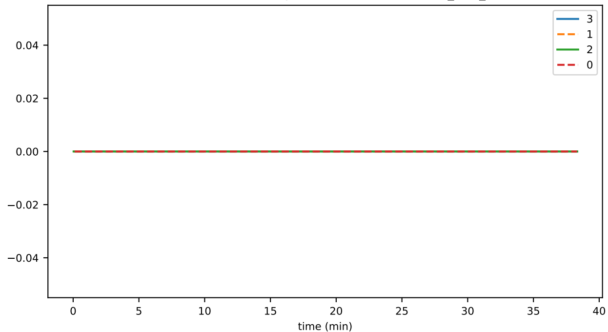
SmartContractService:SystemContractMethodCall_HTS_total
