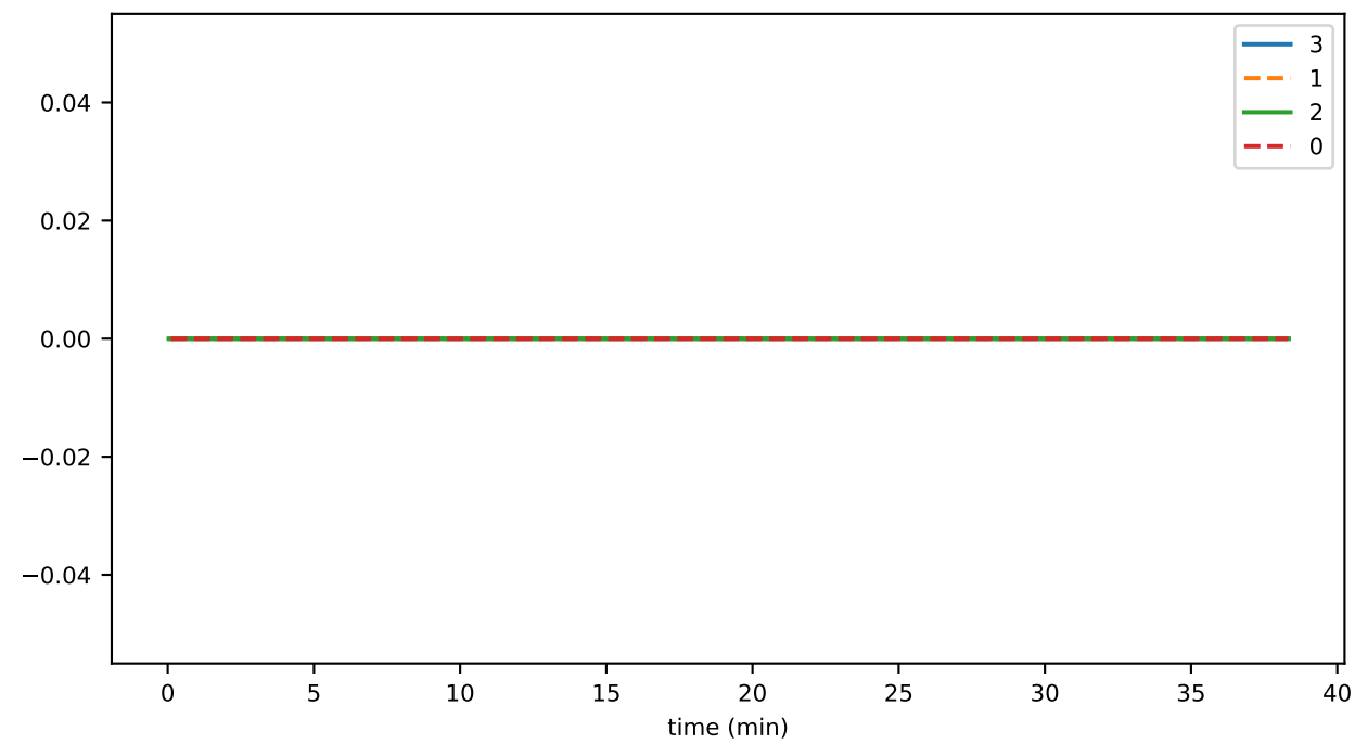
secC2RC
