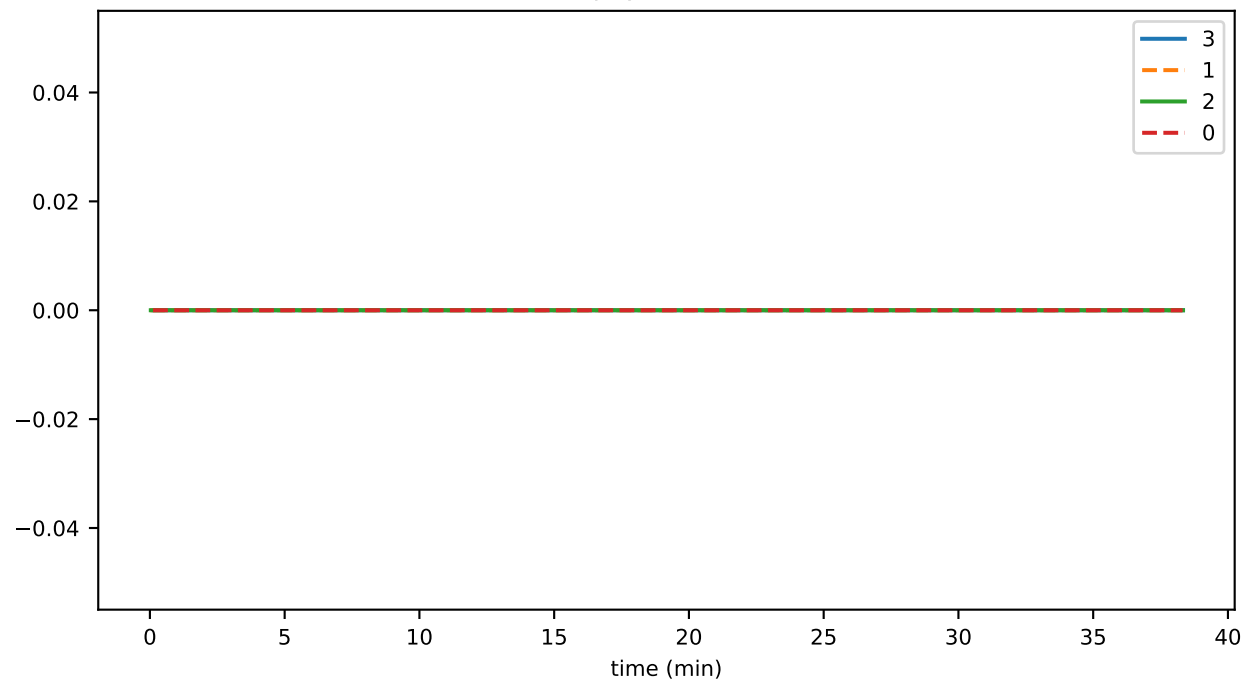
PlatformMonitor_unhandled_task_count
