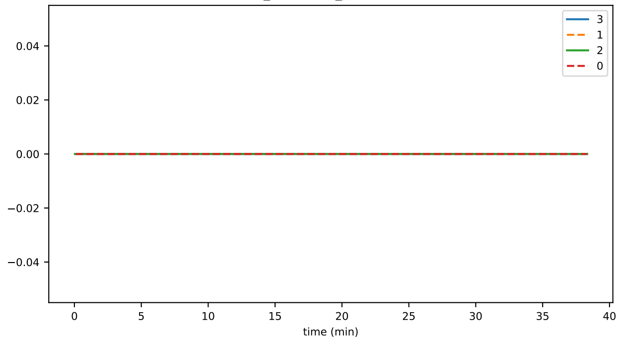
conn_connClose_tooManyEndStreamResponses
