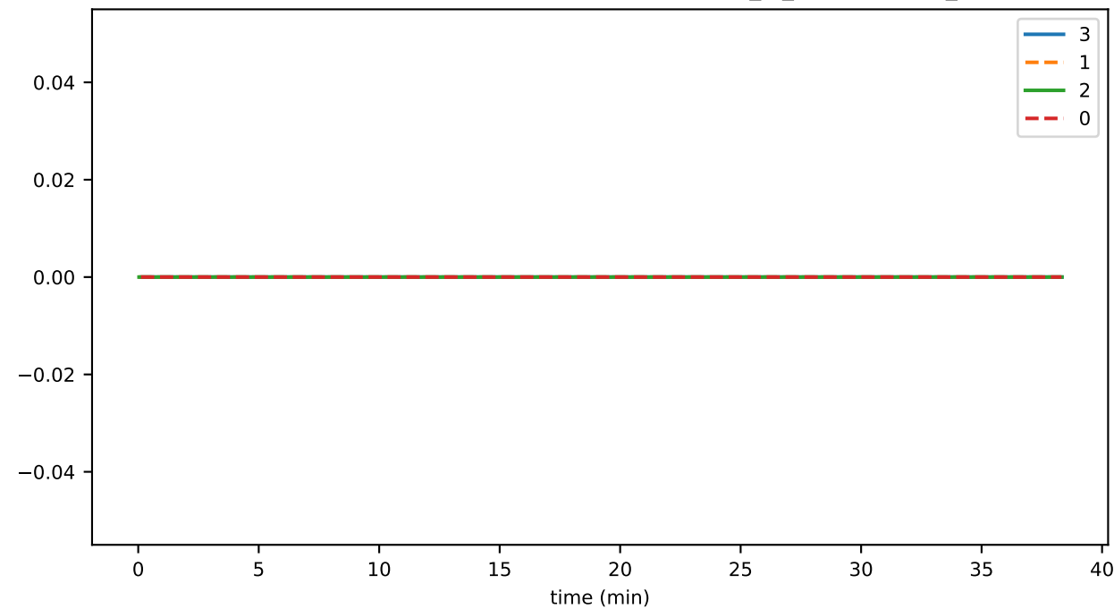
SmartContractService:SystemContractMethodCall_IS_AUTHORIZED_failed
