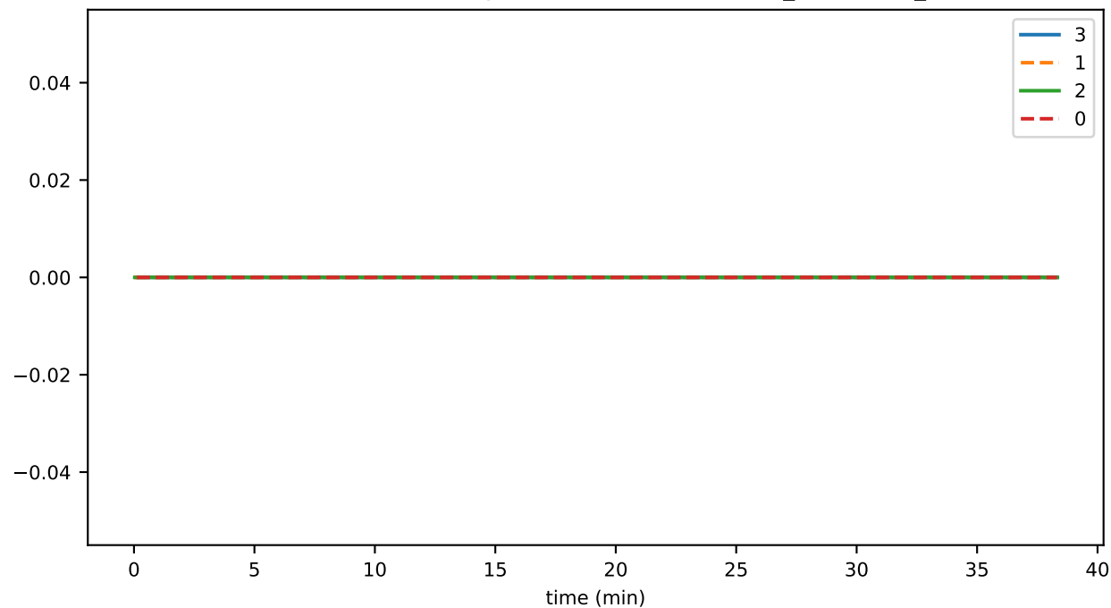
SmartContractService:SystemContractMethodCall_UPDATE_total
