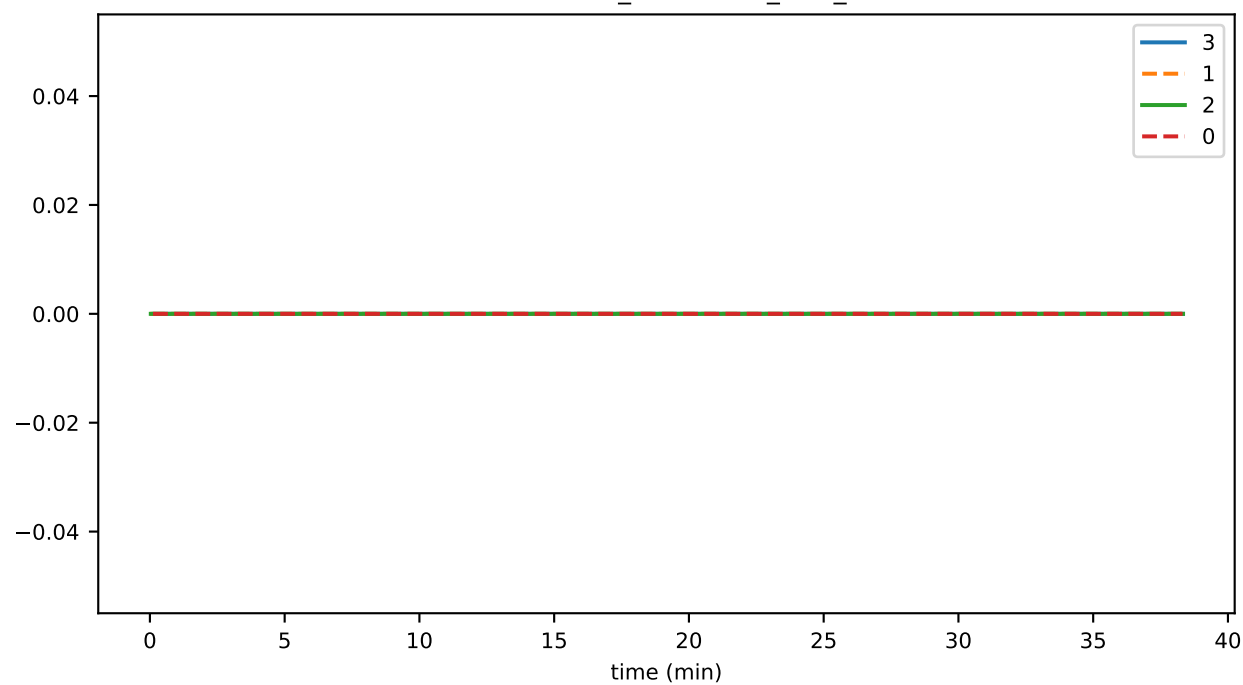
PlatformMonitor_unhandled_task_count
