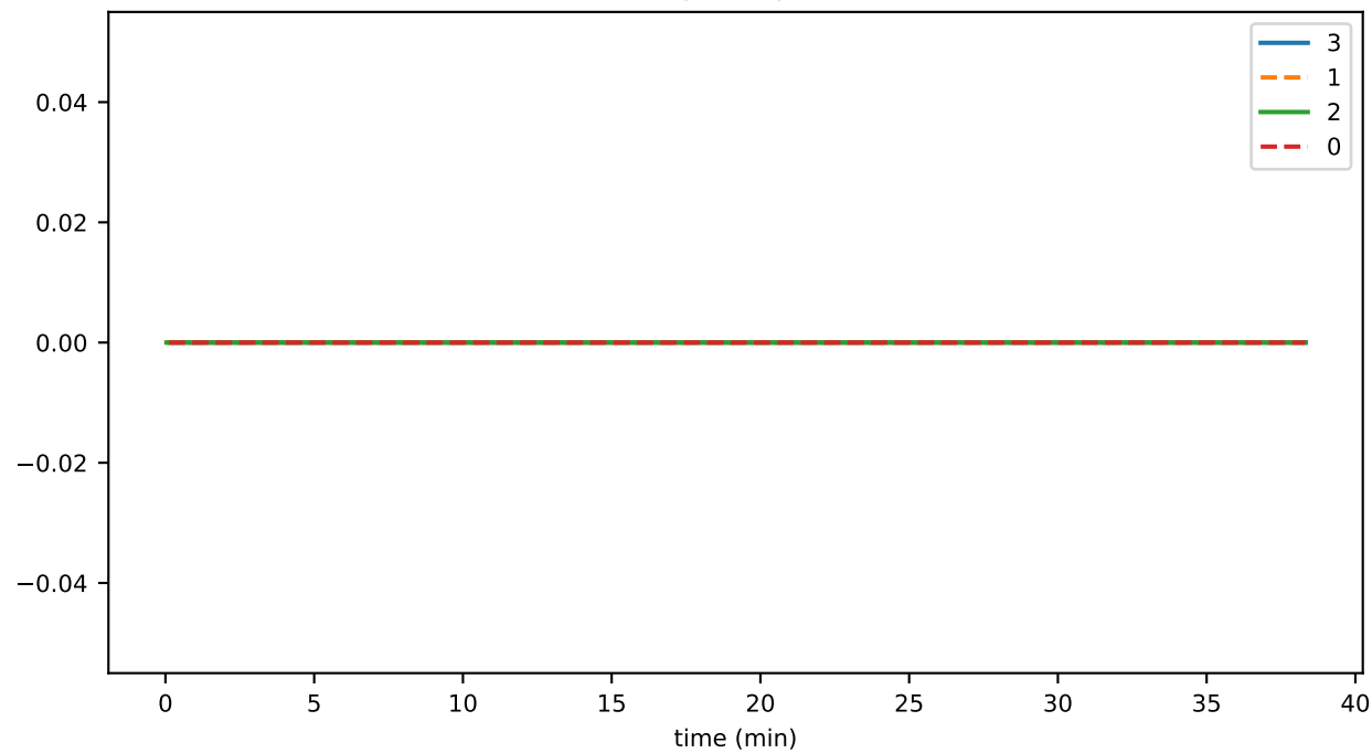
DigSpans_per_sec
