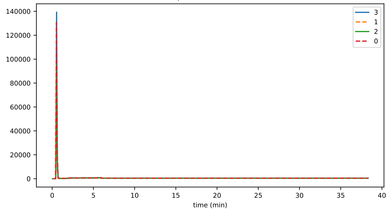
preHandleMicros
