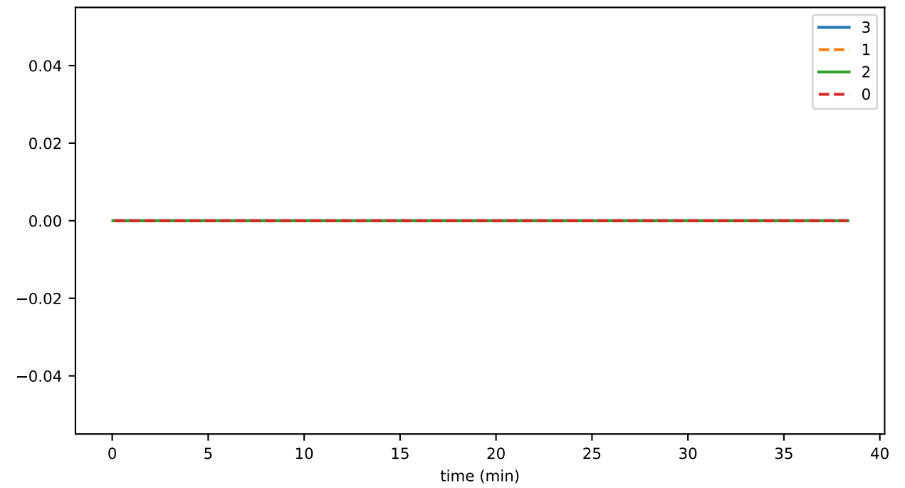
numReportFallenBehind
