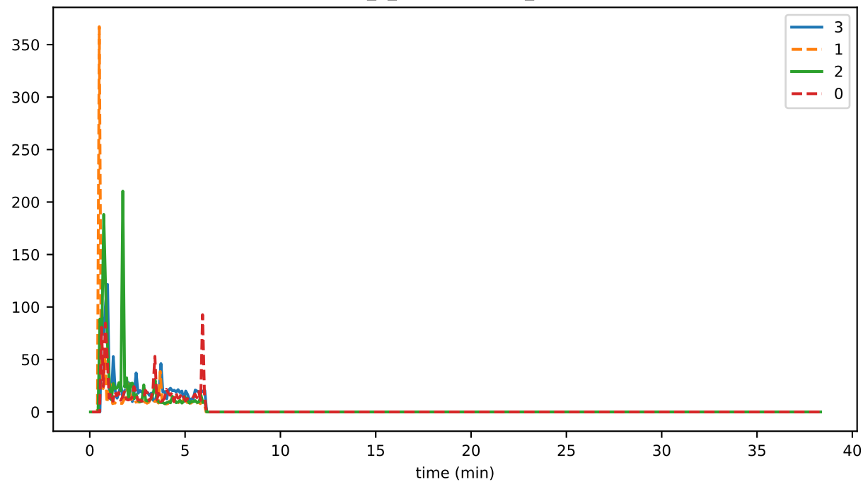
eventDelay_1_eventCreation_runtimeMAX
