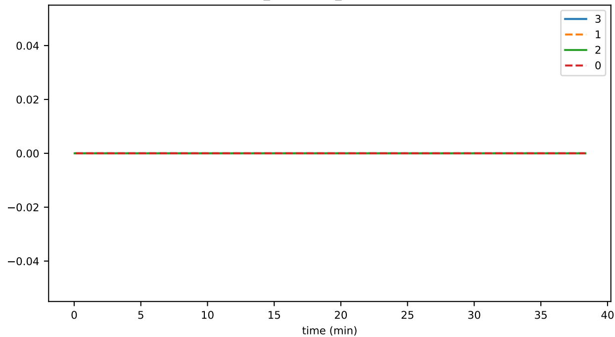
conn_connClose_configUpdate
