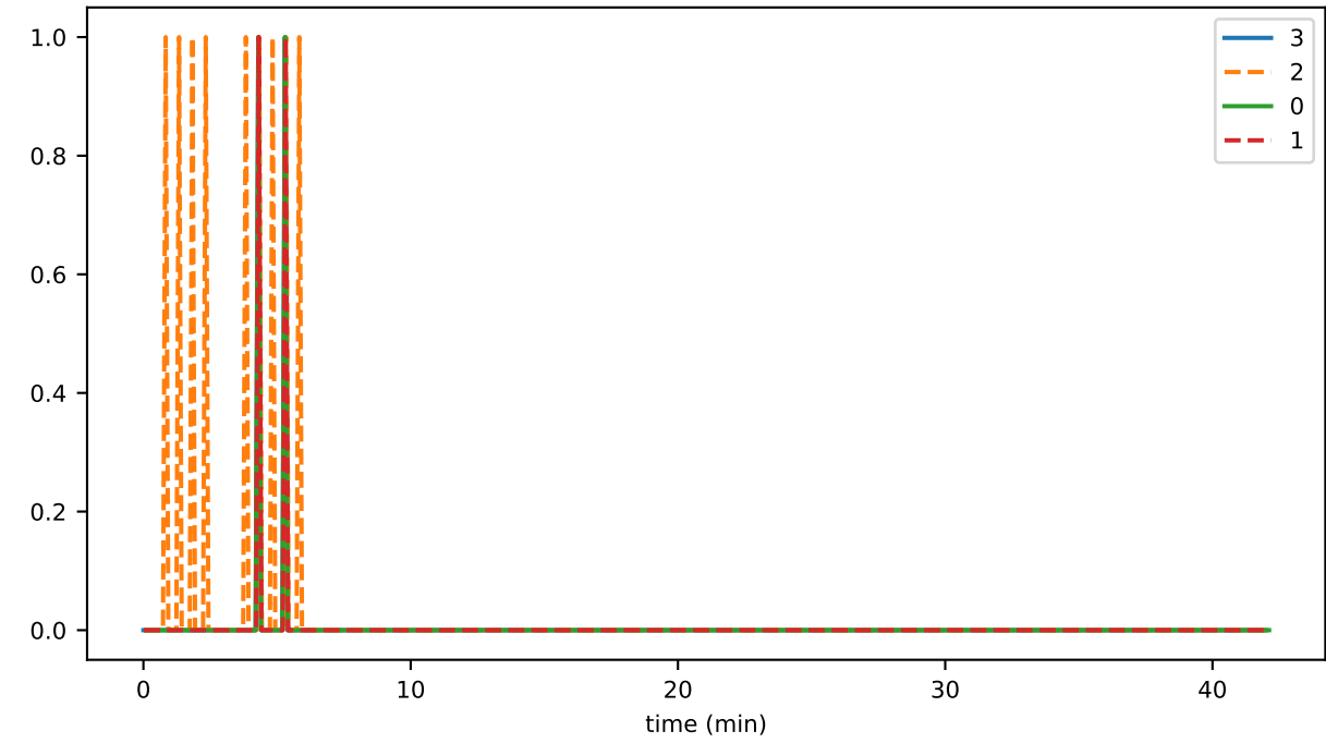
storageSlotsMaxNumber
