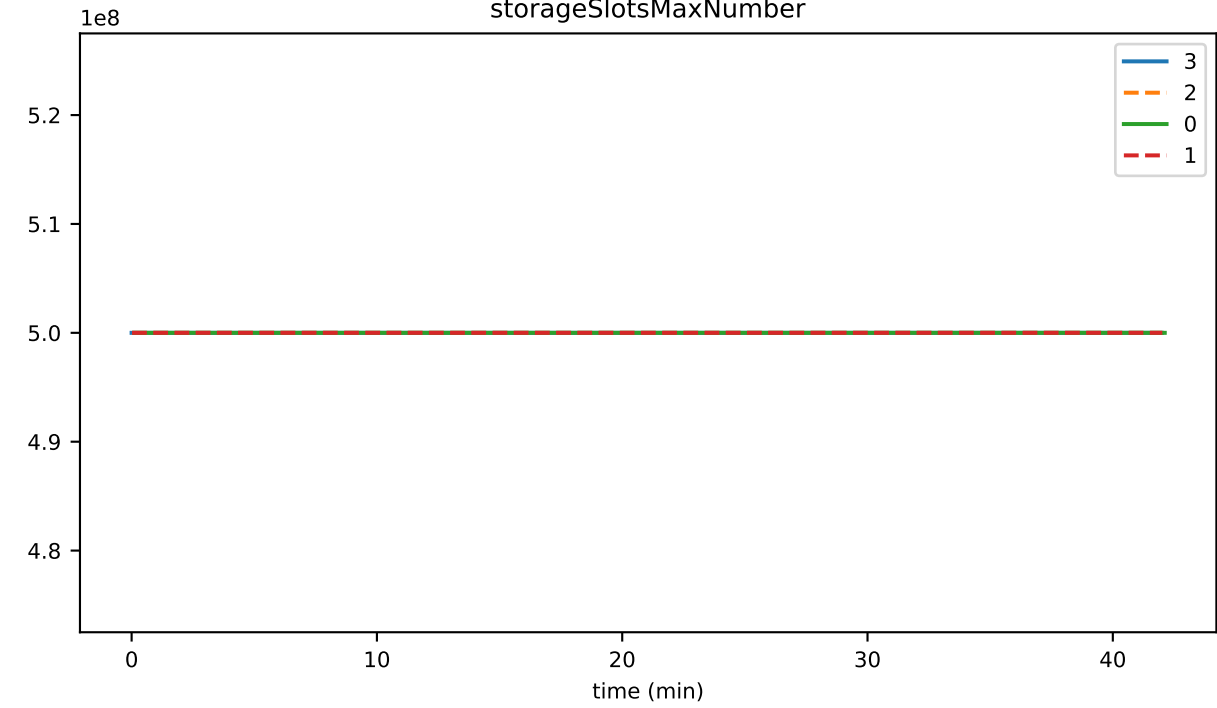
storageSlotsMaxNumber
