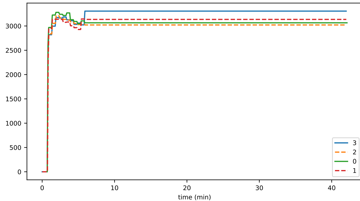
writeMerkleRootToDisk
