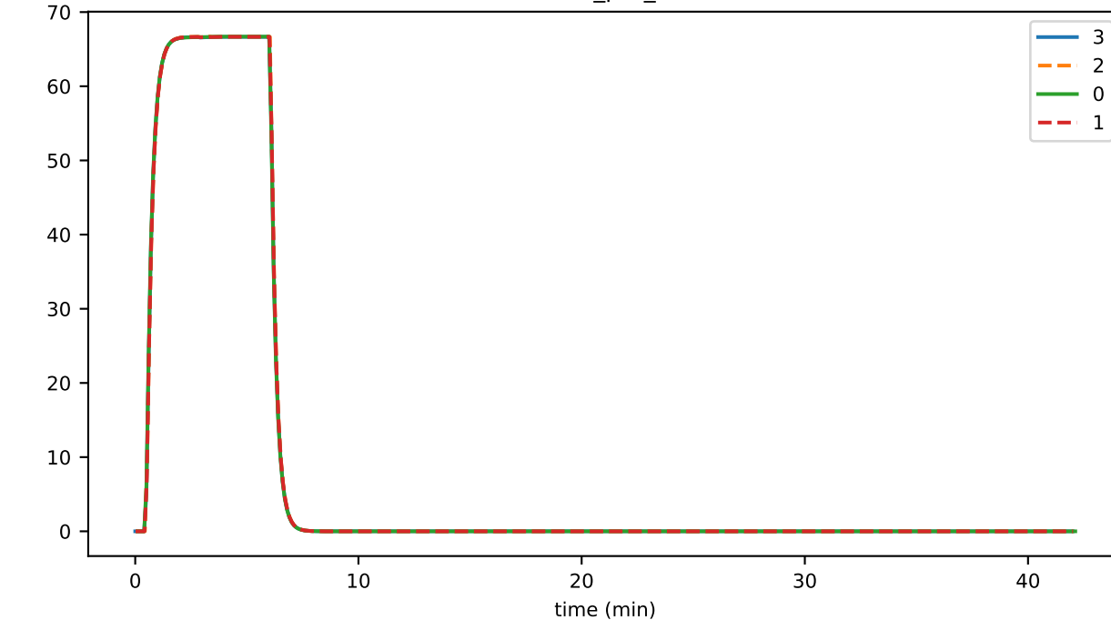
EventSignatureValidator_unhandled_task_count
