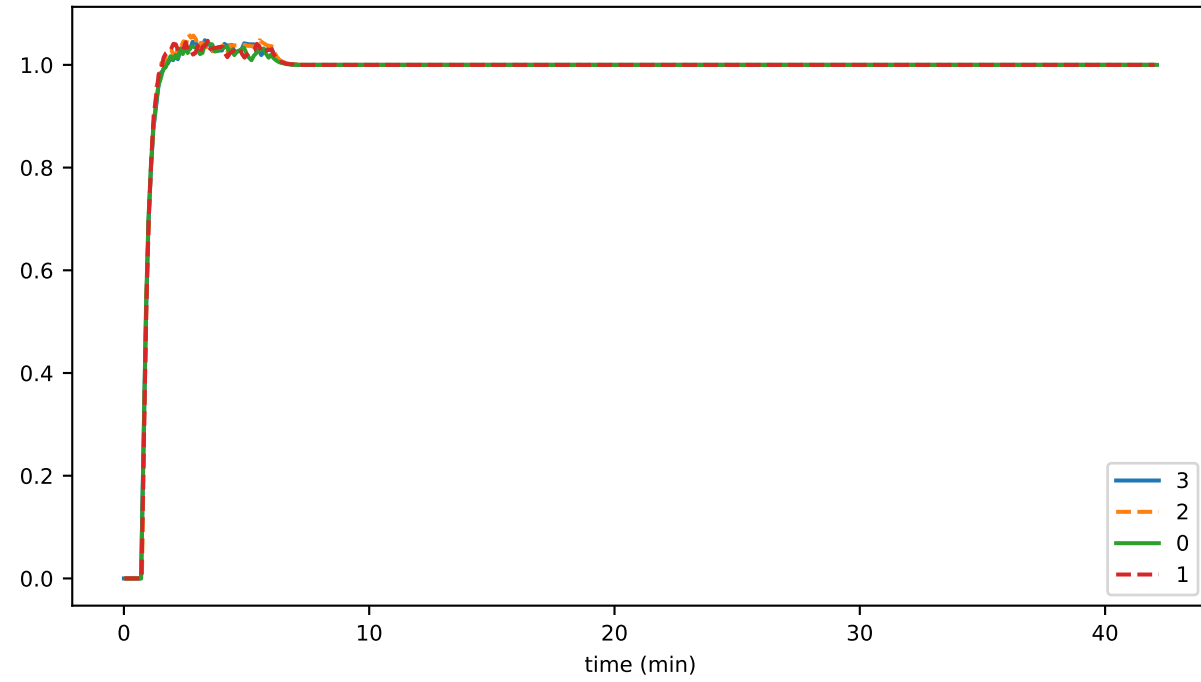
stateToDisk
