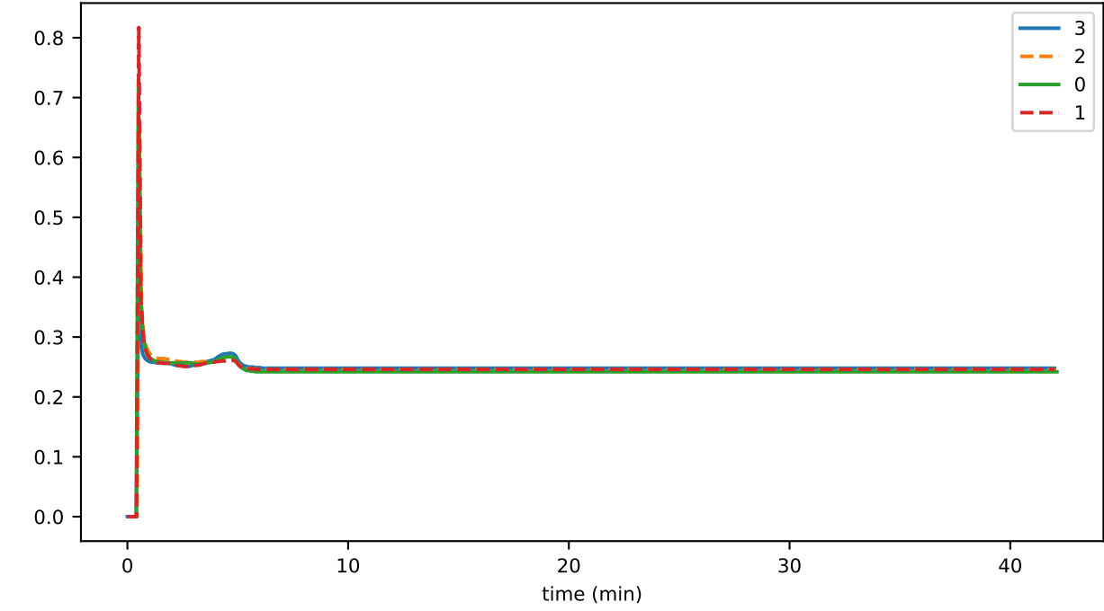
secC2RC
