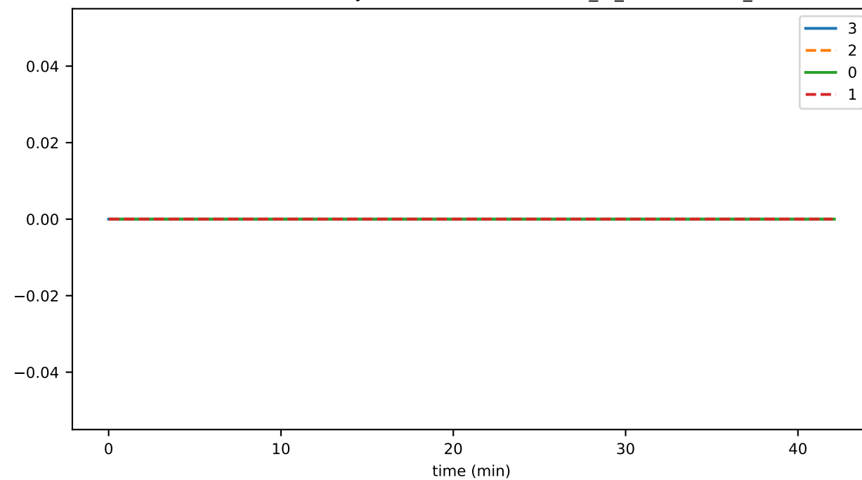
SmartContractService:SystemContractMethodCall_IS_AUTHORIZED_failed
