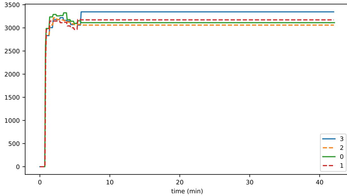
stateToDisk
