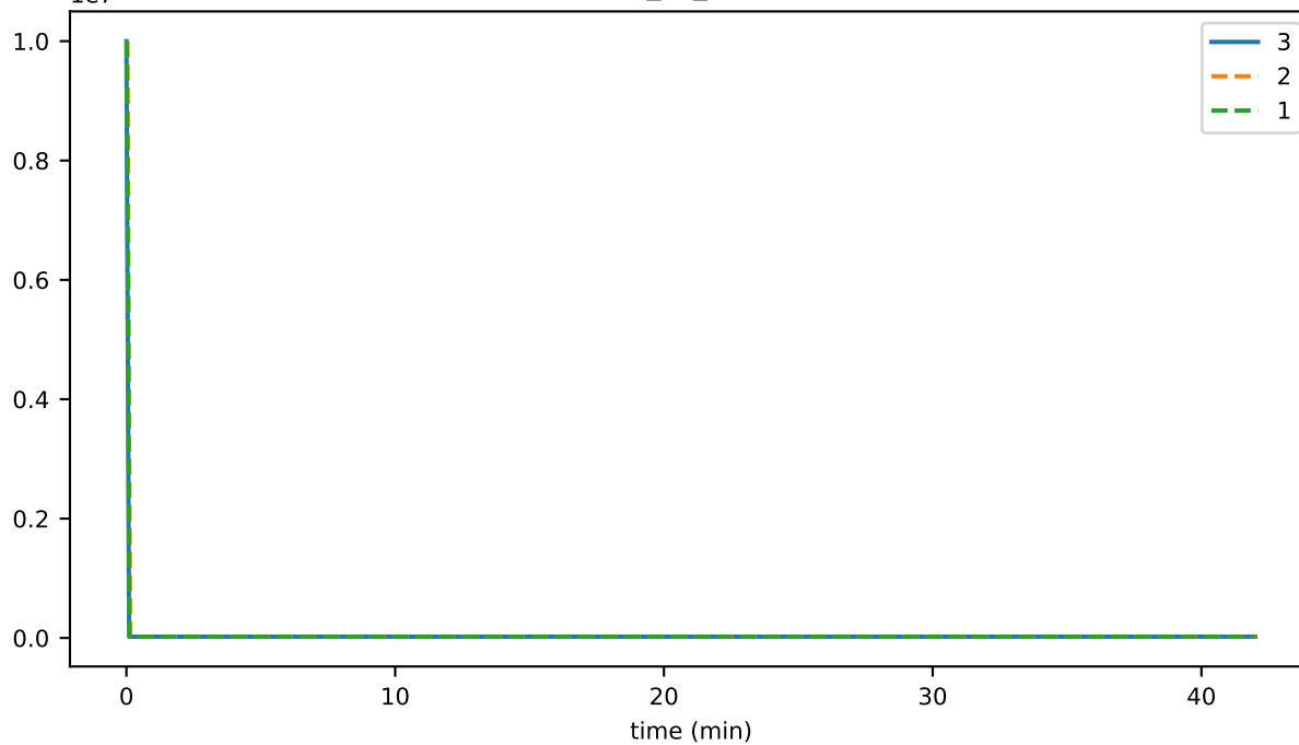
ping_us_00MIN
