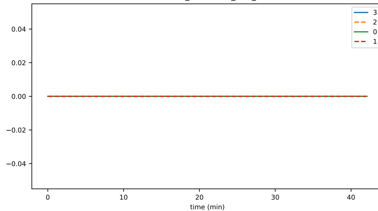
StateHasher_unhandled_task_count
