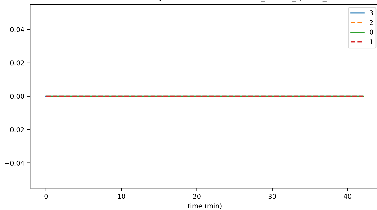
SmartContractService:SystemContractMethodCall_TOKEN_QUERY_total
