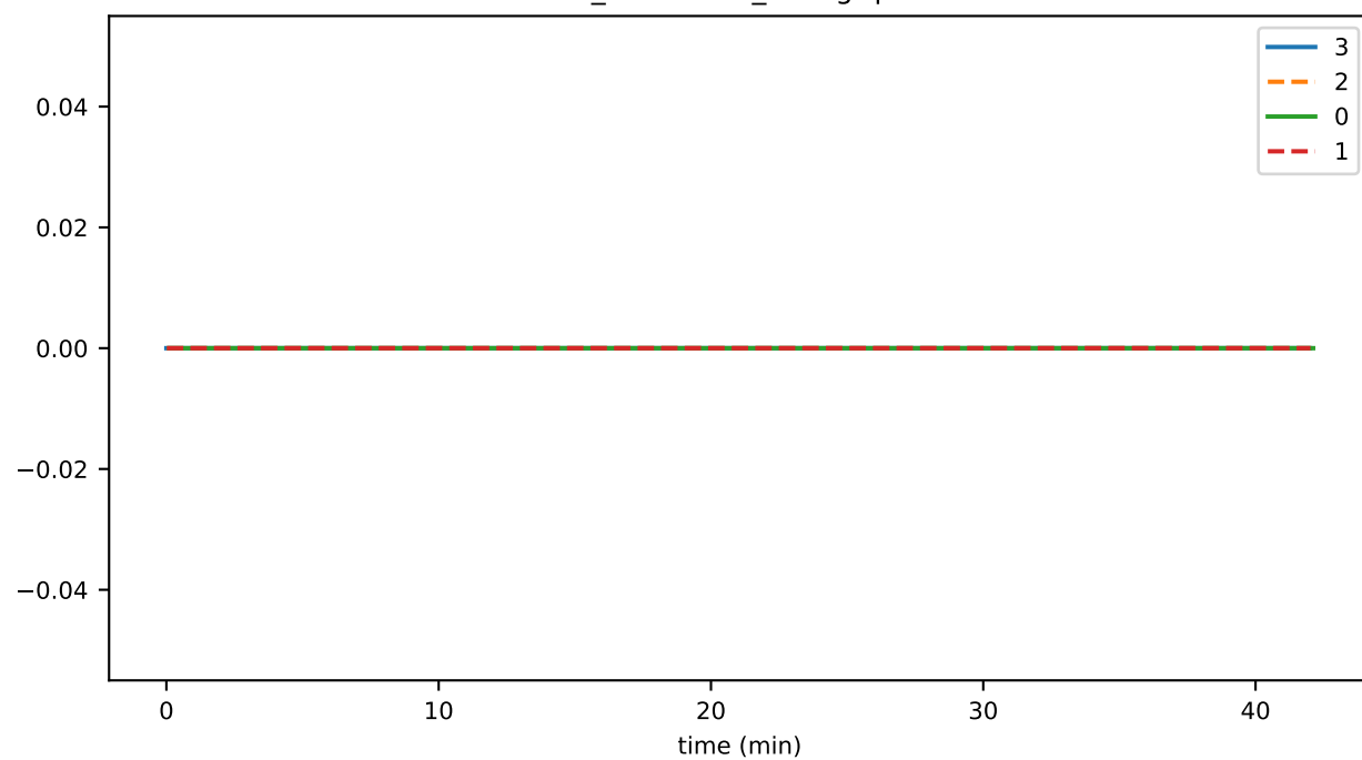
conn_connClose_configUpdate
