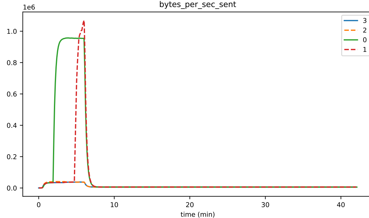
bytes_per_sec_sent_01
