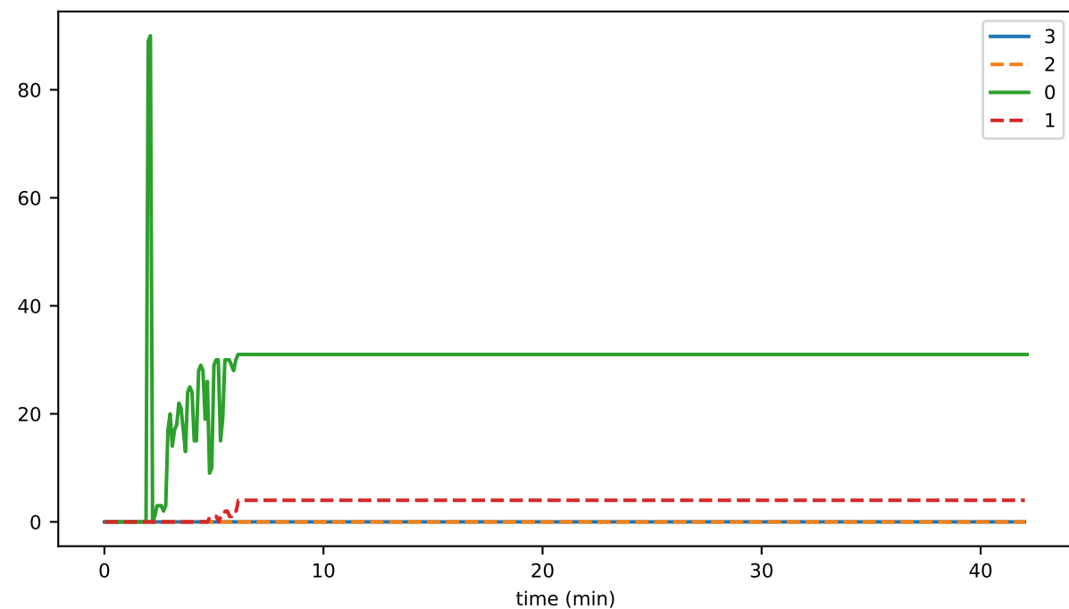
bytes_per_sec_sent_00
