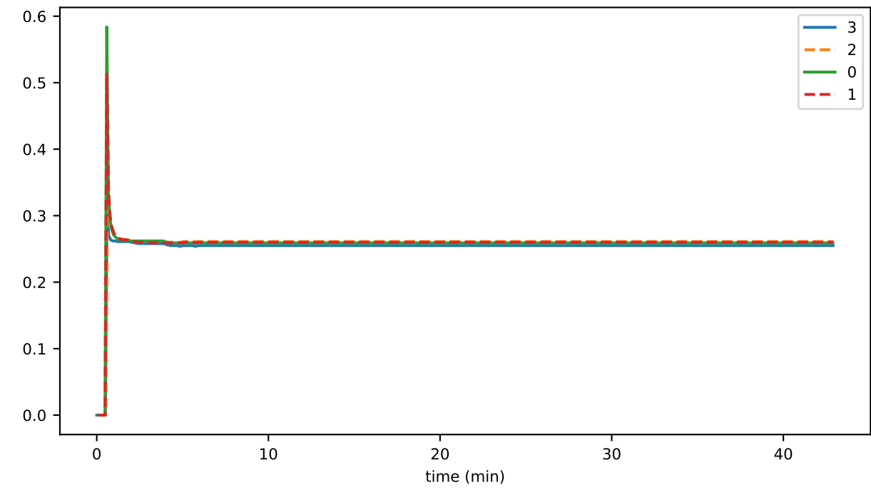
secC2RC
