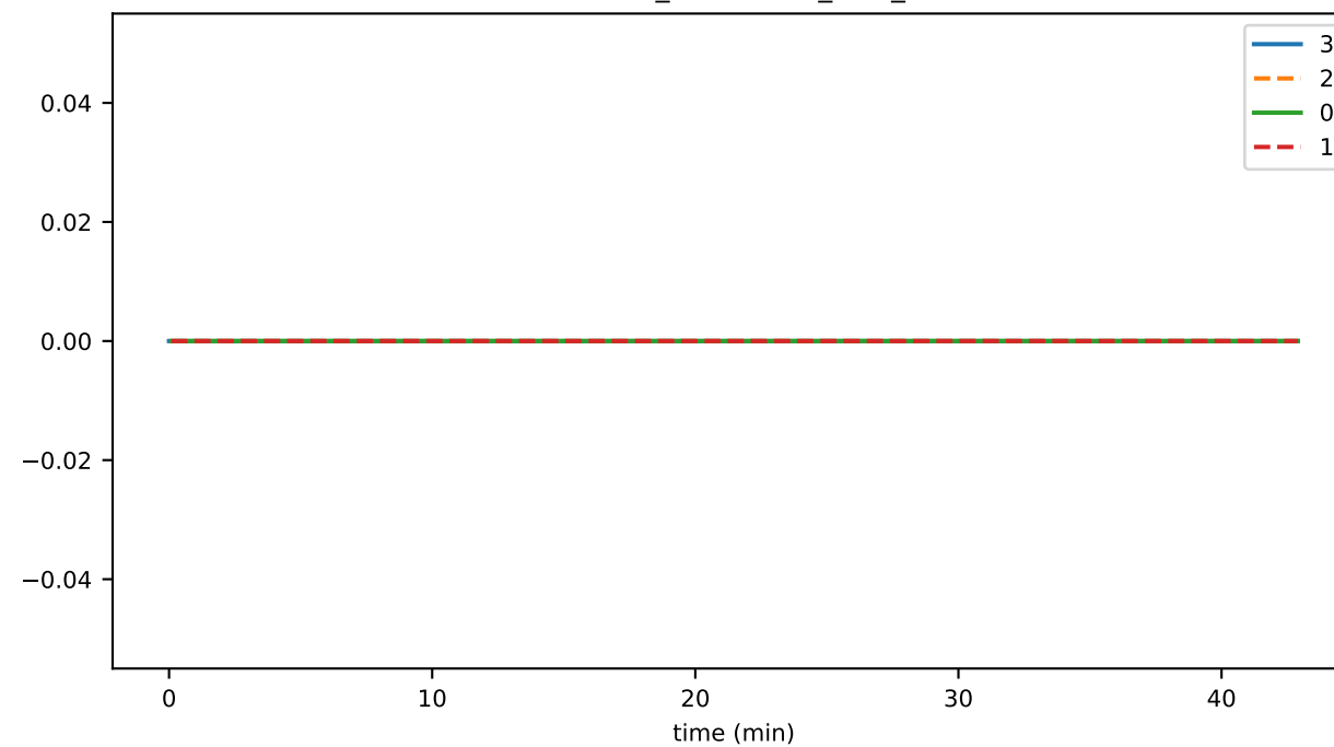
StateHasher_unhandled_task_count
