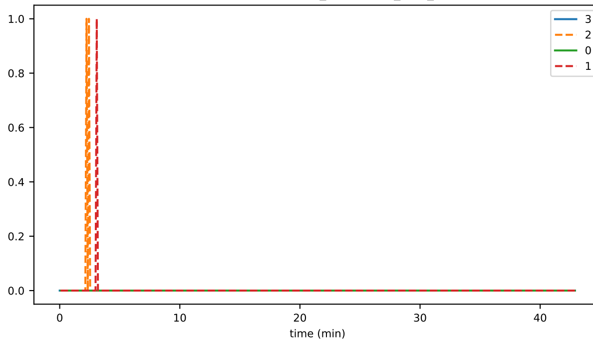
EventSignatureValidator_unhandled_task_count
