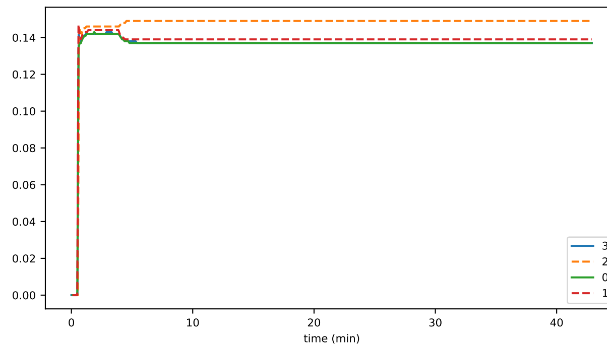
secR2F
