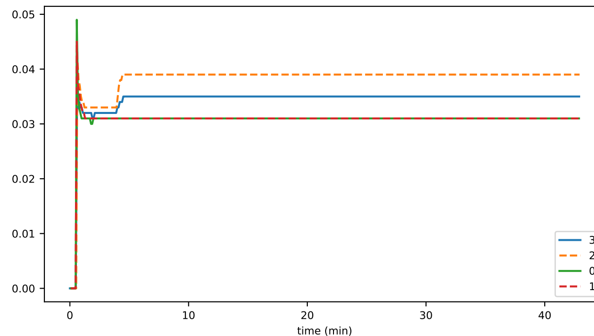
secR2F
