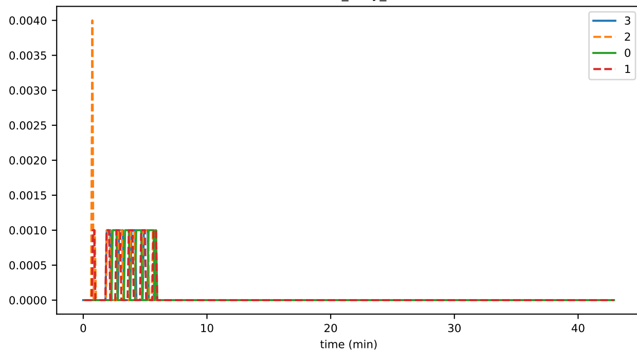
StateHasher_busy_fraction
