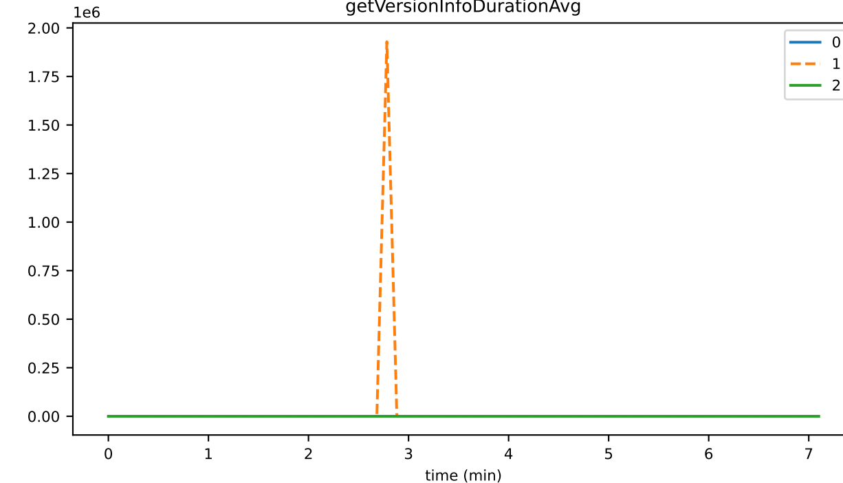
getVersionInfoDurationAvg
