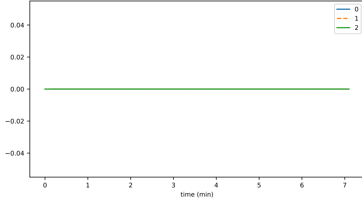
cryptoGetInfoThrottledTxns
