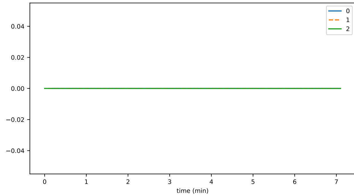
pityParent1
