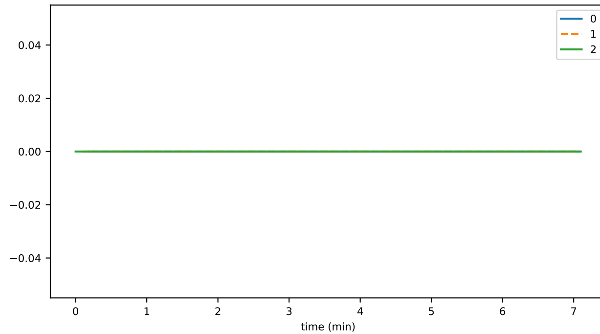
pityParent2
