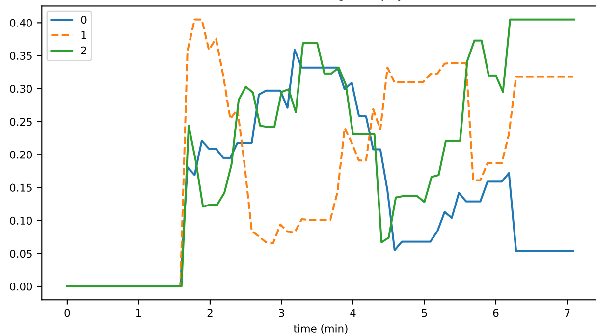
indicatorsWaitingForExpiry
