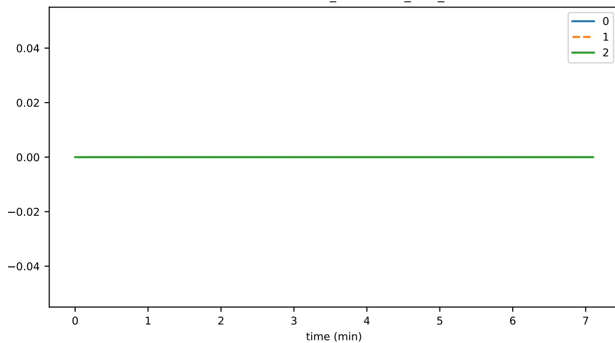
TransactionPrehandler_unhandled_task_count
