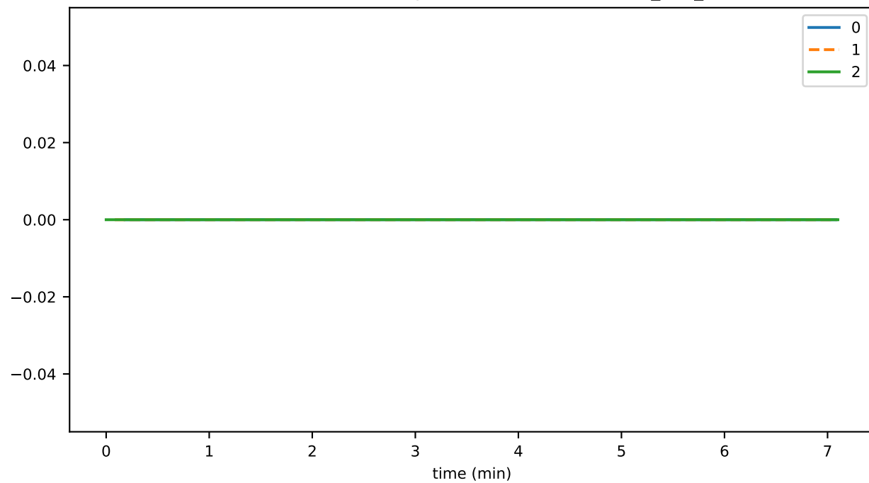
SmartContractService:SystemContractMethodCall_MINT_BURN_total
