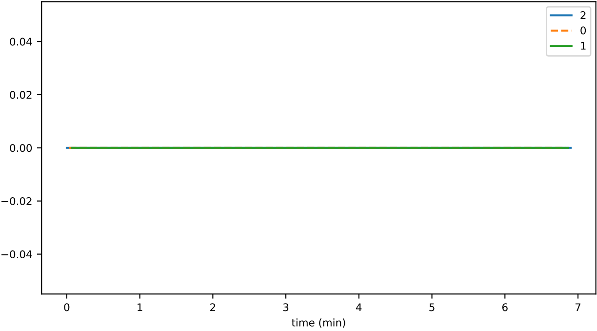
SmartContractService:SystemContractMethodCall_FREEZE_UNFREEZE_total
