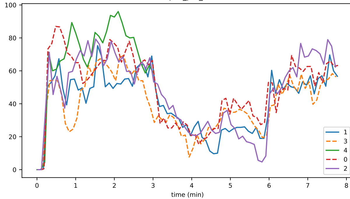
dupEv_per_sec
