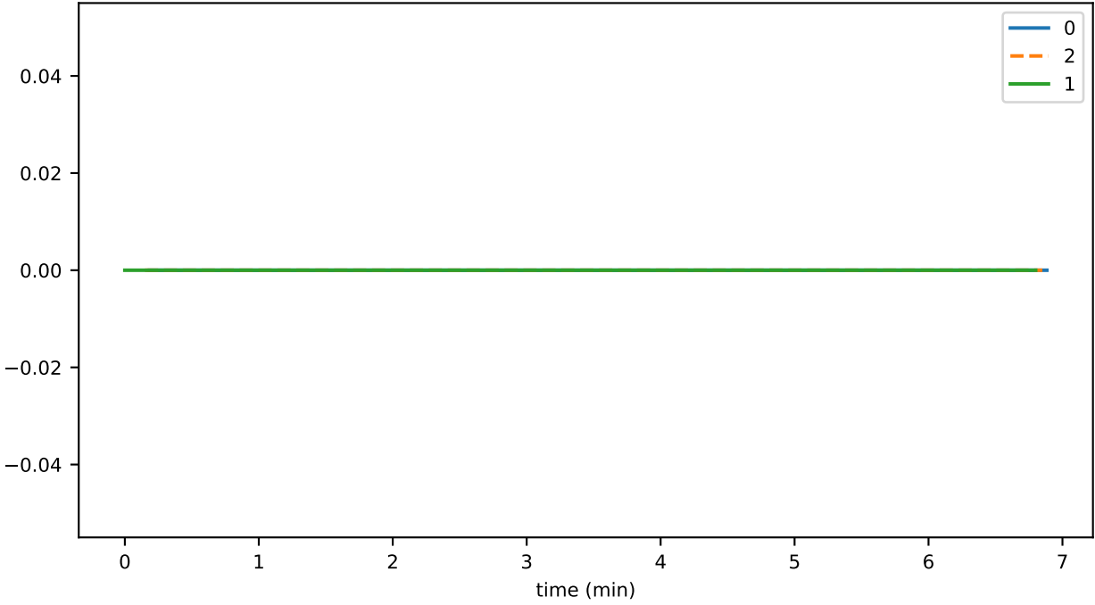
SmartContractService:SystemContractMethodCall_HAS_total
