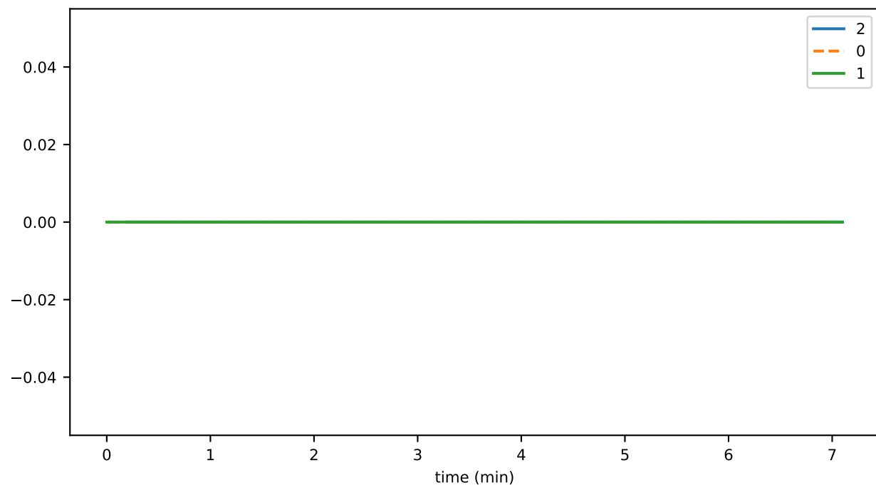
tokenCreateThrottledTxns
