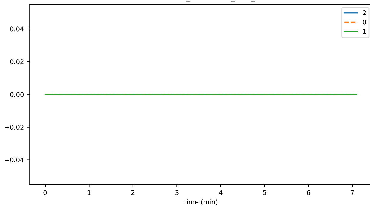
PlatformMonitor_unhandled_task_count
