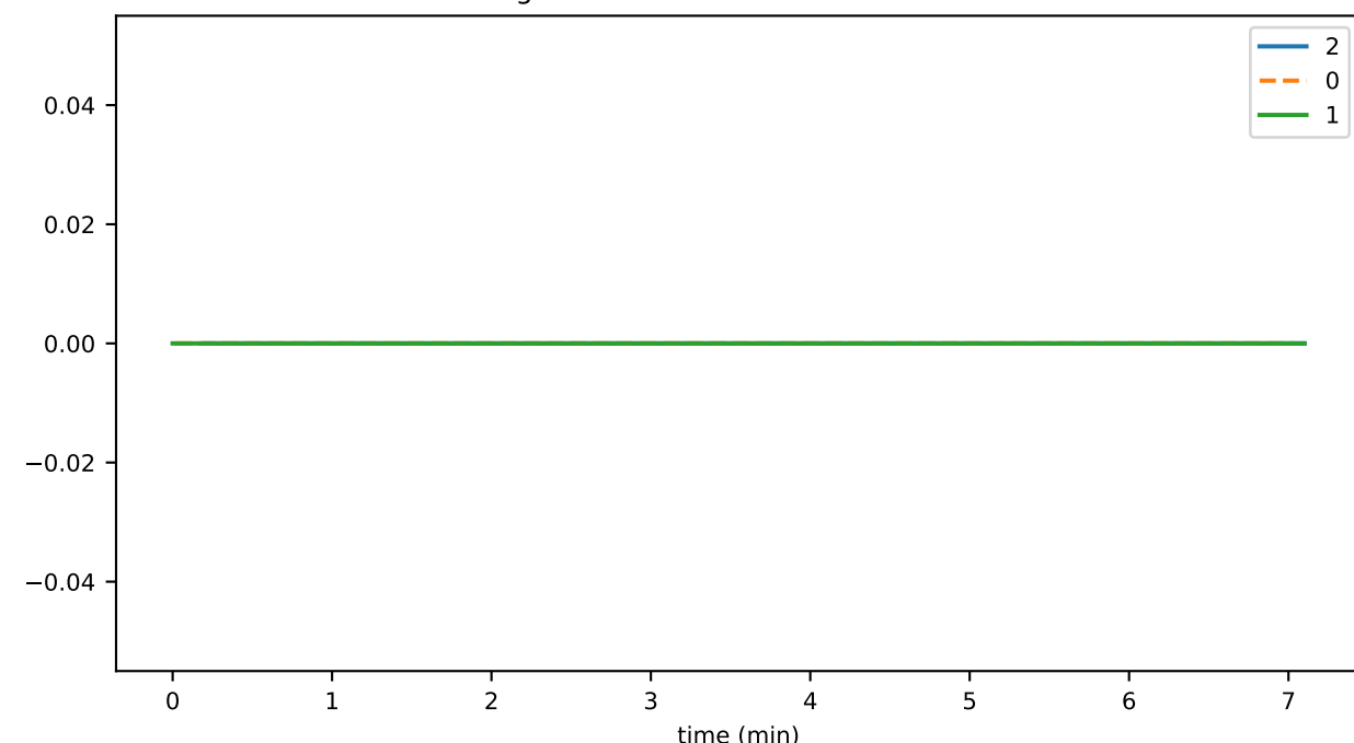
registeredNodeDeleteThrottledTxns
