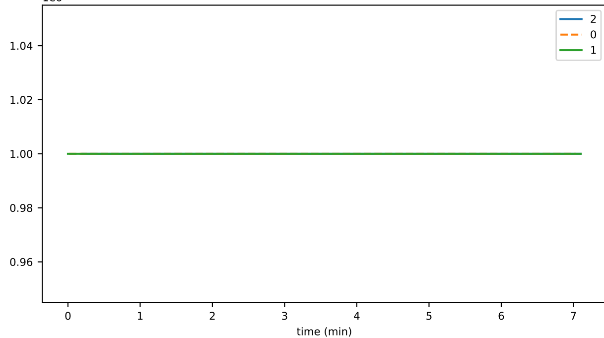
tokensMaxNumber
