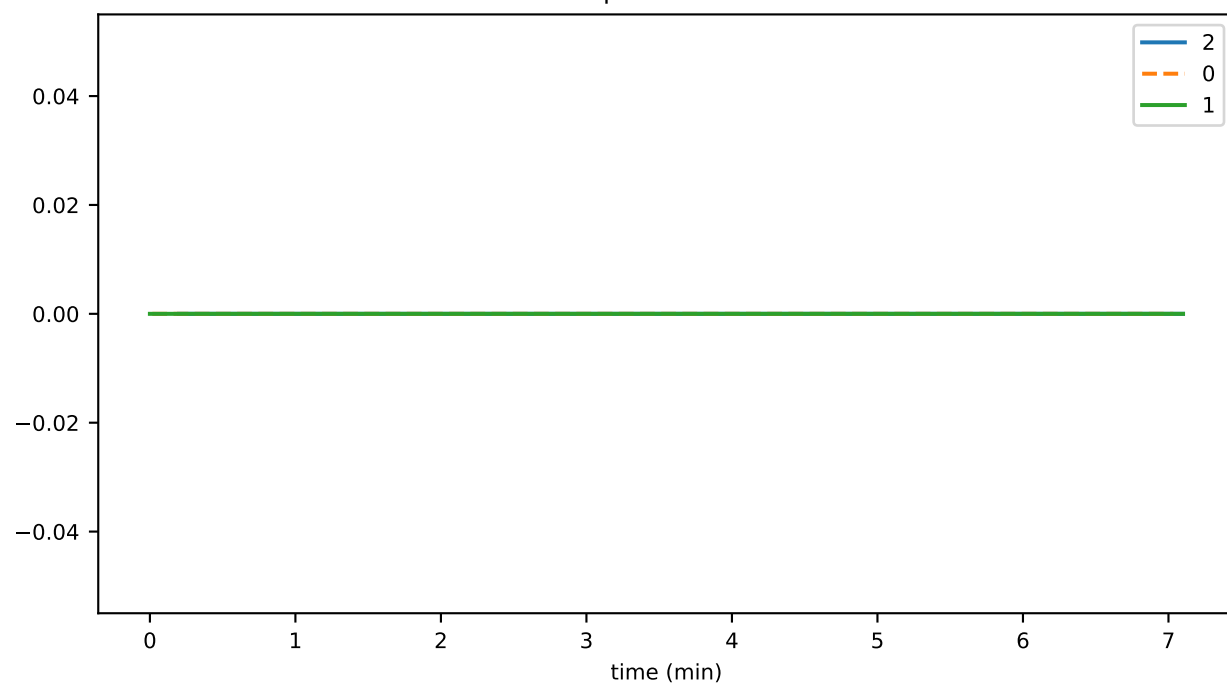
contractUpdateThrottledTxns
