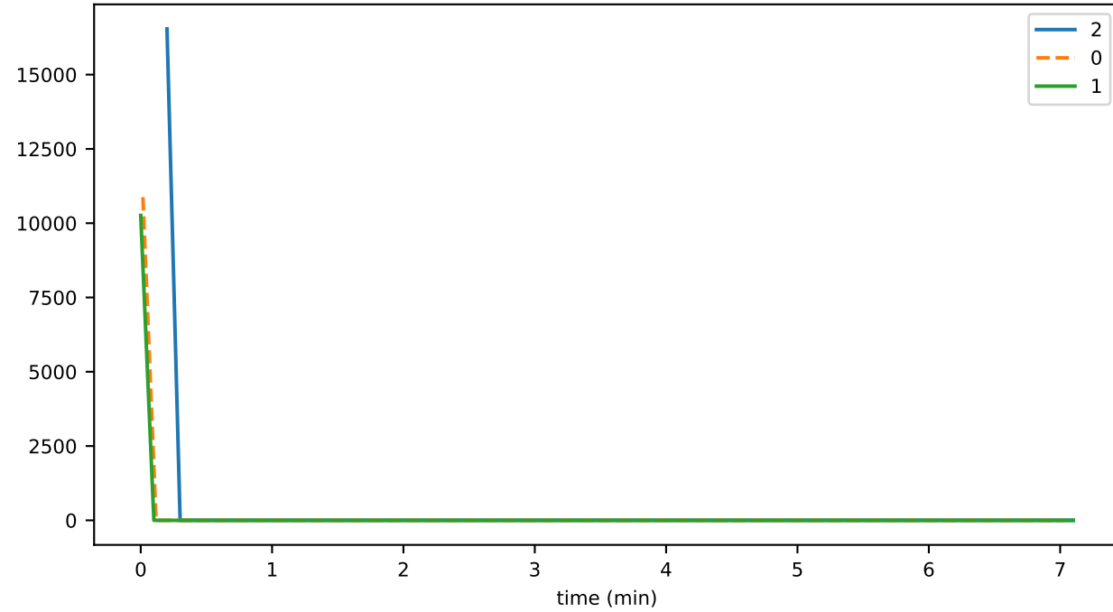
eventDelay_2_validation_gossipMAX
