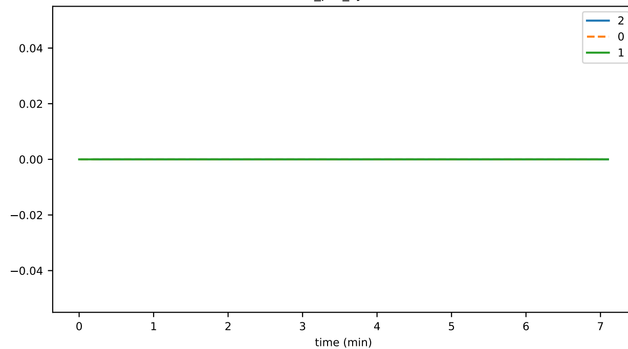
ev_per_syncR
