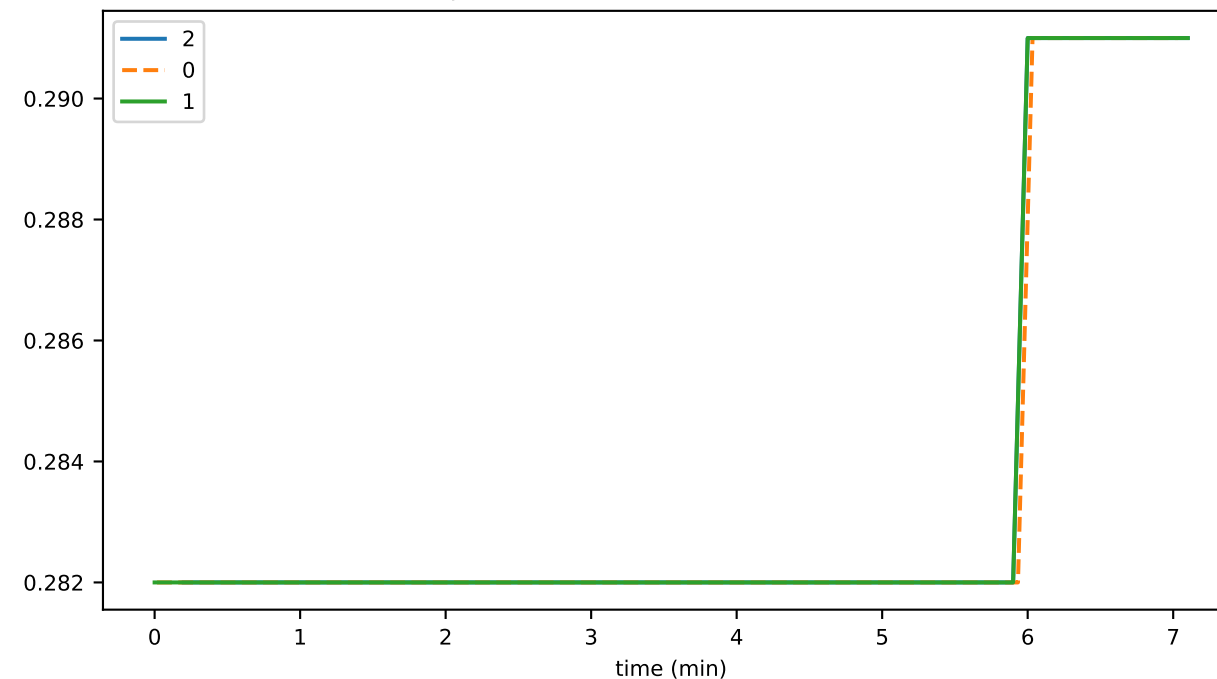
preHandleMicros
