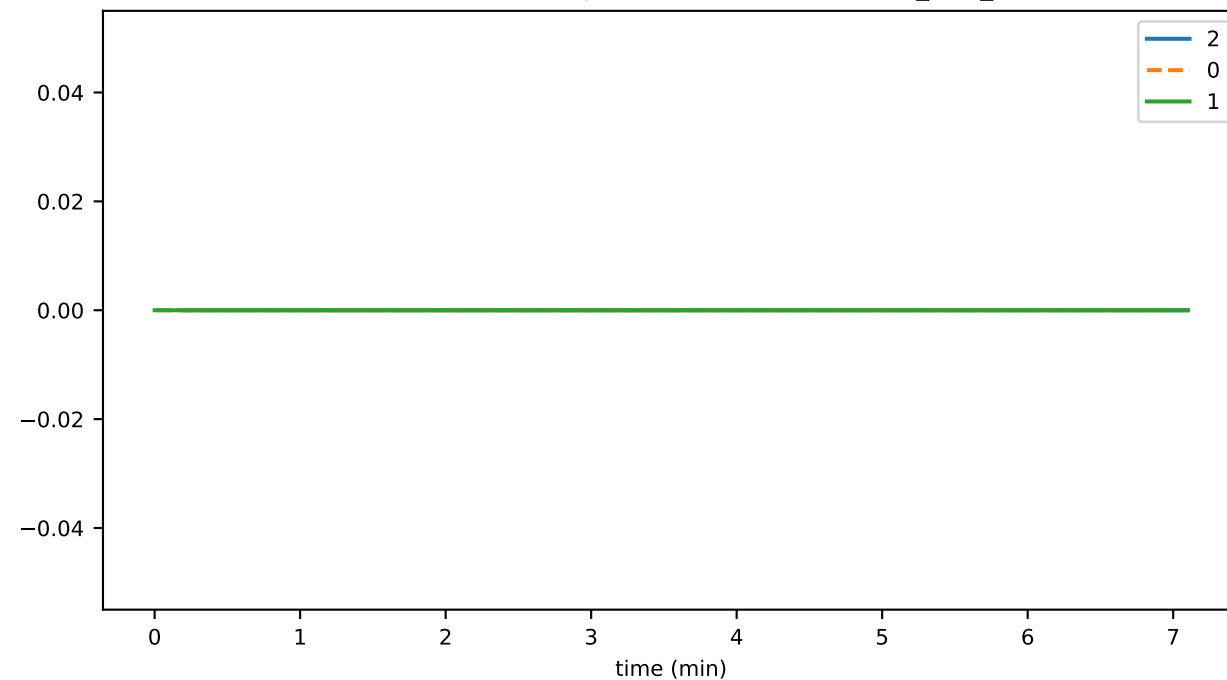
SmartContractService:SystemContractMethodCall_IS_AUTHORIZED_failed
