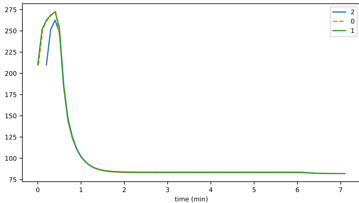
eventsInMem
