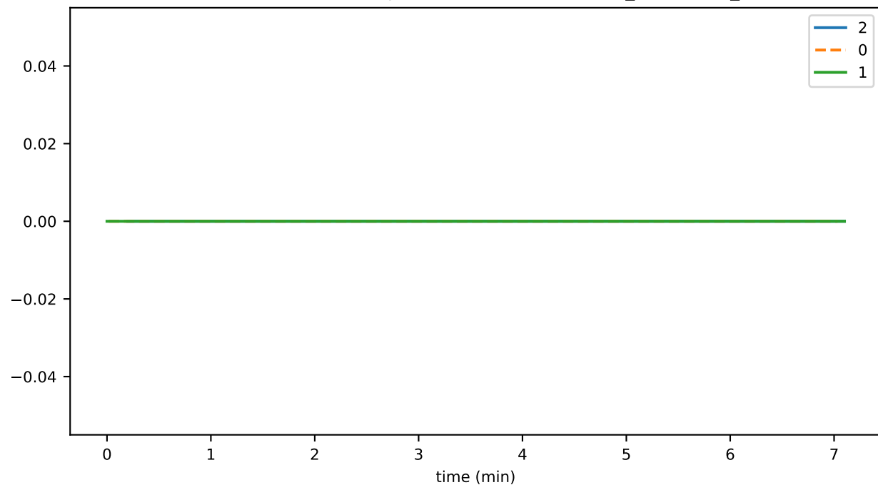
SmartContractService:SystemContractMethodCall_UPDATE_total
