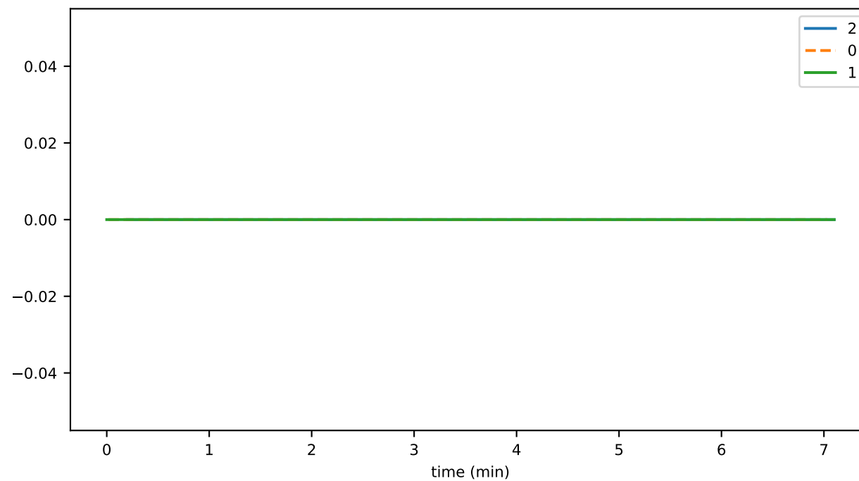
contractsUsed
