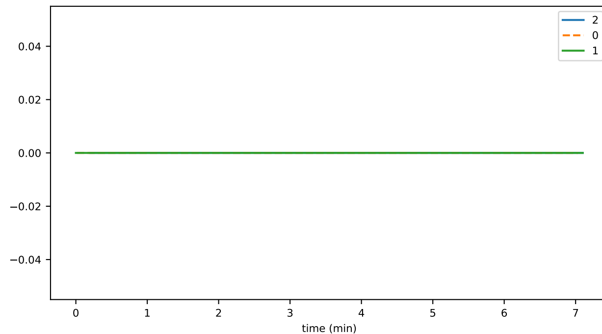
nftsMaxNumber
