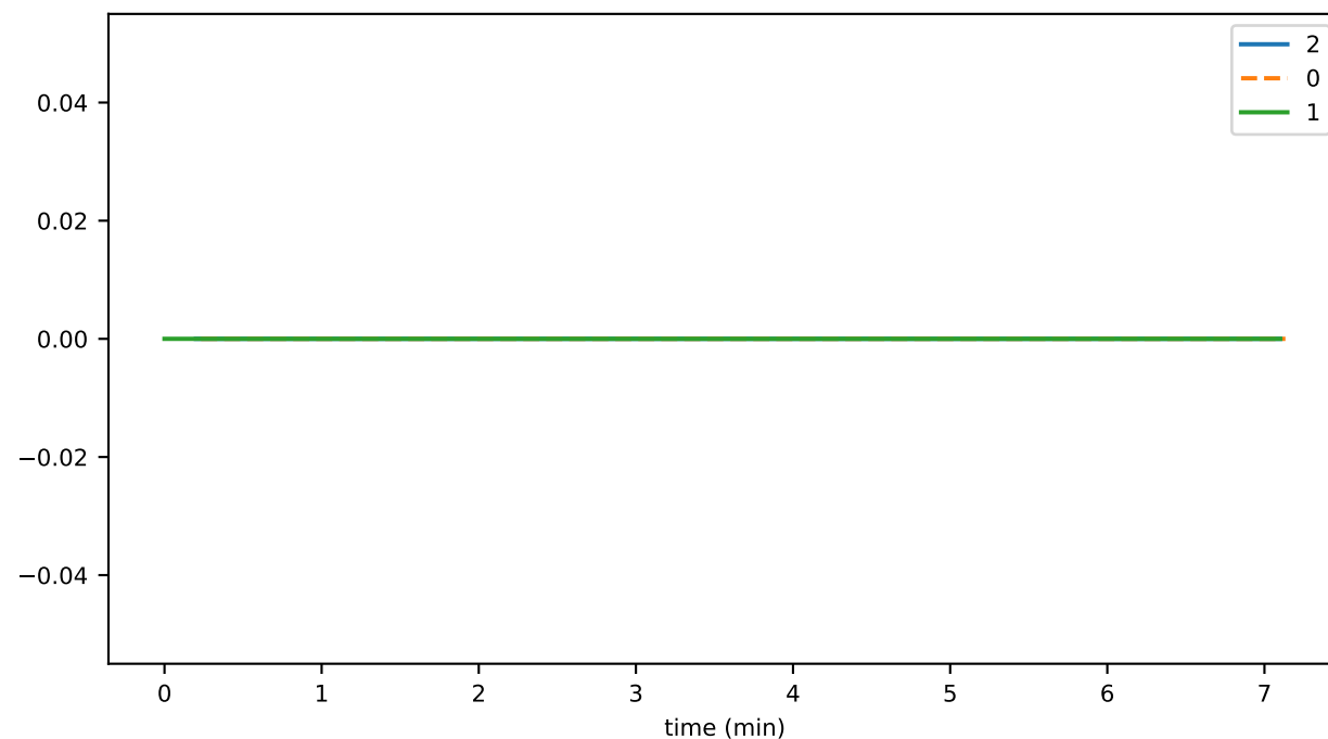
tokenGetNftInfoDurationAvg
