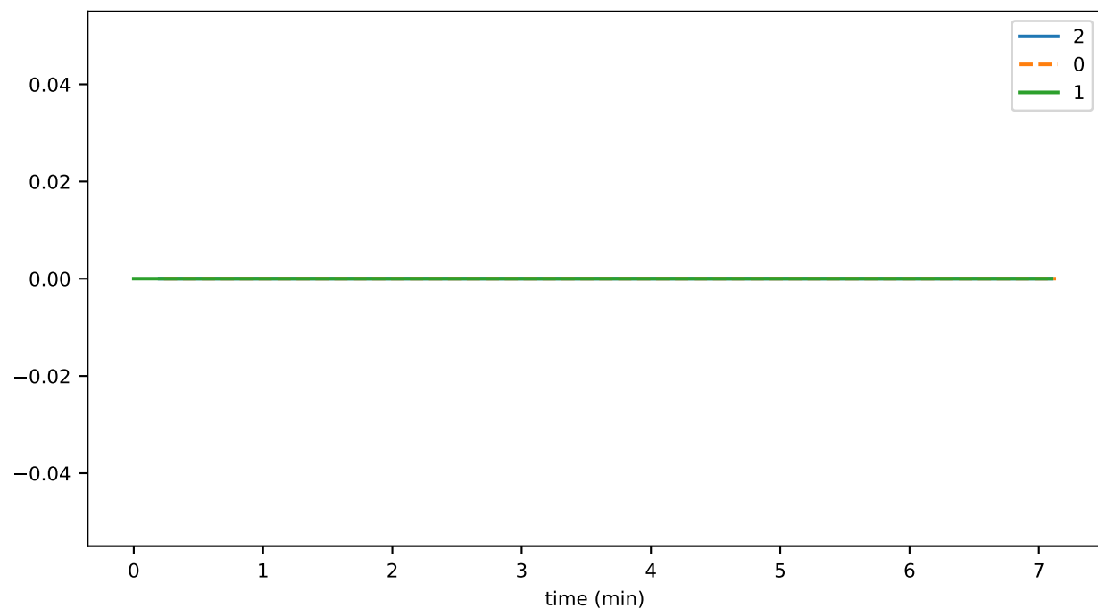
pcesAvgEventSize
