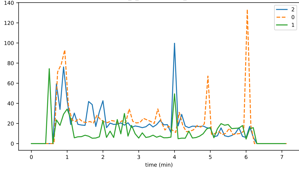
eventDelay_1_eventCreation_runtimeMAX
