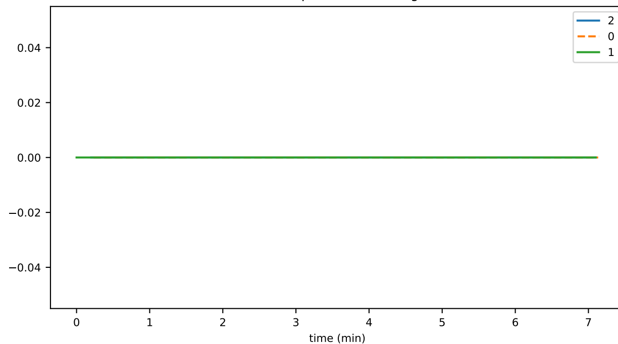
tokenUpdateNftsDurationAvg
