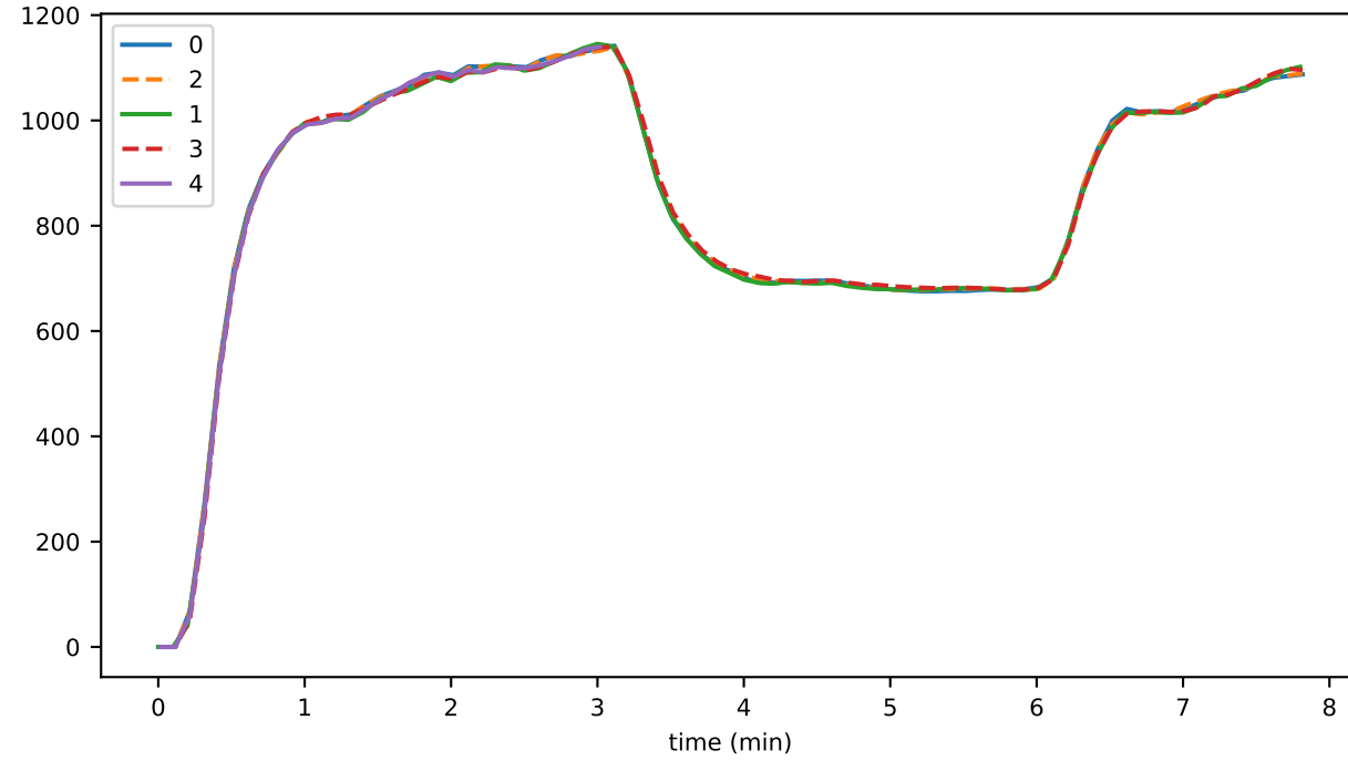
eventsInMem
