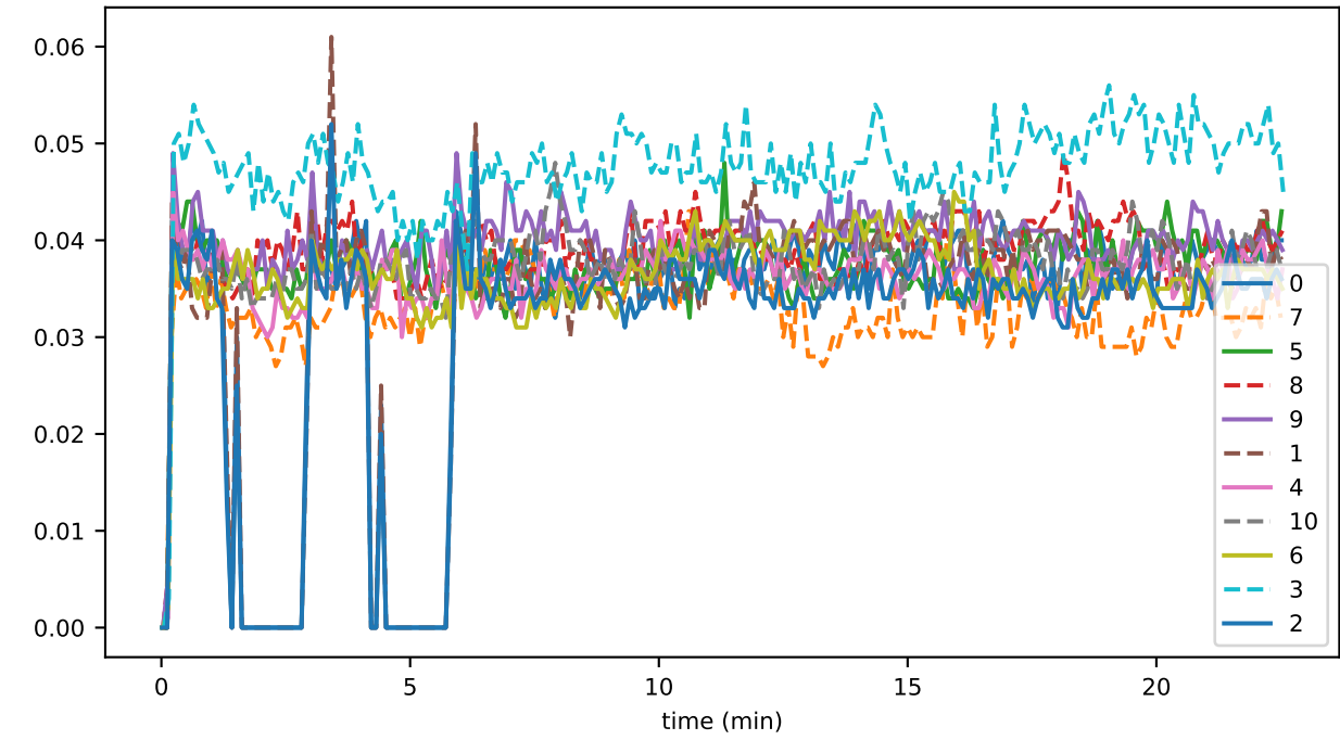
InternalEventValidator_unhandled_task_count
