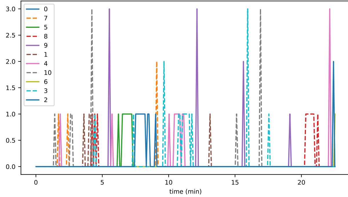
InlinePcesWriter_unhandled_task_count
