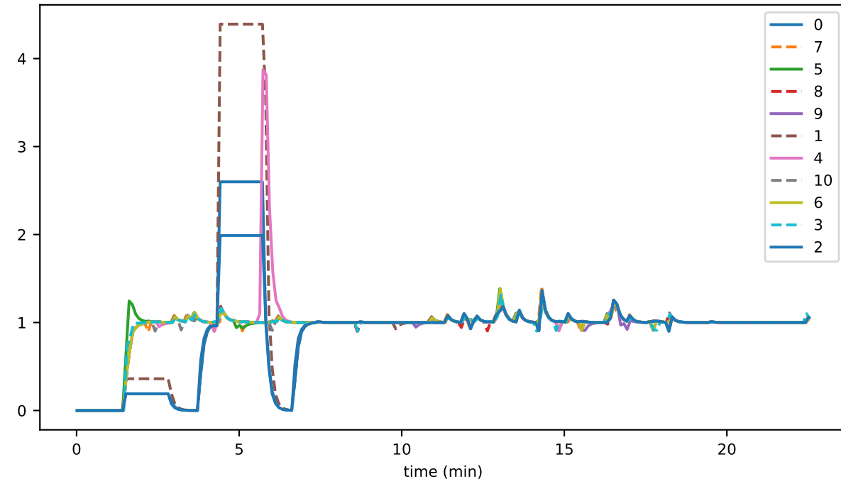
InlinePcesWriter_unhandled_task_count
