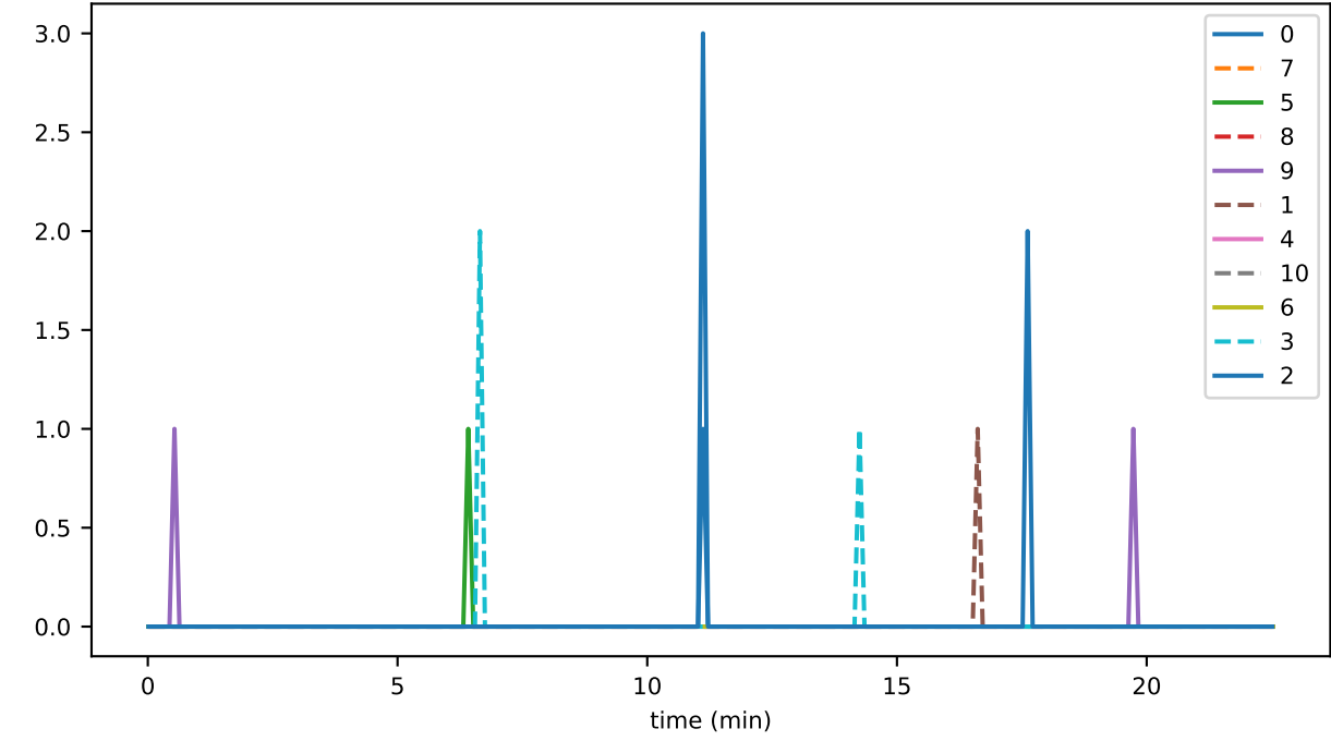
InternalEventValidator_unhandled_task_count
