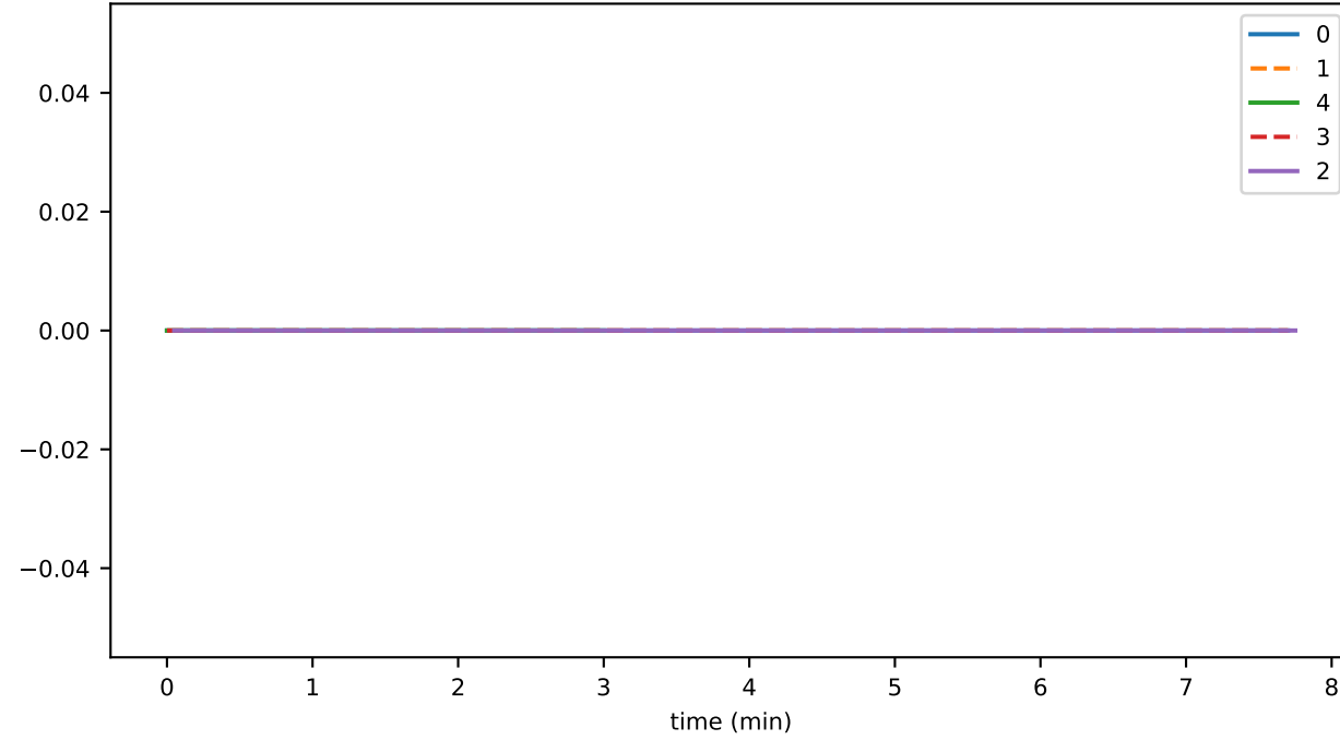
InternalEventValidator_unhandled_task_count
