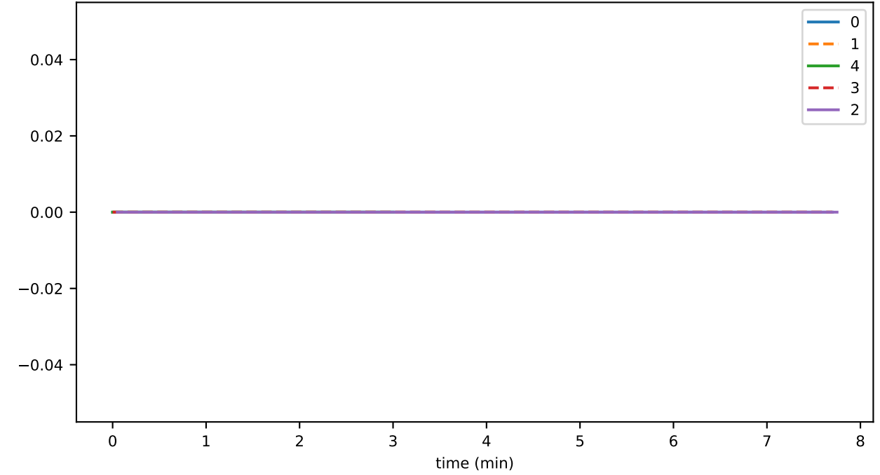
issCount
