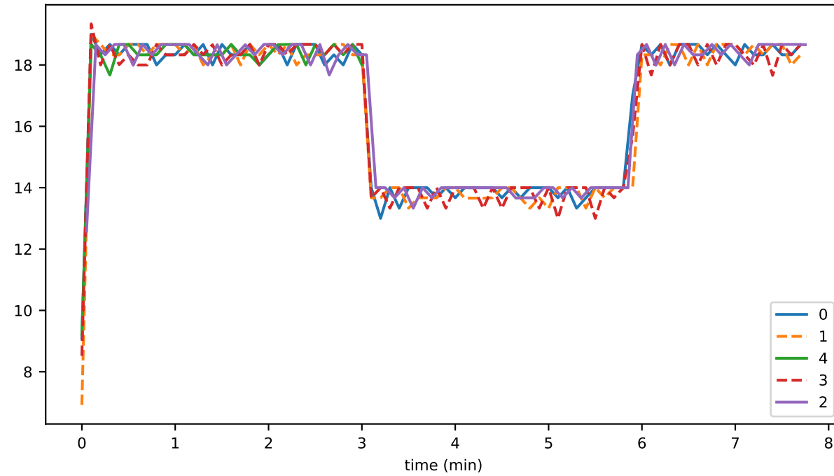
timeFracDot
