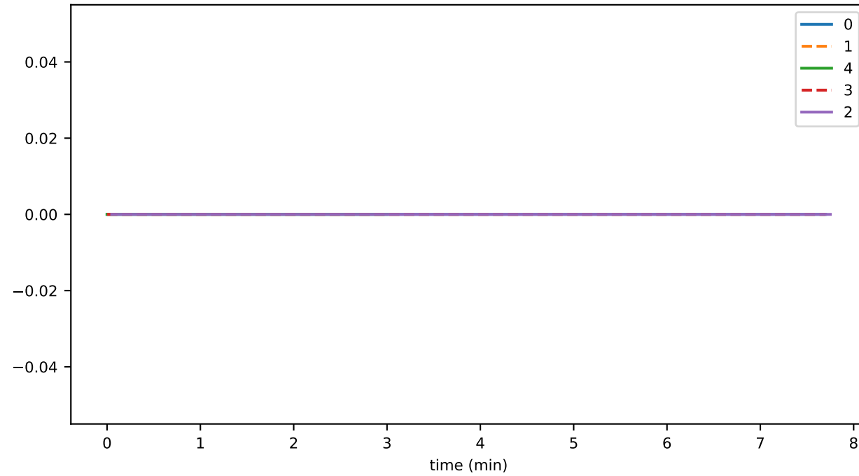
eventsInMem
