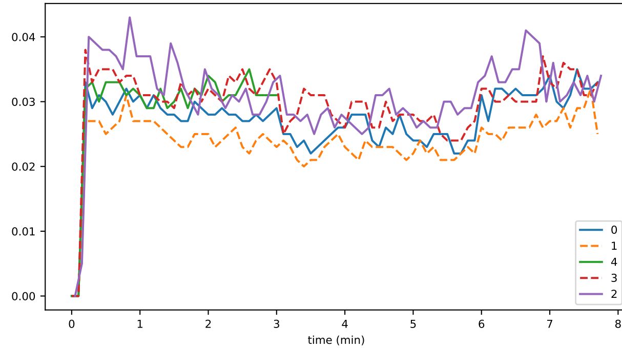
InternalEventValidator_unhandled_task_count
