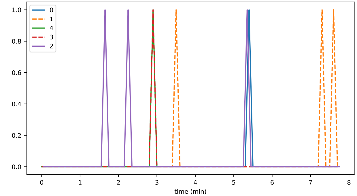
issCount
