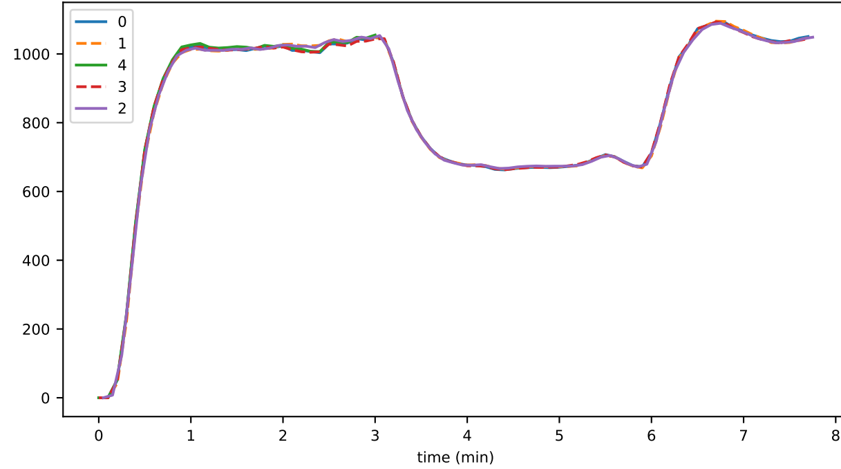
eventsInMem
