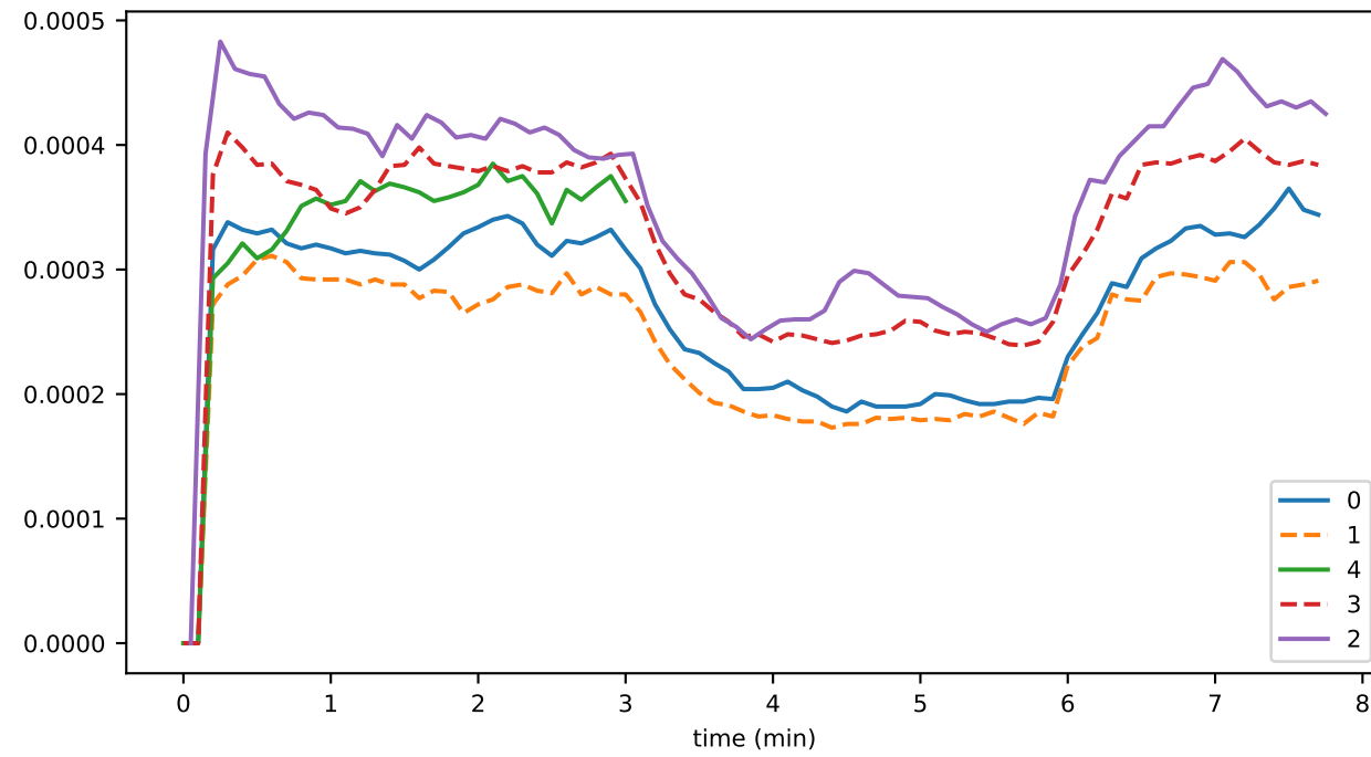
timeFracDot
