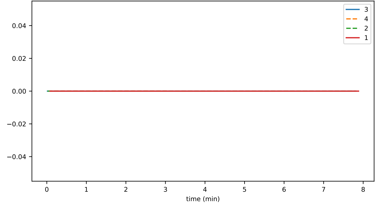
rpc_output_queue_size_00
