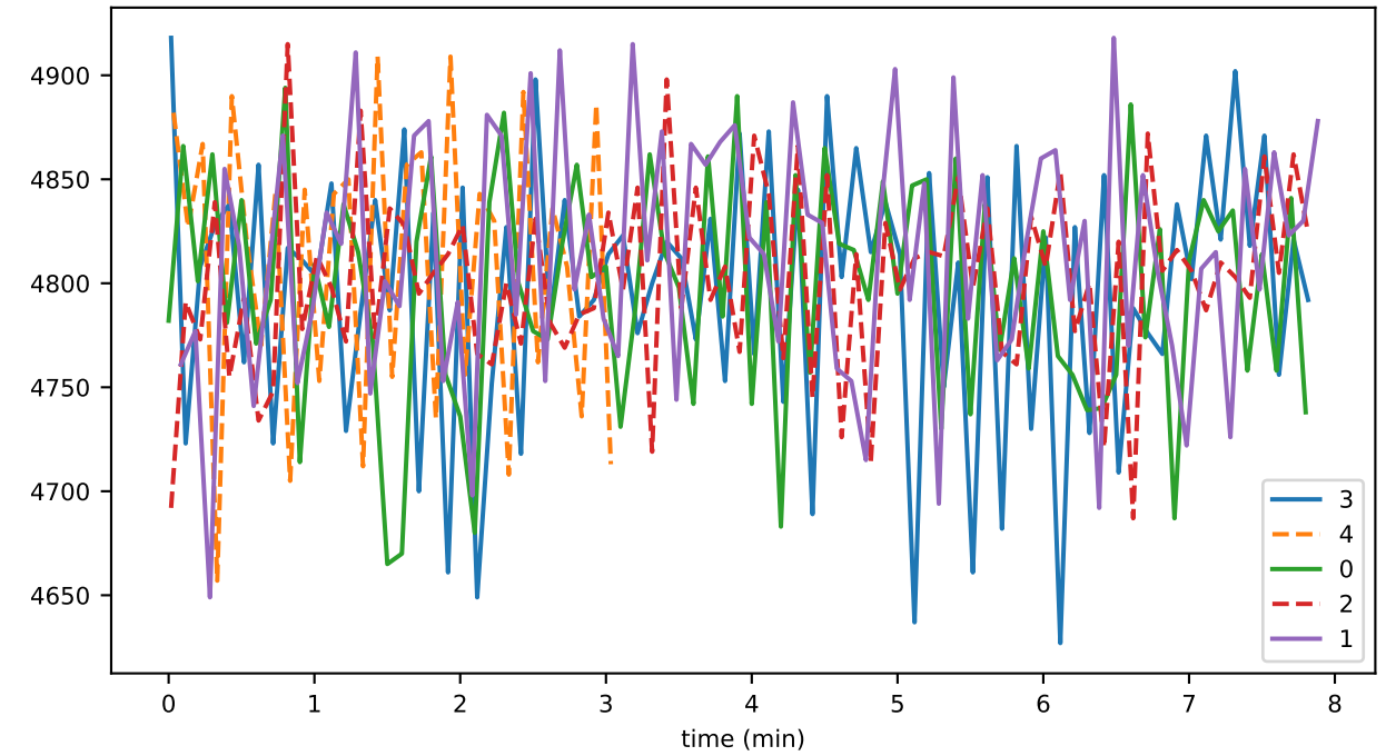
rpc_output_queue_size_00
