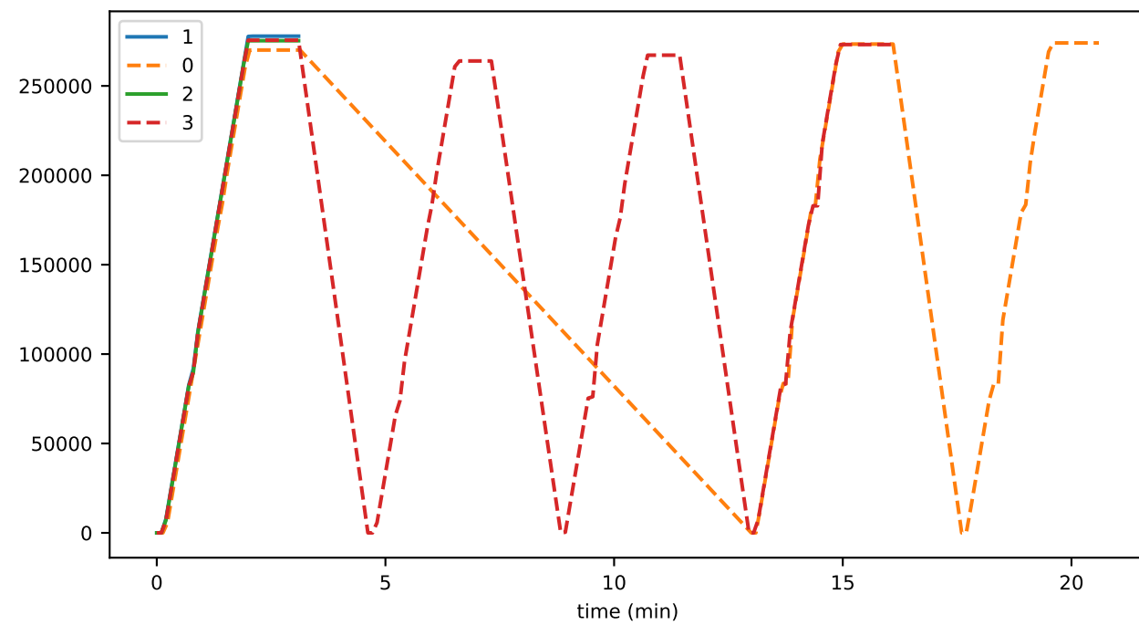
tranSub
