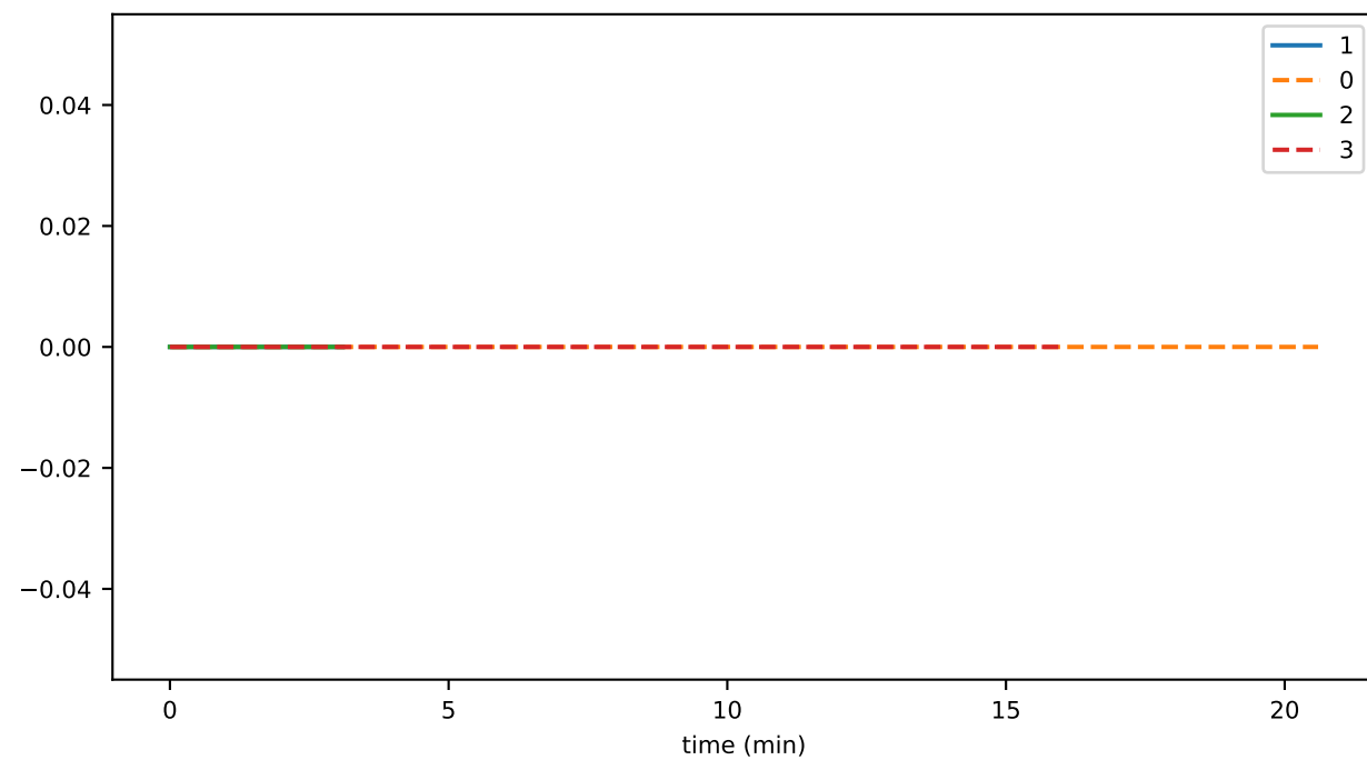
tranSub
