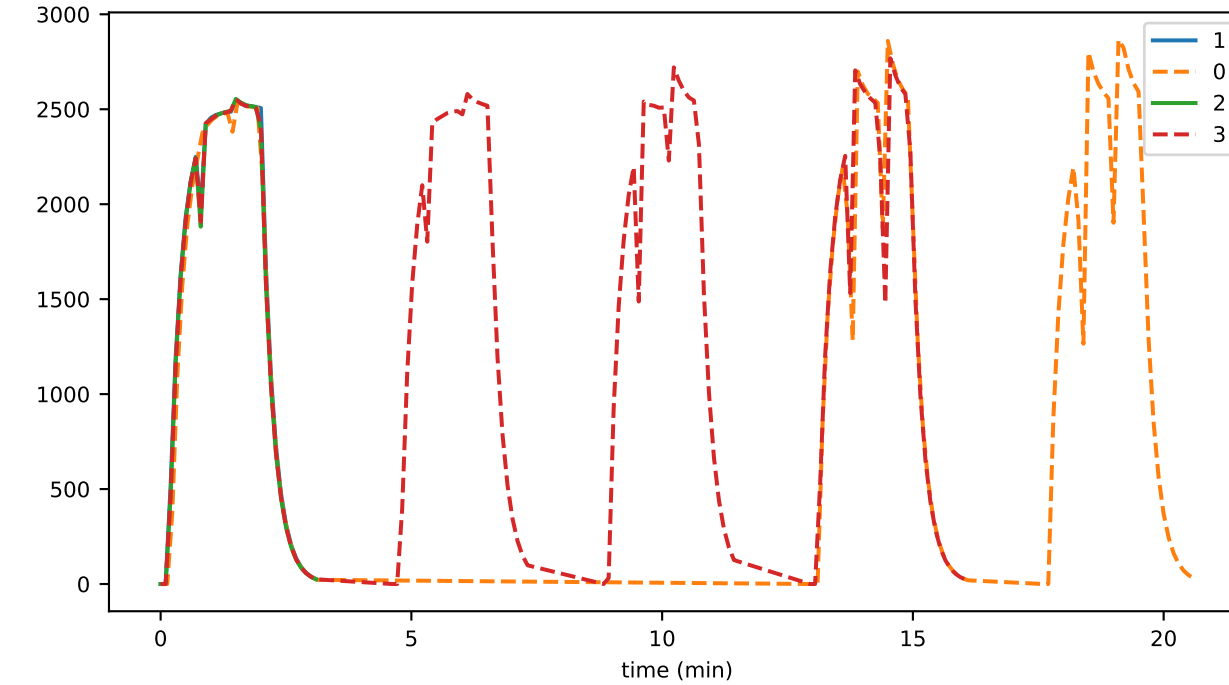
tranSubTPS
