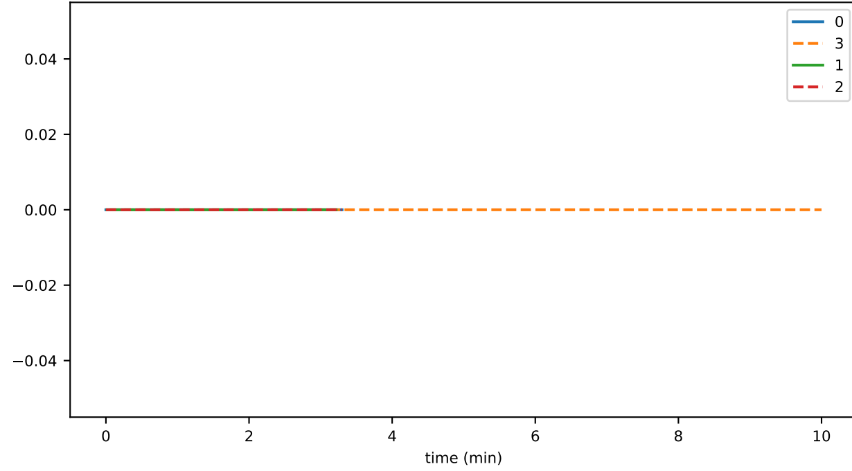
endsReconnectAsSender
