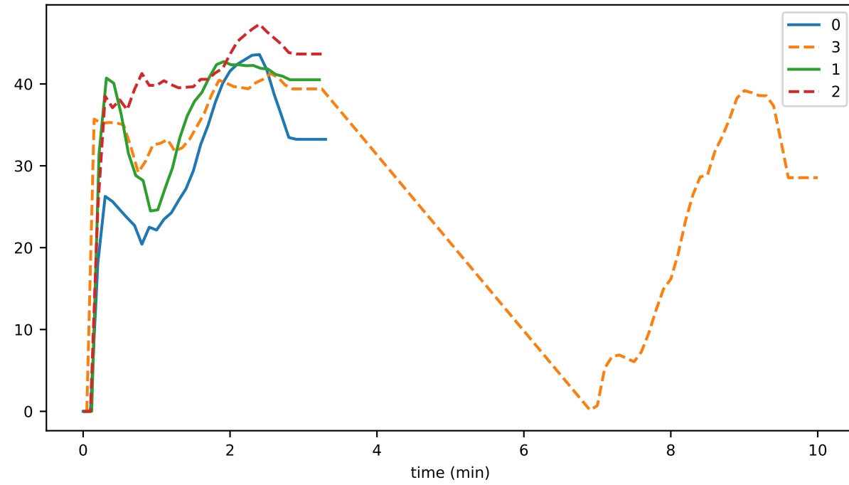
endsReconnectAsSender
