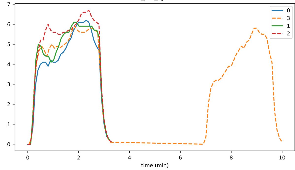
ev_per_syncR
