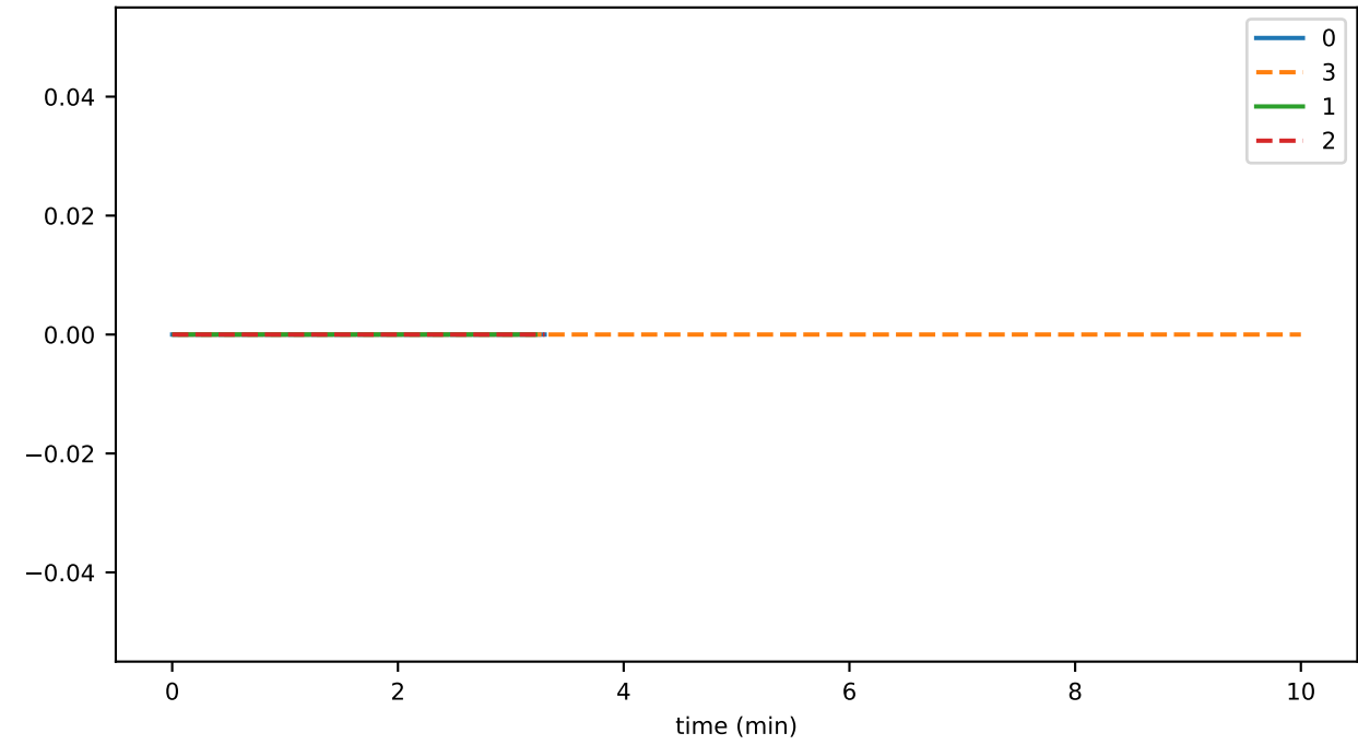
ev_per_syncR
