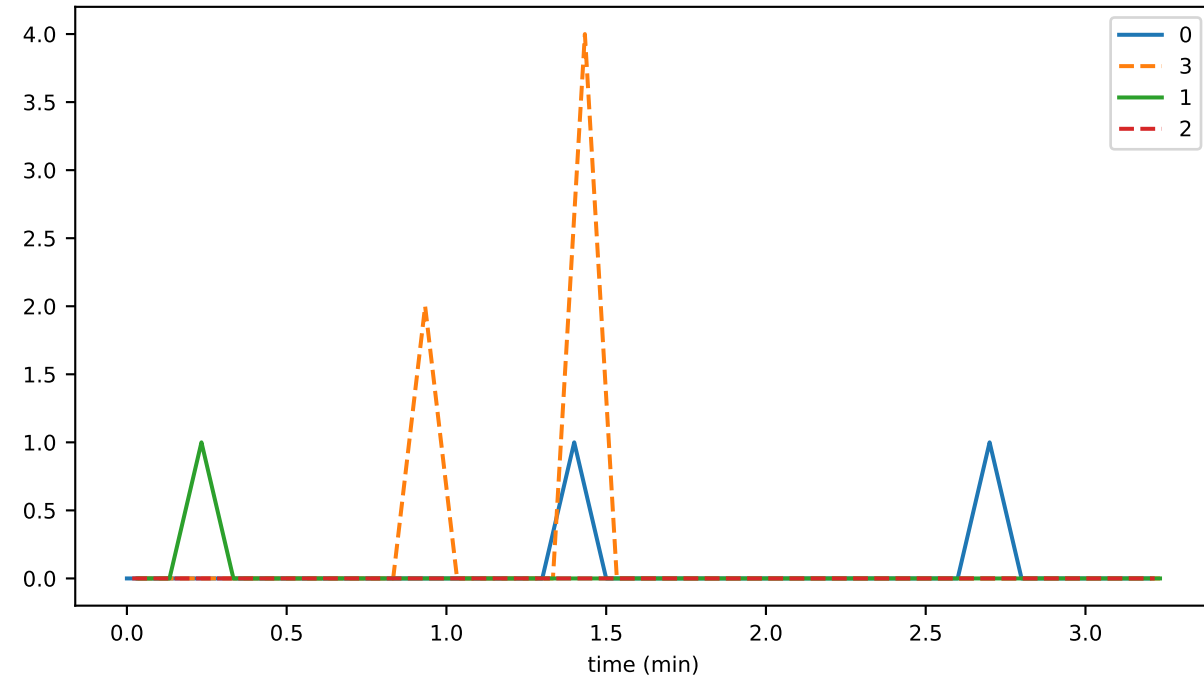
EventHasher_unhandled_task_count
