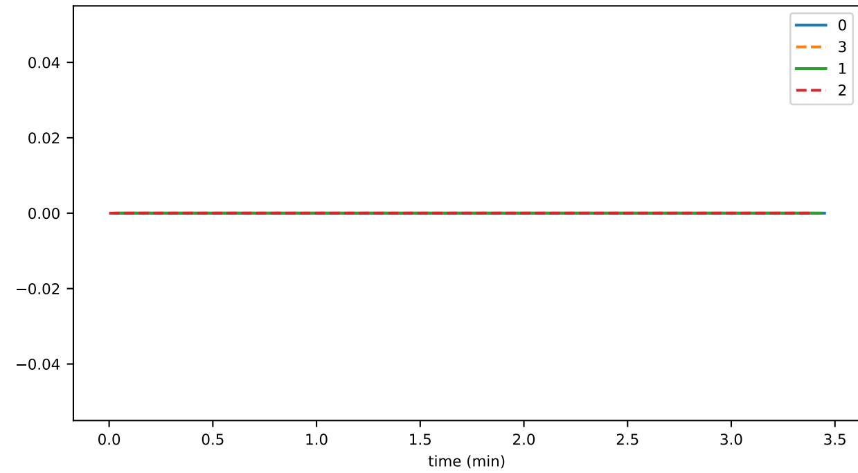
sync_round_lag
