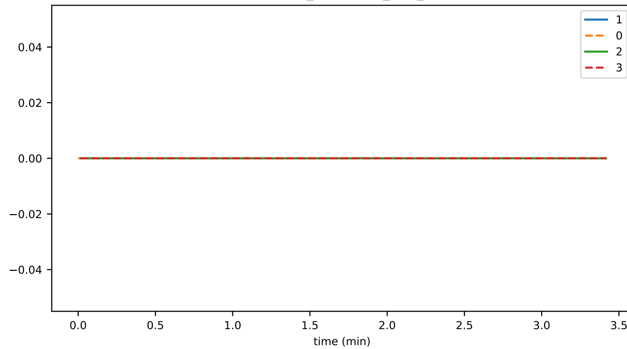
EventHasher_unhandled_task_count
