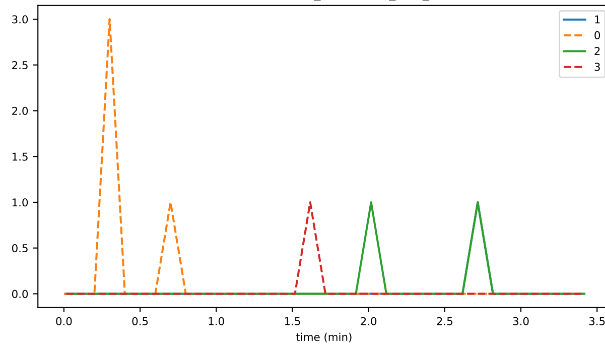
EventHasher_unhandled_task_count
