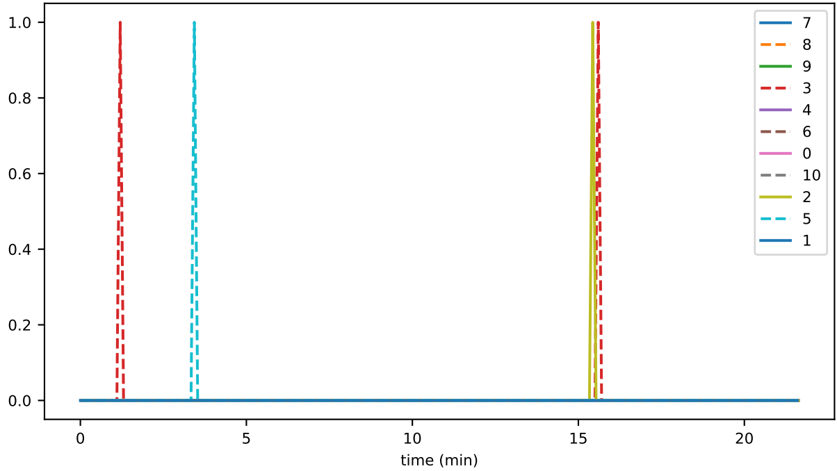
IssDetector_unhandled_task_count
