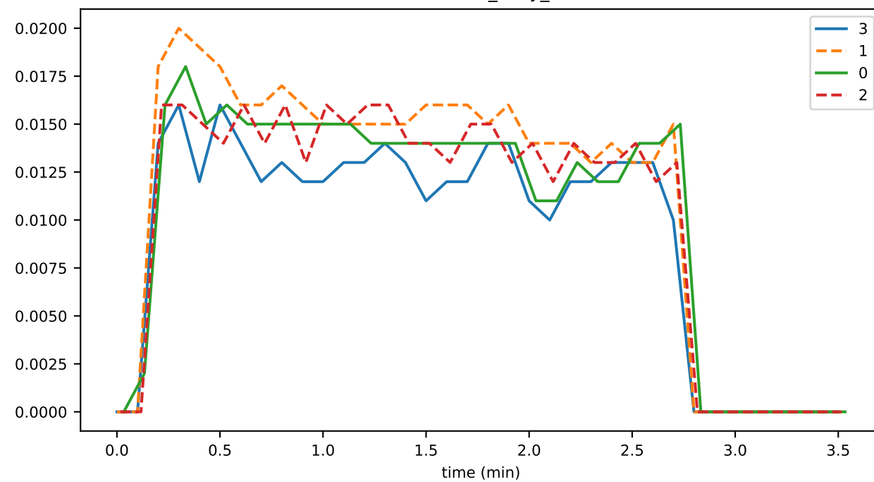
InternalEventValidator_unhandled_task_count
