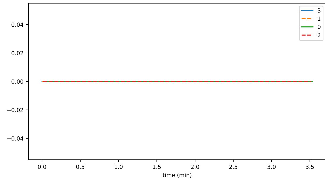
issCount
