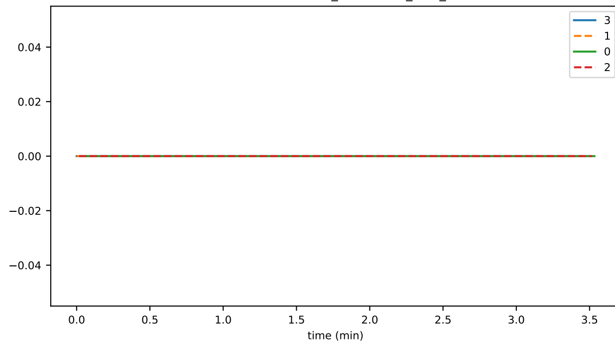
InternalEventValidator_unhandled_task_count
