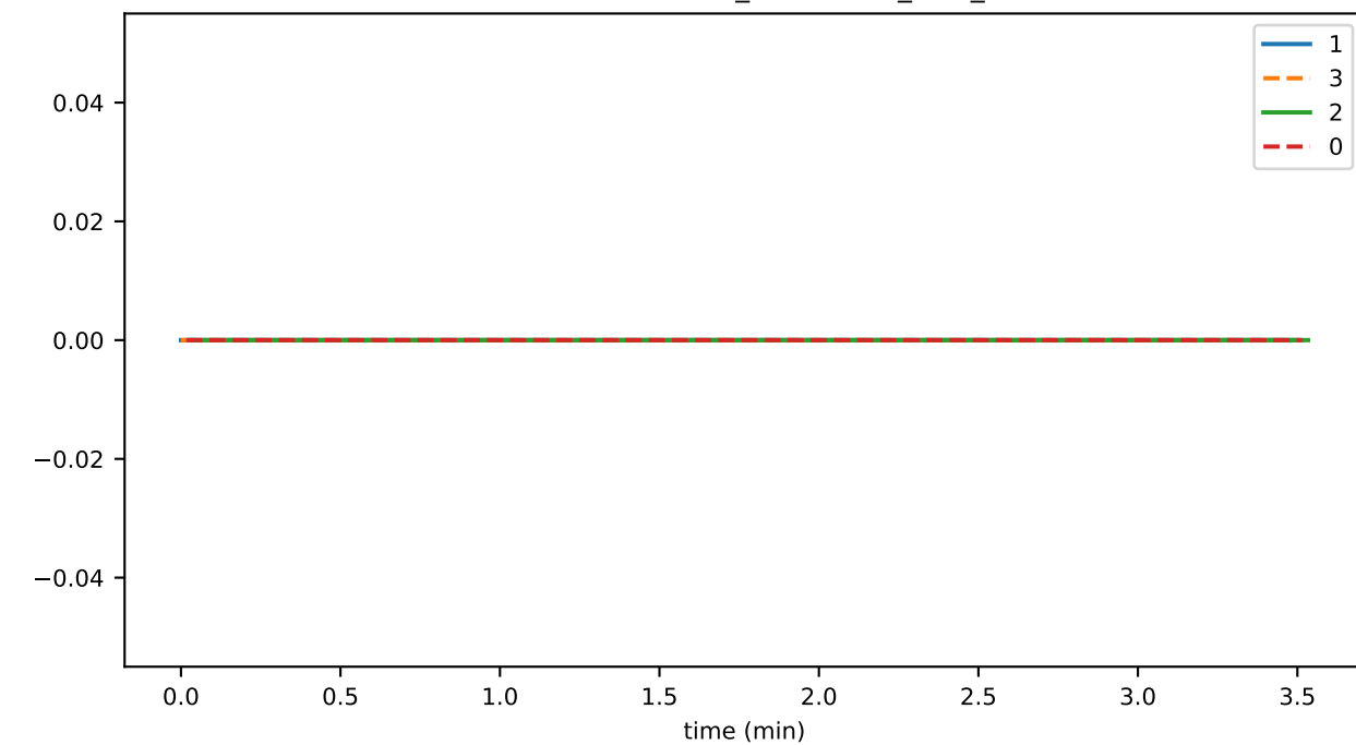
InternalEventValidator_unhandled_task_count
