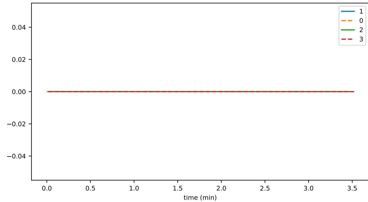
issCount
