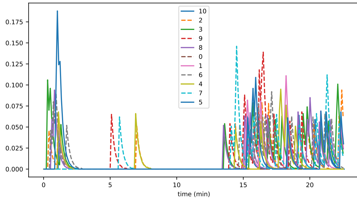
pityParent0
