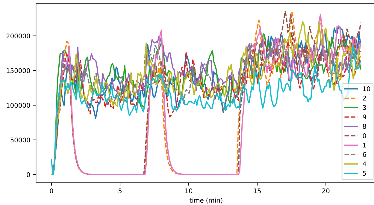
bytes_per_sec_sent_09
