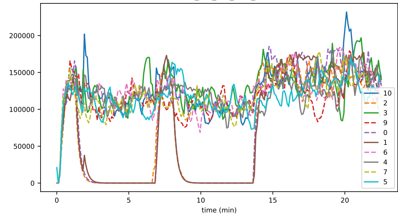
bytes_per_sec_sent_10
