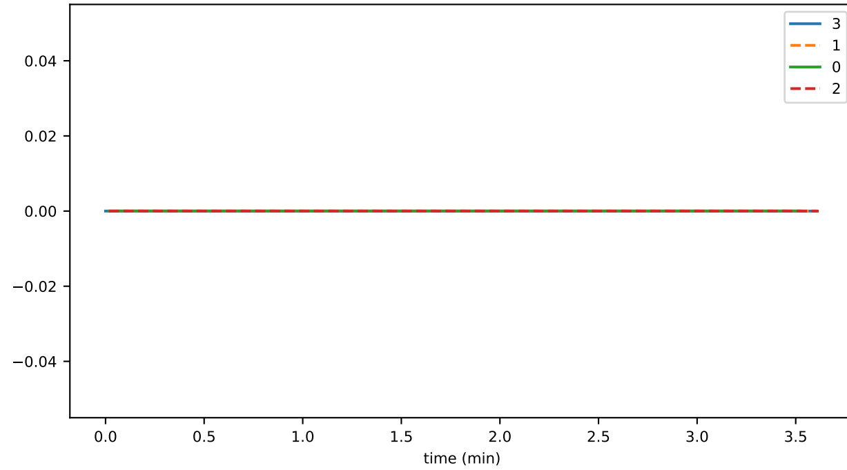
PlatSigExpandTime
