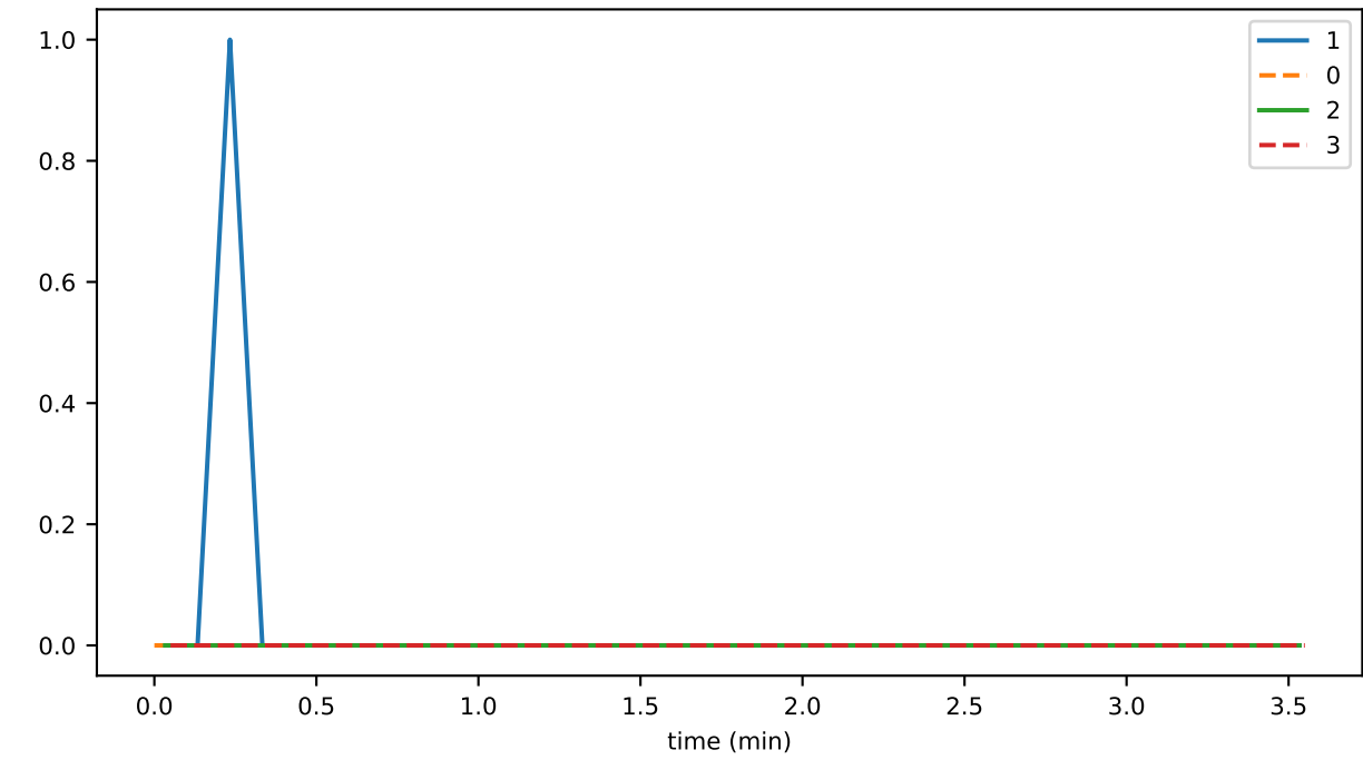
InlinePcesWriter_unhandled_task_count
