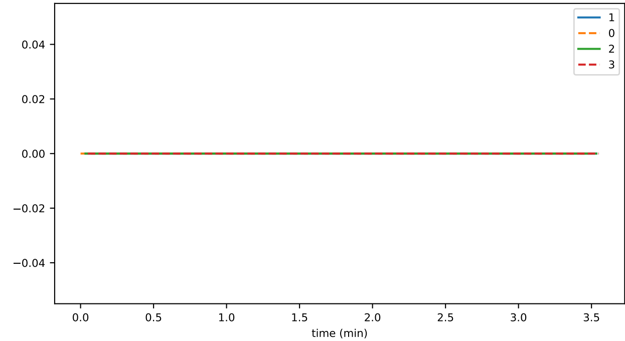
InlinePcesWriter_unhandled_task_count
