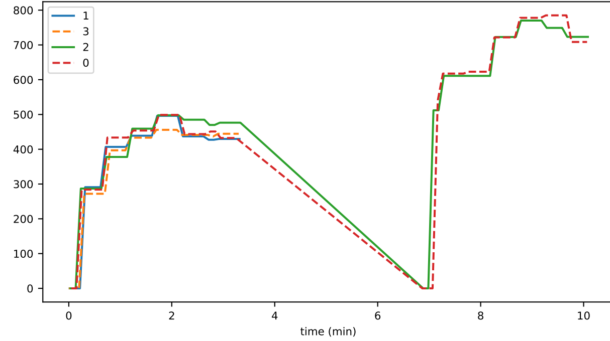
writeMerkleRootToDisk
