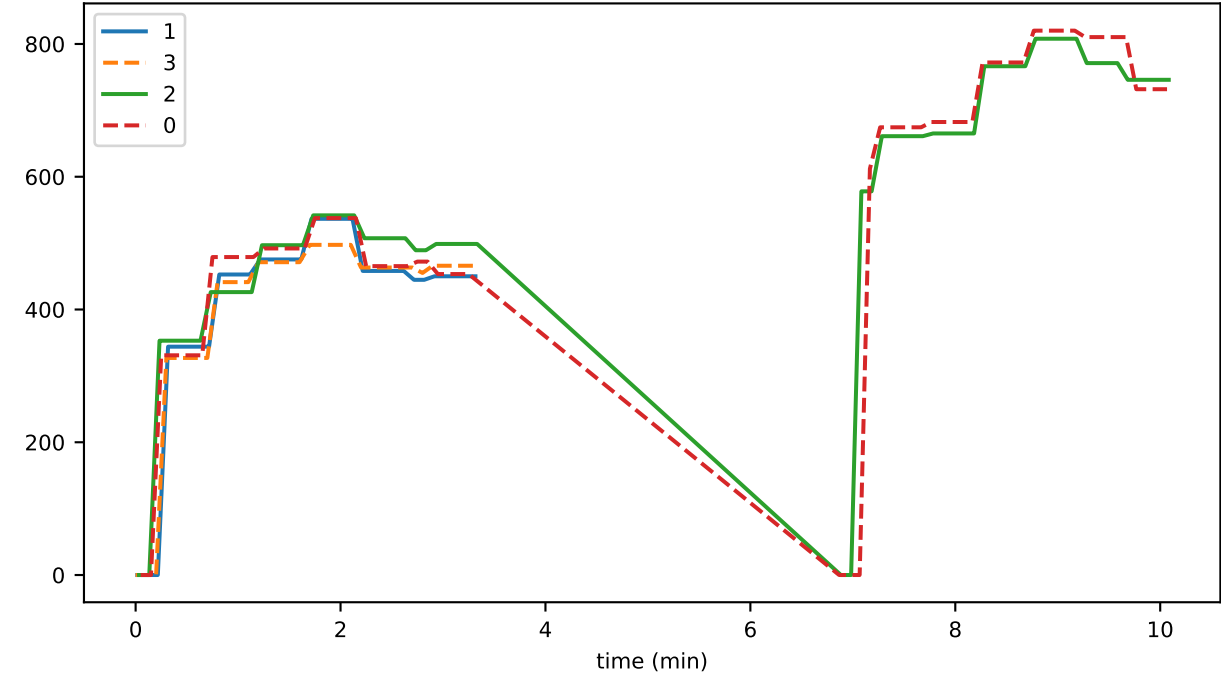
writeStateToDisk
