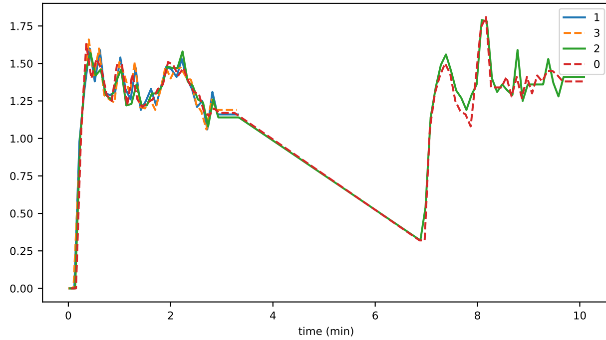
writeMerkleRootToDisk
