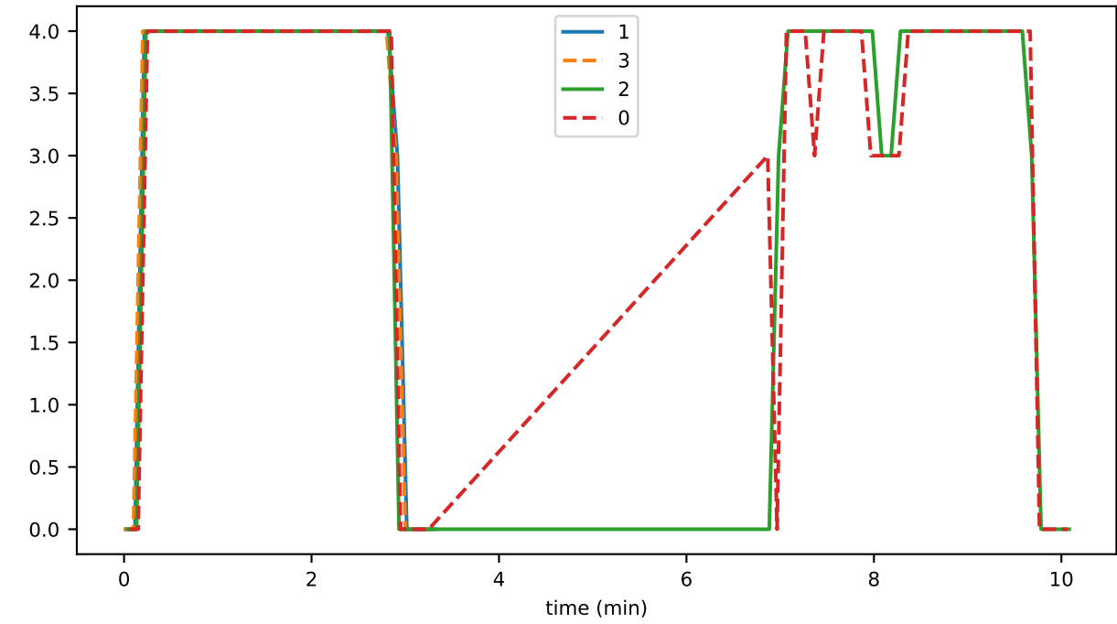
writeStateToDisk
