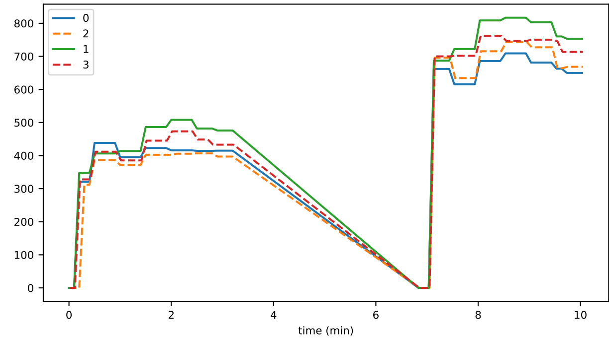
writeStateToDisk
