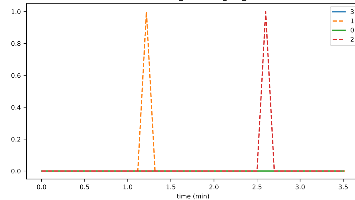
InlinePcesWriter_unhandled_task_count
