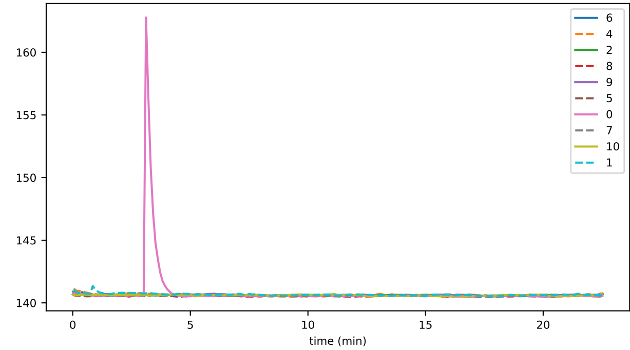
ping_ms_05
