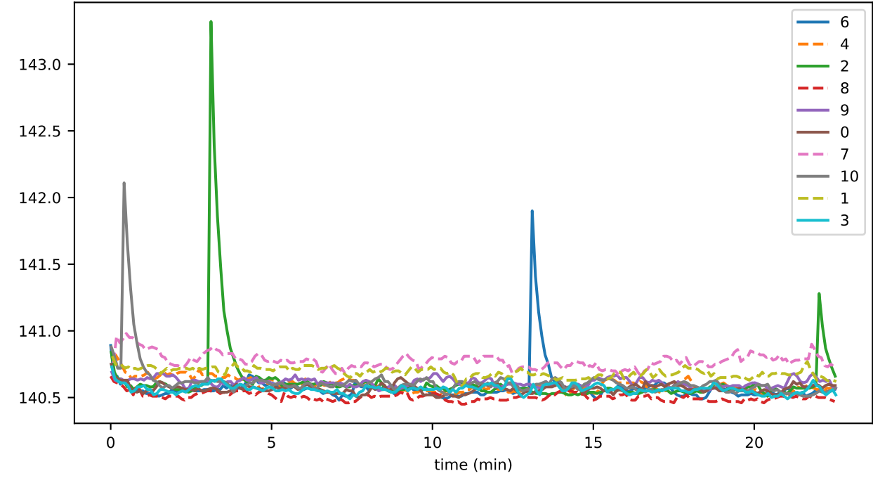
ping_ms_05
