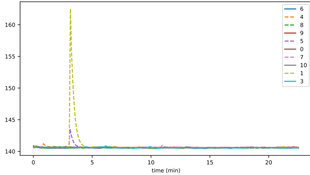
ping_ms_04
