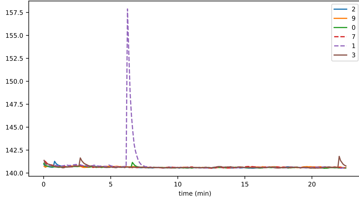
ping_ms_04
