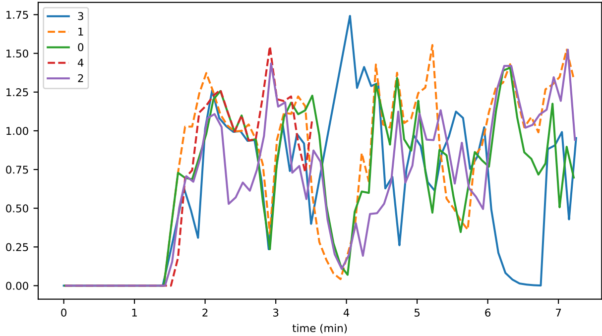
InlinePcesWriter_unhandled_task_count
