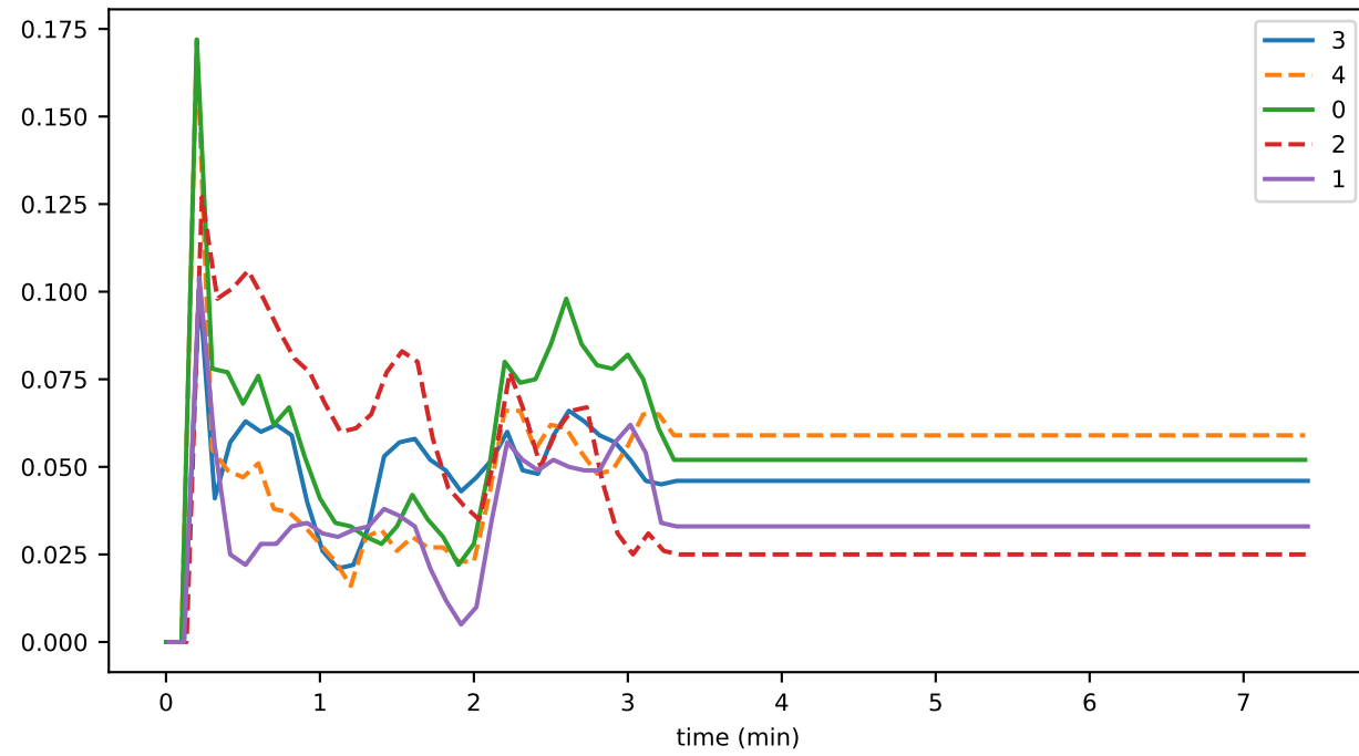
secOR2T
