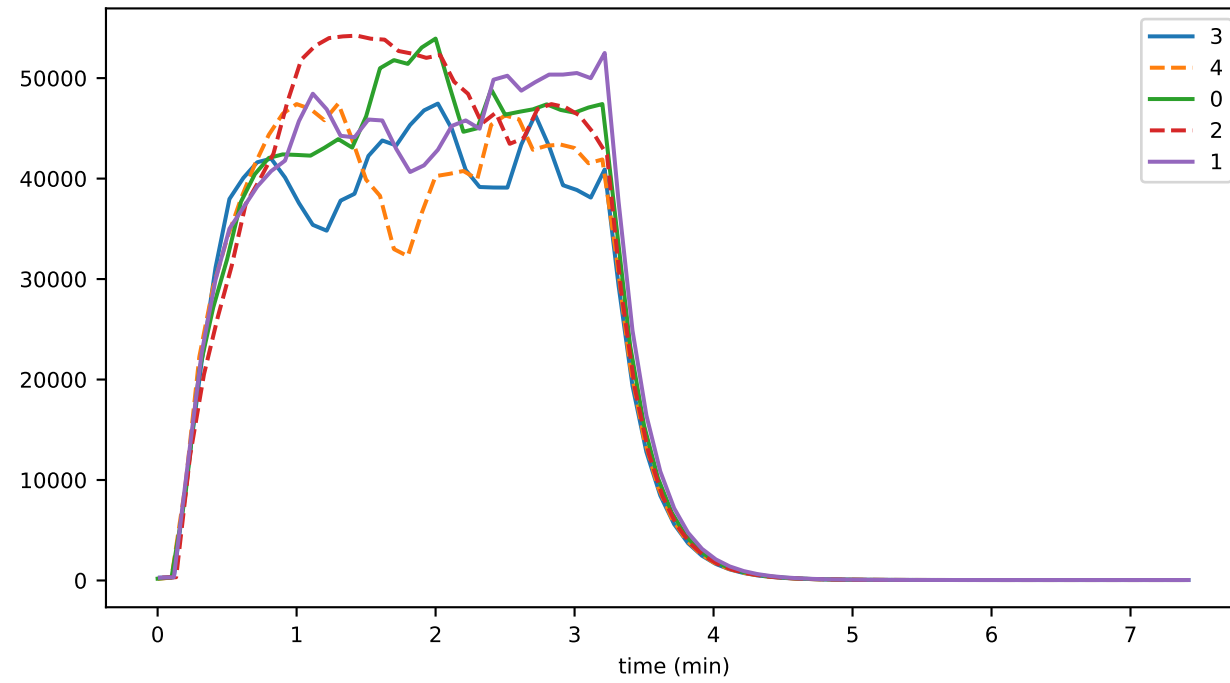
bytes_per_sec_sent
