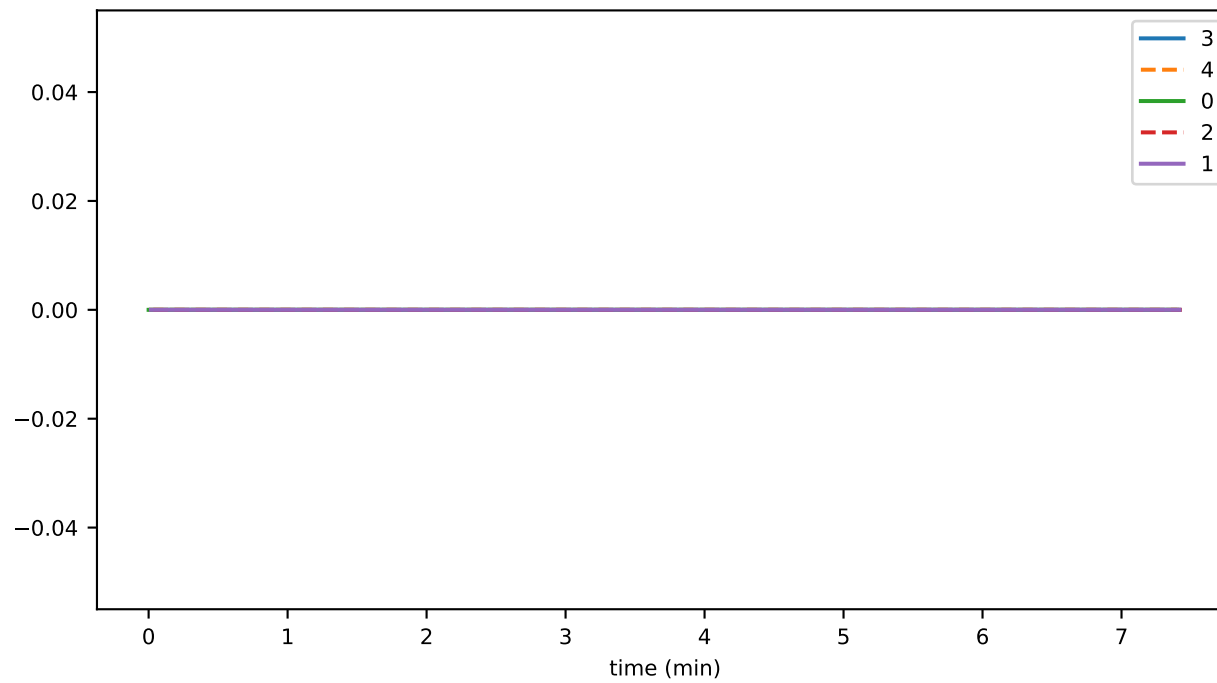
TtISig
