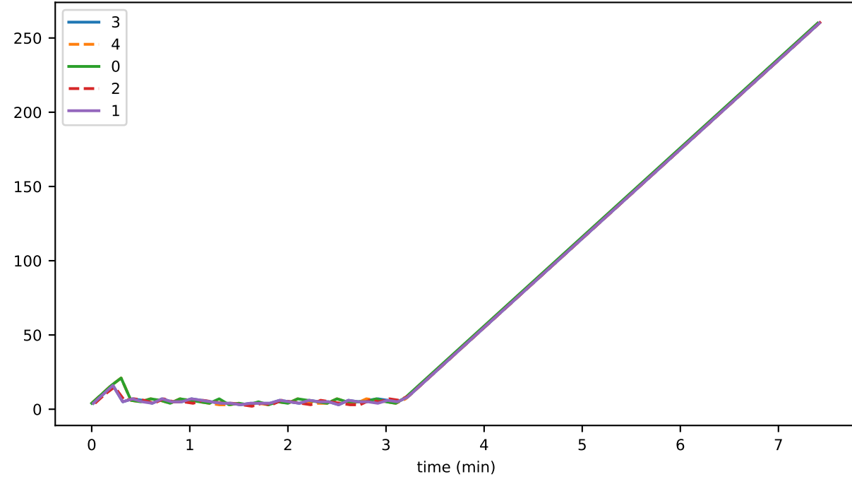
oldestISSTestingToolStateSeconds
