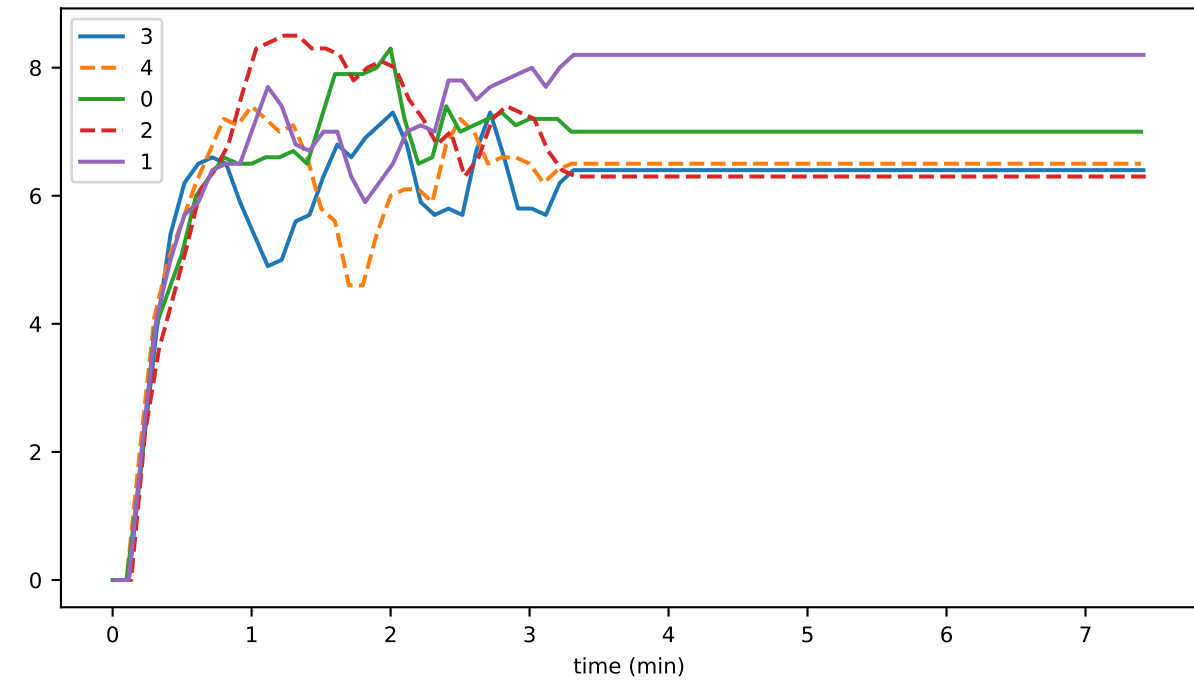
ev_per_syncS
