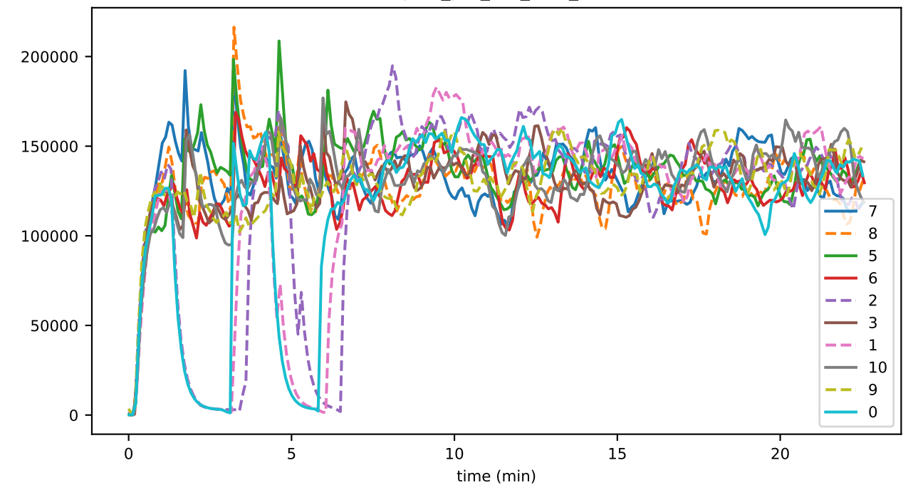
bytes_per_sec_sent_06
