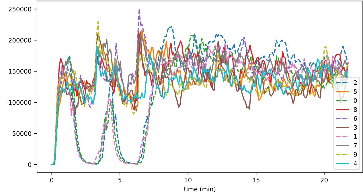
bytes_per_sec_sent_10
