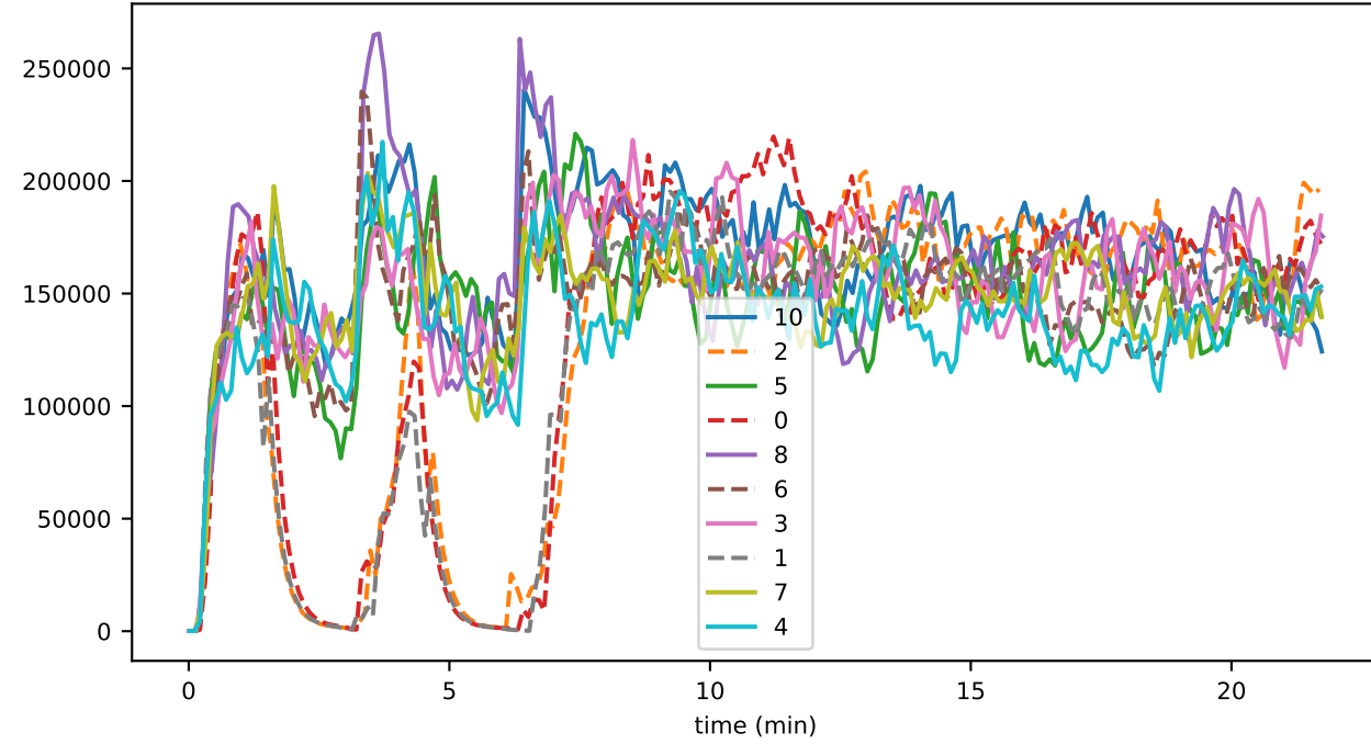
bytes_per_sec_sent_09
