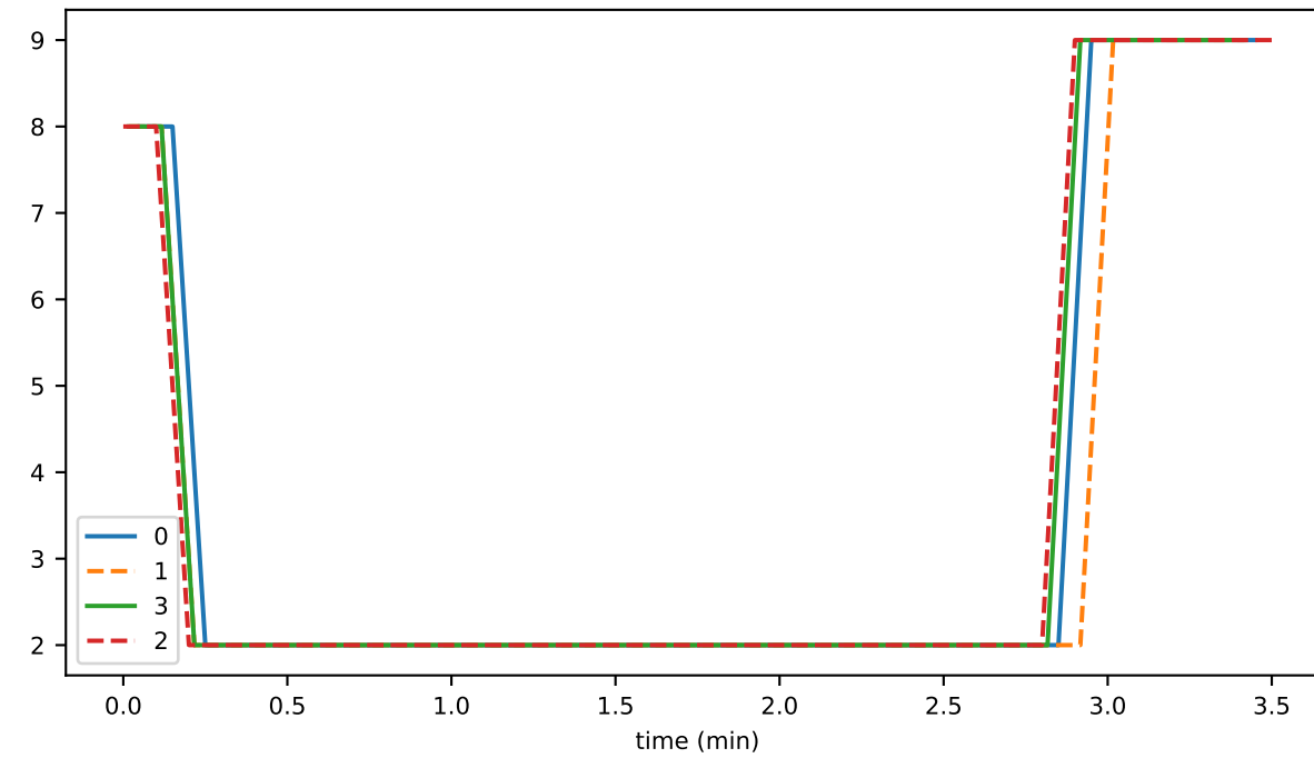
PlatSigExpandTime
