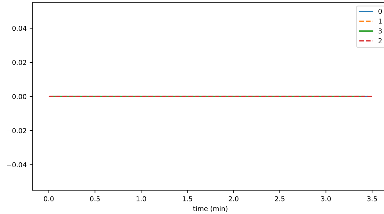
PlatSigExpandTime
