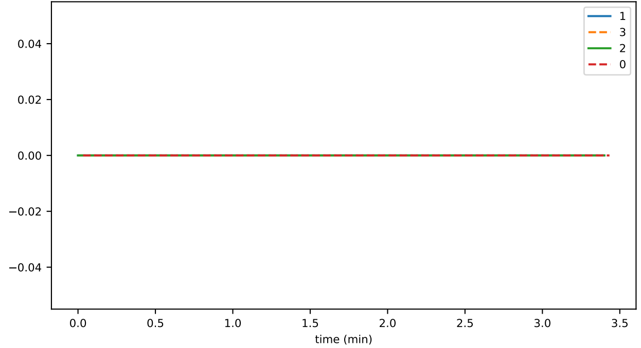
InternalEventValidator_unhandled_task_count
