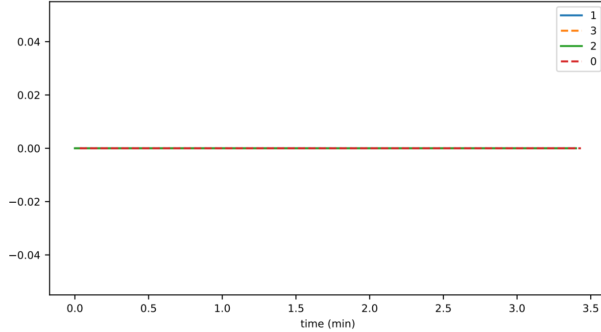
InlinePcesWriter_unhandled_task_count
