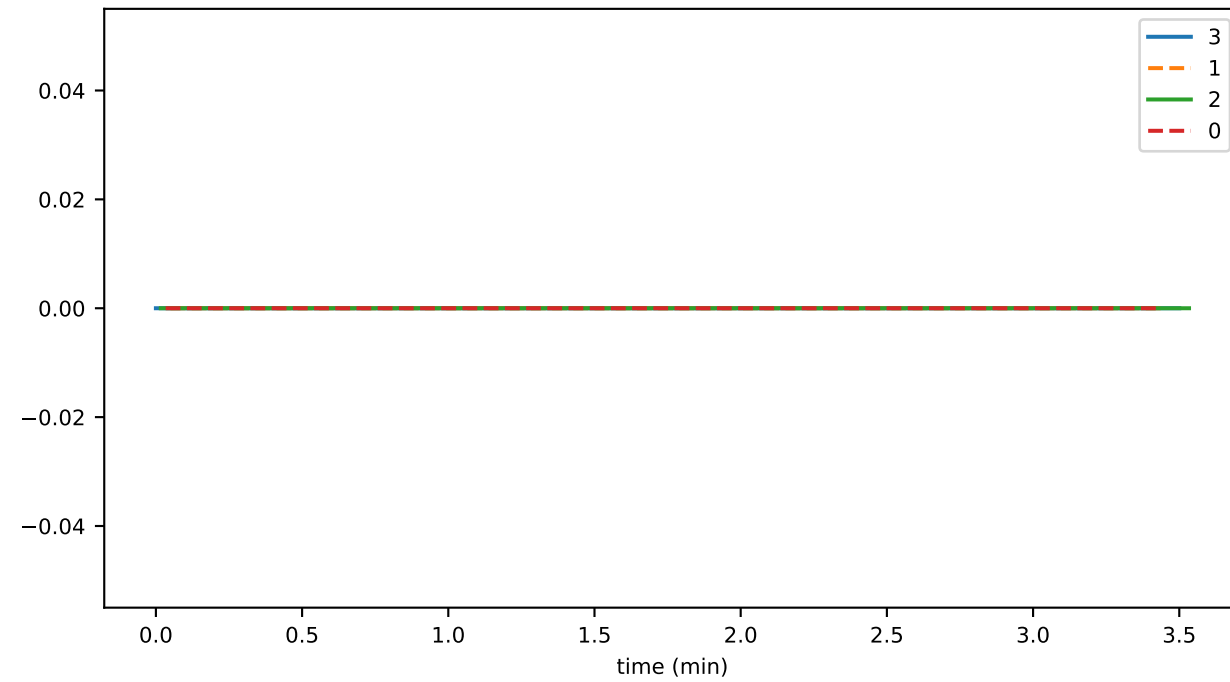
eventsInMem
