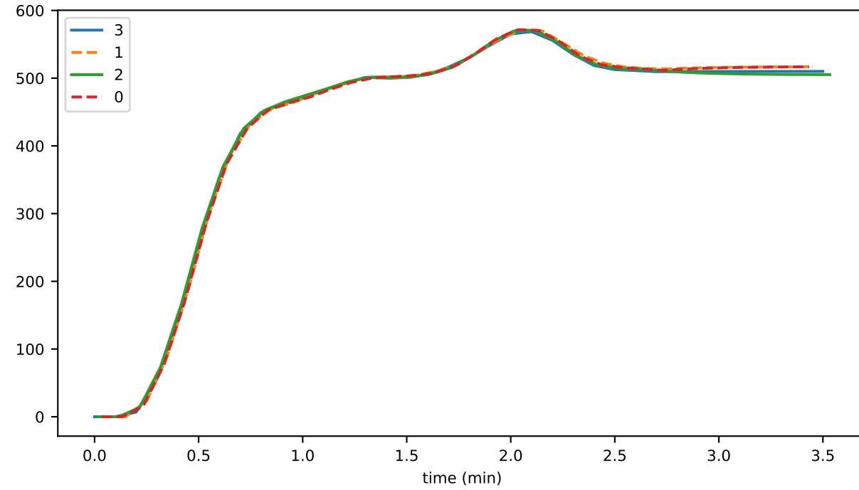
eventsInMem
