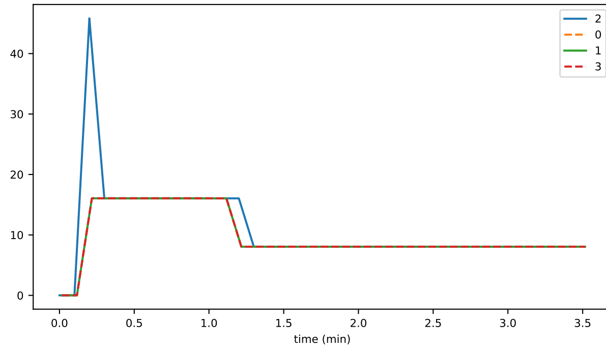
DiskspaceFree
