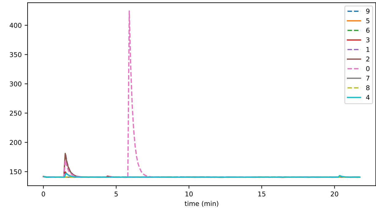
pityParent1
