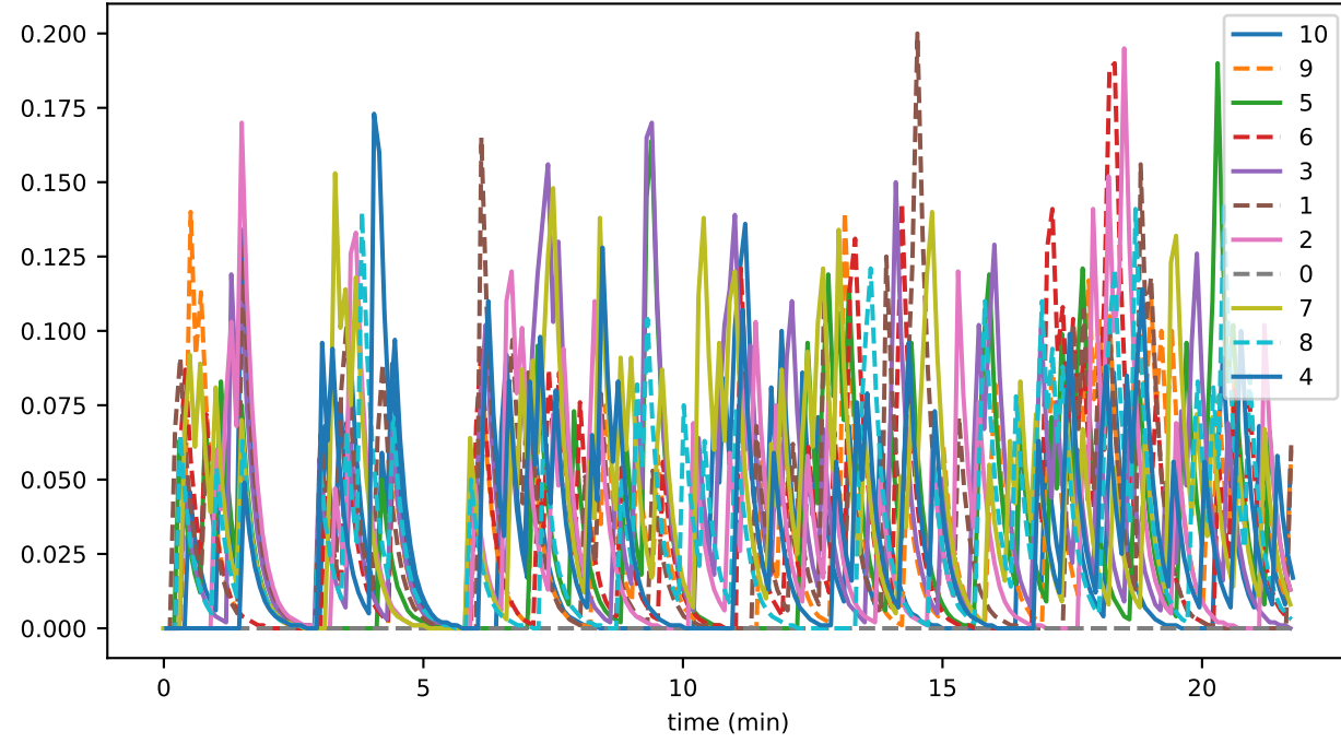
pityParent0
