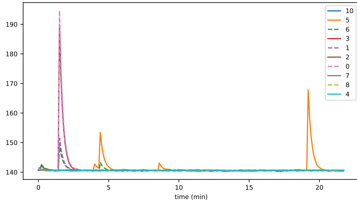
pityParent0
