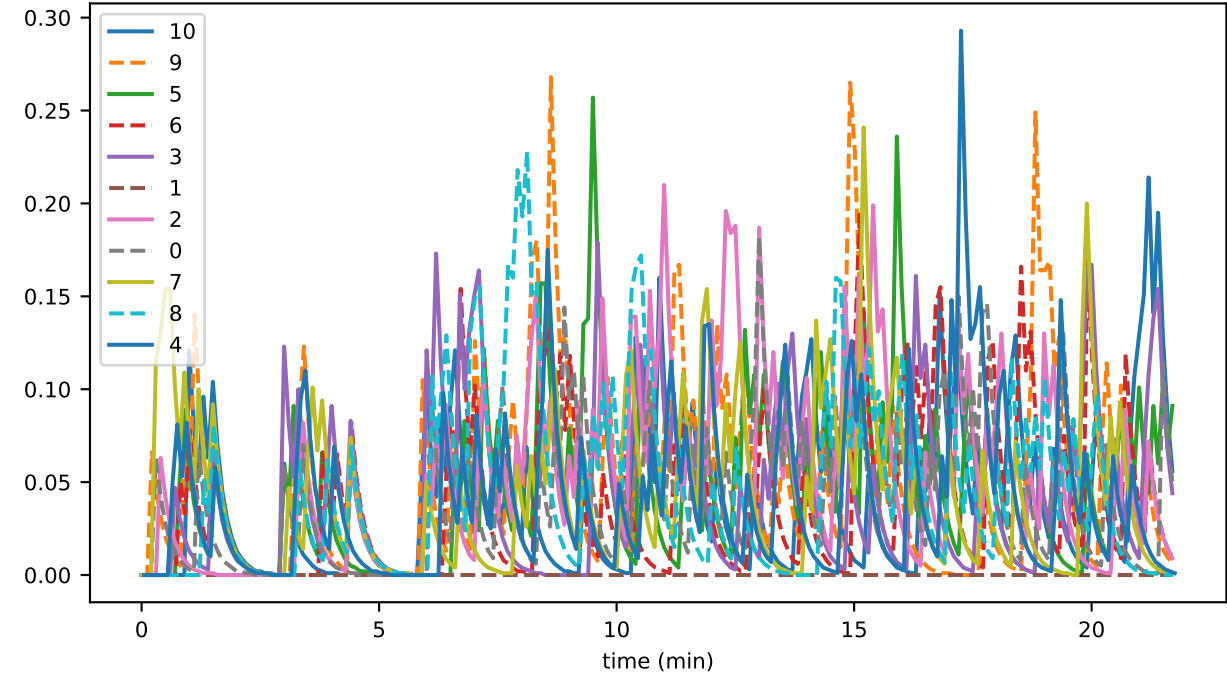
pityParent1
